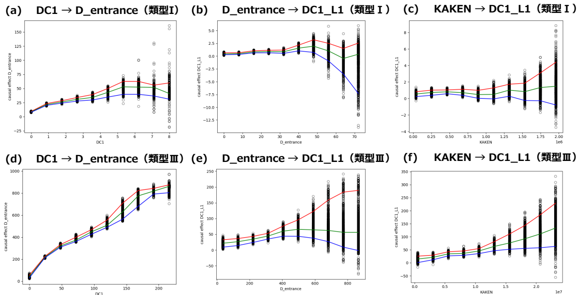
図 2: RESIT を bootstrap 法と組み合わせて因果探索・予測を繰り返し、代表的なパスについて非線形因果効果を可視化したもの。
