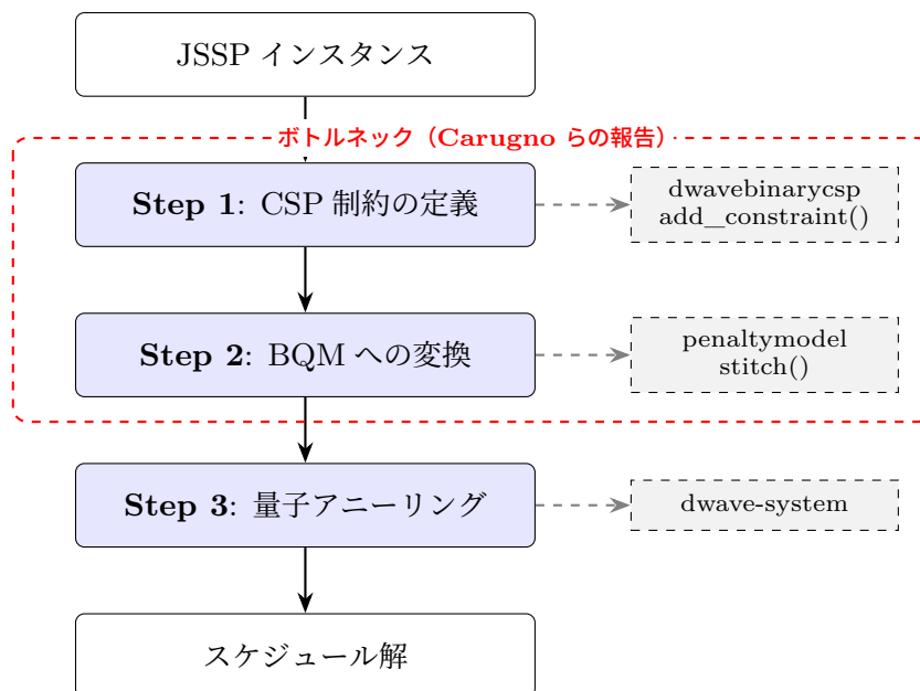
図 4.1 Carugno らの手法の全体フロー。JSSP インスタンスを CSP 形式で記述し、BQM に変換後、量子アニーリングで求解する。赤枠部分が Carugno らによりボトルネックと報告されている。
