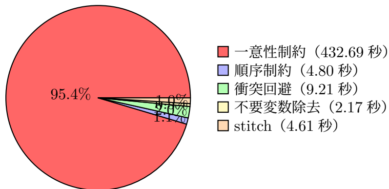
図 4.6 n = 20 における処理時間の内訳．一意性制約が 95.4% を占める．
