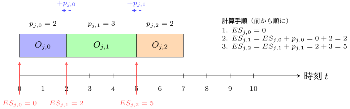
図 3.7 最早開始時刻（ES）の計算．各操作の最早開始時刻は，先行操作の処理時間を前から順に累積して求める． ES_{j,k} = \sum_{k' < k} p_{j,k'}
