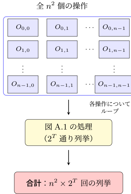
図 A.2 一意性制約登録の全体ループ. 全 n^2 個の操作それぞれに対して図 A.1 の処理が実行され, 合計 n^2 \times 2^T 回の列挙が発生する.
