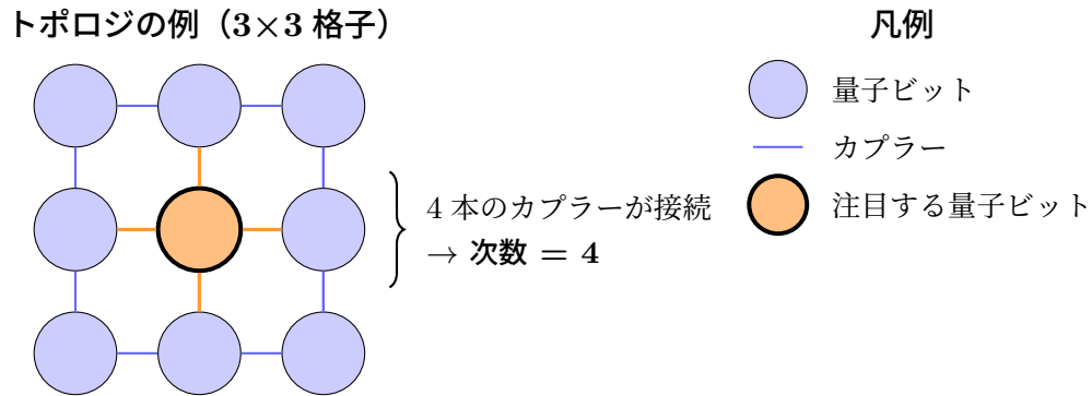
図 2.1 トポロジ・次数・カプラーの概念図
