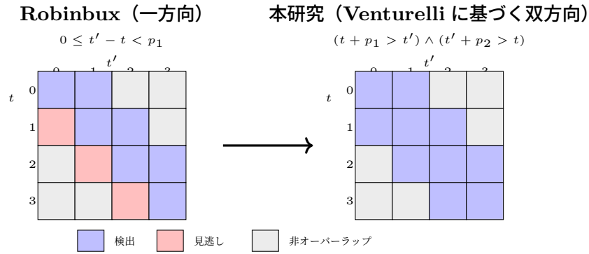
図 5.13 h_2 制約判定の比較 ( p_1 = p_2 = 2 の例)．左：Robinbux（一方向判定，赤は見逃し），右：本研究（双方向判定）．
