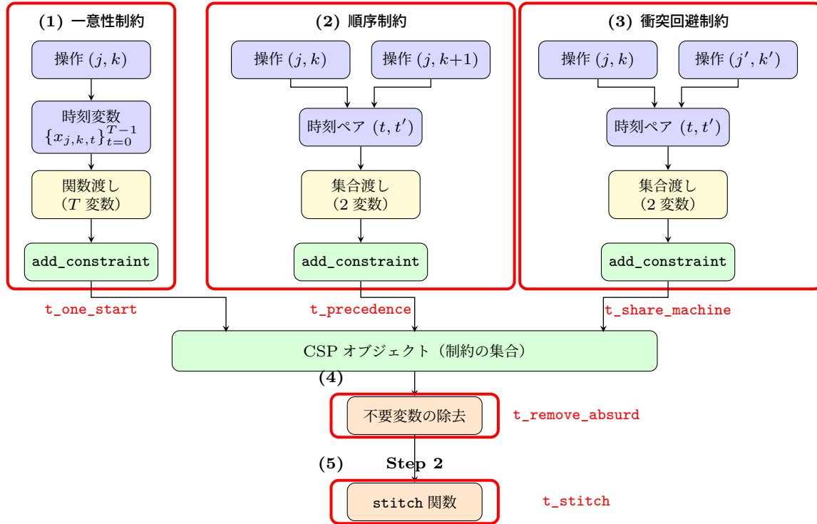
図 4.3 処理時間の測定箇所 (図 4.2 を再掲). 赤枠で囲んだ 5 箇所の処理時間を測定する.
