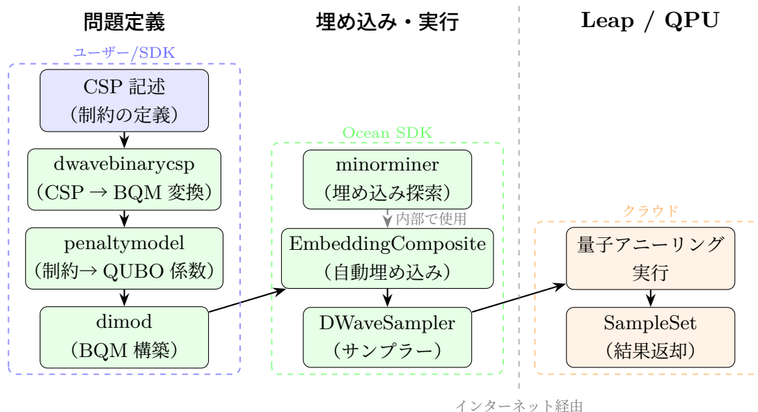
図 2.3 Ocean SDK の主要コンポーネントと実行フロー
