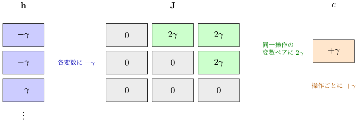
図 5.4 h_3 制約の係数加算. 一意性制約の展開により, h の各要素に -\gamma , J の上三角部分に 2\gamma , c に +\gamma が加算される ( \gamma はペナルティ係数).
