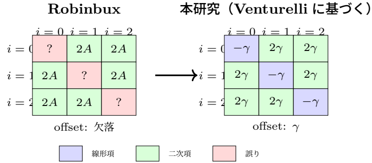
図 5.12 h_3 制約係数の比較 (1 操作・3 変数の例). 左: Robinbux (線形項誤り・offset 欠落), 右: 本研究 (Venturelli の定式化に基づく正確な係数).
