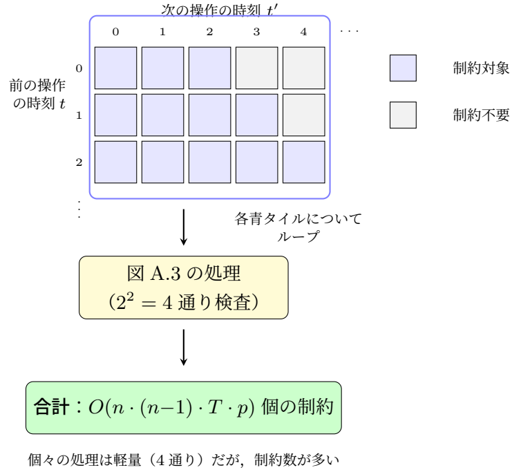
図 A.4 順序制約登録の全体ループ. 1 つの操作ペア (O_{j,k}, O_{j,k+1}) に対して, 青タイルの数だけ add_constraint が実行される.
