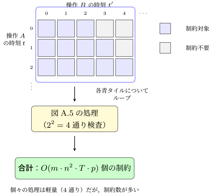
図 A.6 衝突回避制約登録の全体ループ. 同一機械上の操作ペア (O_A, O_B) に対して, 青タイルの数だけ add_constraint が実行される.
