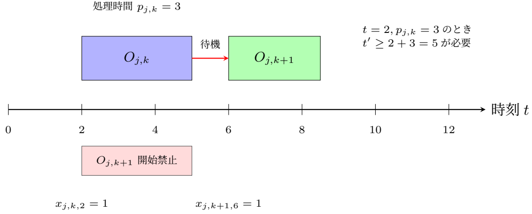
図 3.3 順序制約の概念. 操作 O_{j,k} が時刻 t に開始し処理時間 p_{j,k} の場合, 次の操作 O_{j,k+1} は時刻 t + p_{j,k} 以降にしか開始できない.
