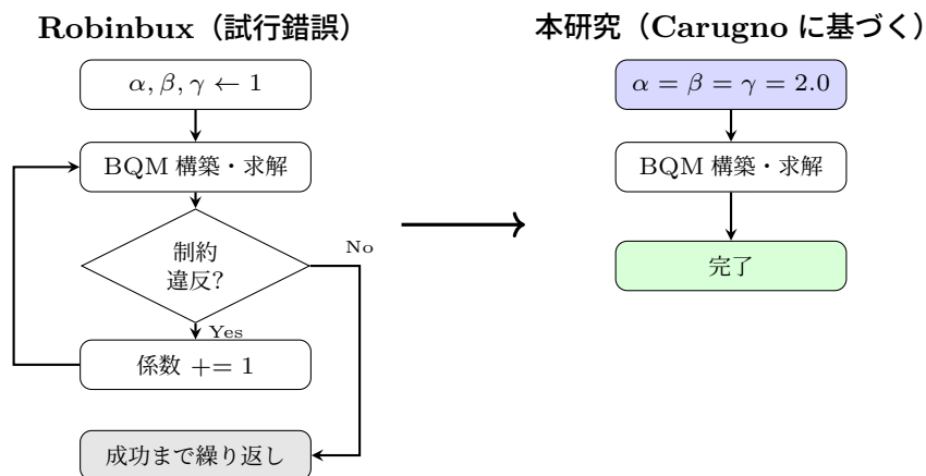
図 5.10 ペナルティ係数設定の比較．左：Robinbux（試行錯誤ループ），右：本研究（Carugno らの設定値を直接使用）．
