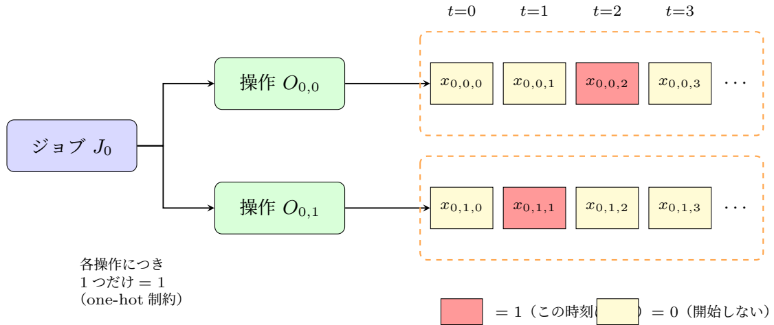
図 3.1 ジョブ，操作，時間インデックス変数の関係．各ジョブは複数の操作を持ち，各操作に対して時刻ごとの二値変数が存在する．各操作について，正確に 1 つの変数のみが 1 となる（one-hot 制約）．
