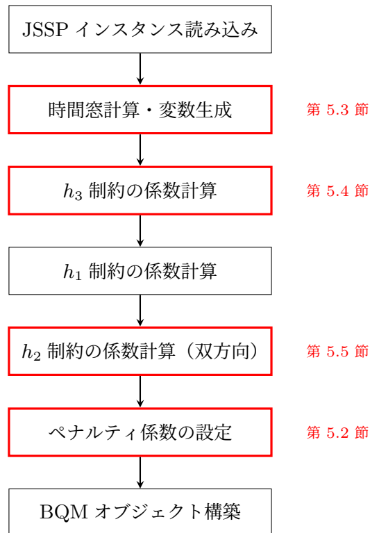
図 5.9 BQM 直接構築の処理フロー（赤枠：本研究の貢献部分）
