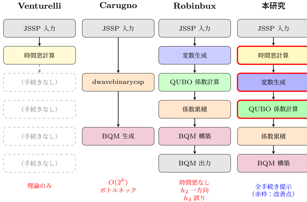
図 5.14 各手法の BQM 構築フロー比較. 左から Venturelli, Carugno, Robinbux, 本研究. 赤枠は本研究での改善点.
