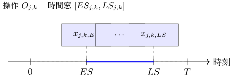
図 5.3 時間窓に基づく変数生成（時間窓内のみに変数を生成）
