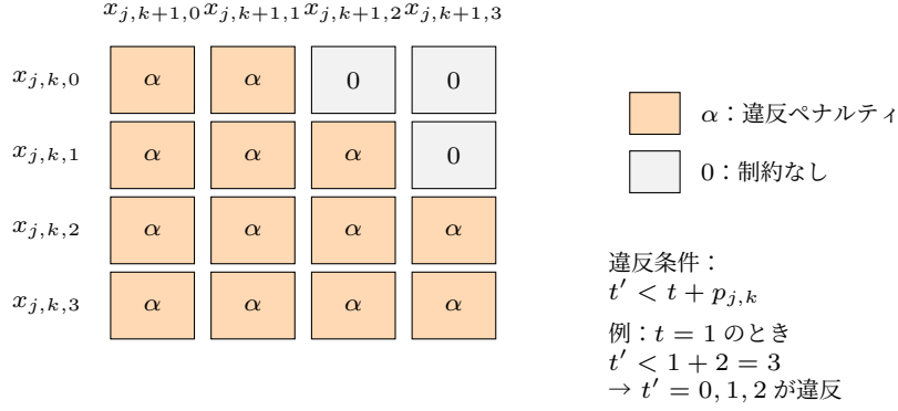
図 3.4 順序制約における QUBO 部分行列の構造 ( p_{j,k} = 2 の場合). 行は操作 O_{j,k} の時刻変数, 列は操作 O_{j,k+1} の時刻変数を表す. 違反条件 t' < t + p_{j,k} を満たす (t, t') ペアに対して係数 \alpha が設定される.
