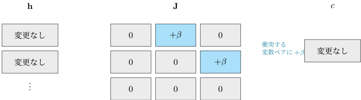
図 5.6 h_2 制約の係数加算．同一機械で時間的に重複する変数ペア (i, j) に対して J_{ij} に +\beta が加算される ( \beta はペナルティ係数)． \mathbf{h} と \mathbf{c} は変更なし．
