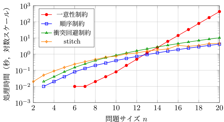
図 4.4 問題サイズと処理時間の関係 (対数スケール). 一意性制約のみが指数的增长を示し, 他の処理は緩やかな増加にとどまる.
