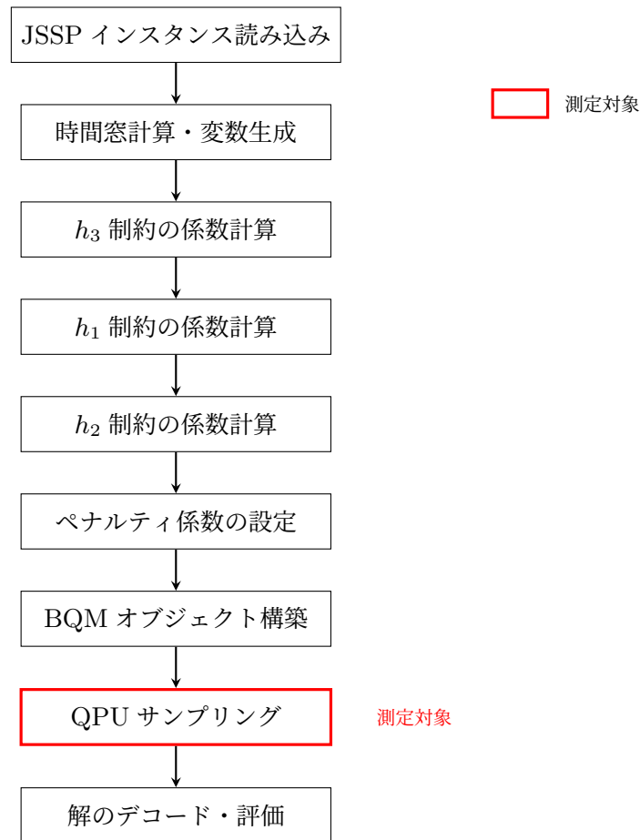
図 6.5 実験 2 の測定対象（赤枠：QPU 実行時間の測定箇所）
