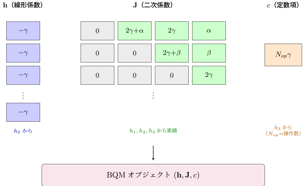
図 5.8 累積された係数の最終的な構造. \mathbf{h} は h_3 制約から, \mathbf{J} は h_1, h_2, h_3 制約から, c は h_3 制約から累積される.
