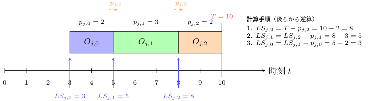
図 3.8 最遅開始時刻（LS）の計算．各操作の最遅開始時刻は，timespan から後続操作の処理時間を後ろから逆算して求める． LS_{j,k} = T - \sum_{k' \geq k} p_{j,k'}
