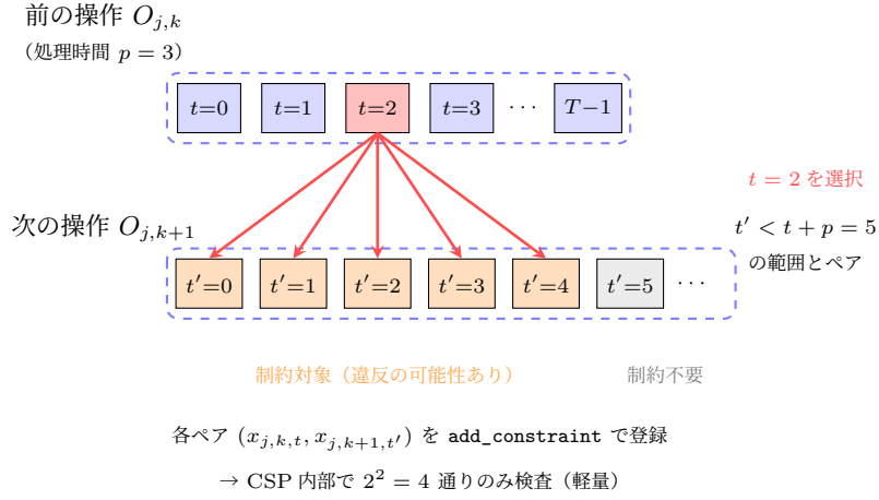
図 A.3 順序制約のペア生成. 前の操作 O_{j,k} の時刻 t (例: t = 2 ) に対して, 次の操作 O_{j,k+1} の t' < t + p の範囲とペアを作り制約を登録する.
