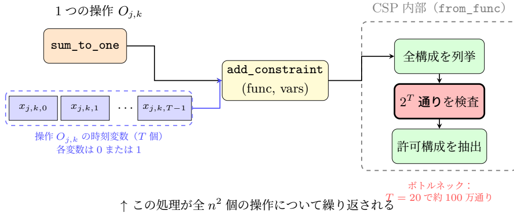
図 A.1 一意性制約の登録 (1つの操作あたり). 操作 O_{j,k} に対する T 個の時刻変数と判定関数が CSP に渡され, 内部で 2^T 通りの全構成が列挙・検査される.
