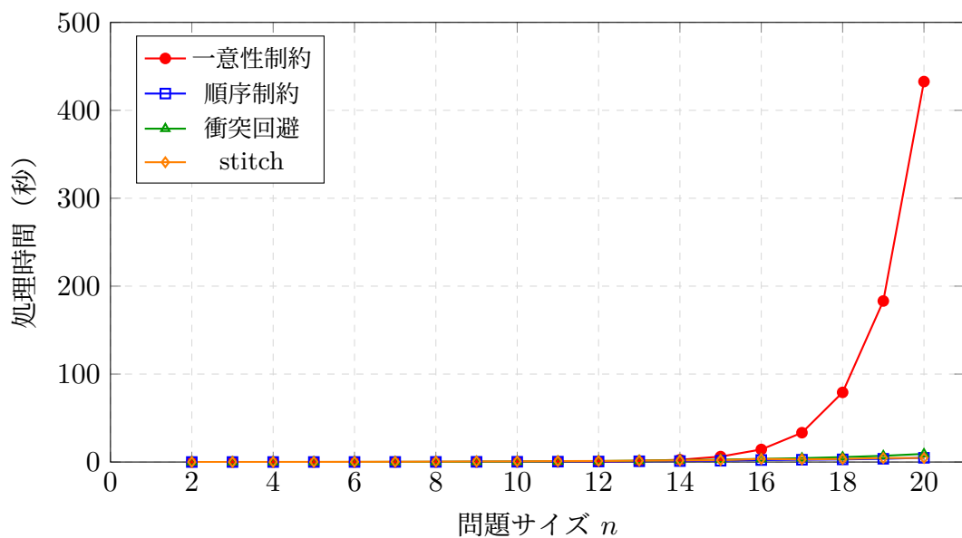
図 4.5 問題サイズと処理時間の関係 (線形スケール). 一意性制約の処理時間が指数的に増加し, 他の処理を圧倒している.
