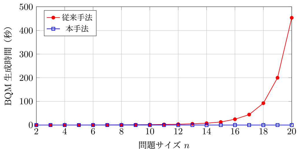
図 6.3 問題サイズと BQM 生成時間の関係 (秒スケール). 従来手法は n \geq 16 で急激に増加する.
