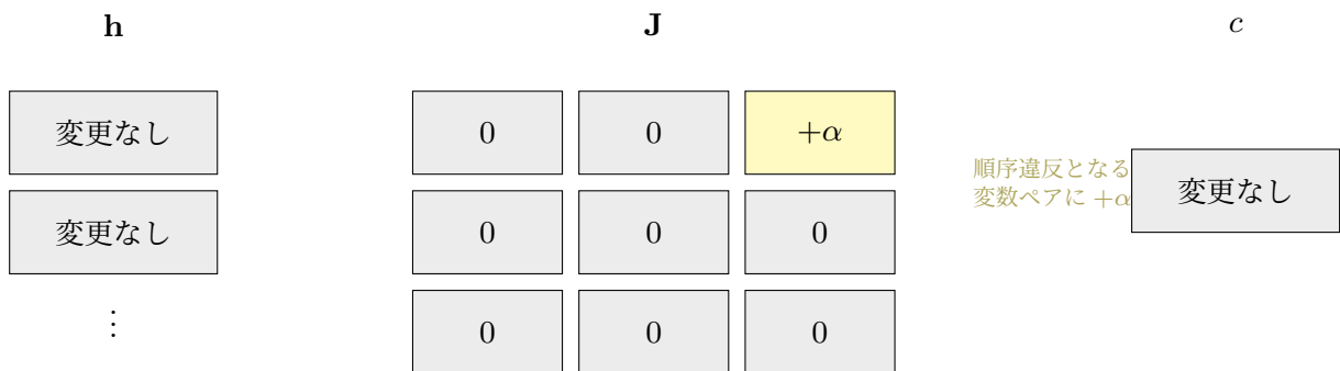
図 5.5 h_1 制約の係数加算. 順序違反となる変数ペア (i, j) に対して J_{ij} に +\alpha が加算される ( \alpha はペナルティ係数). h と c は変更なし.
