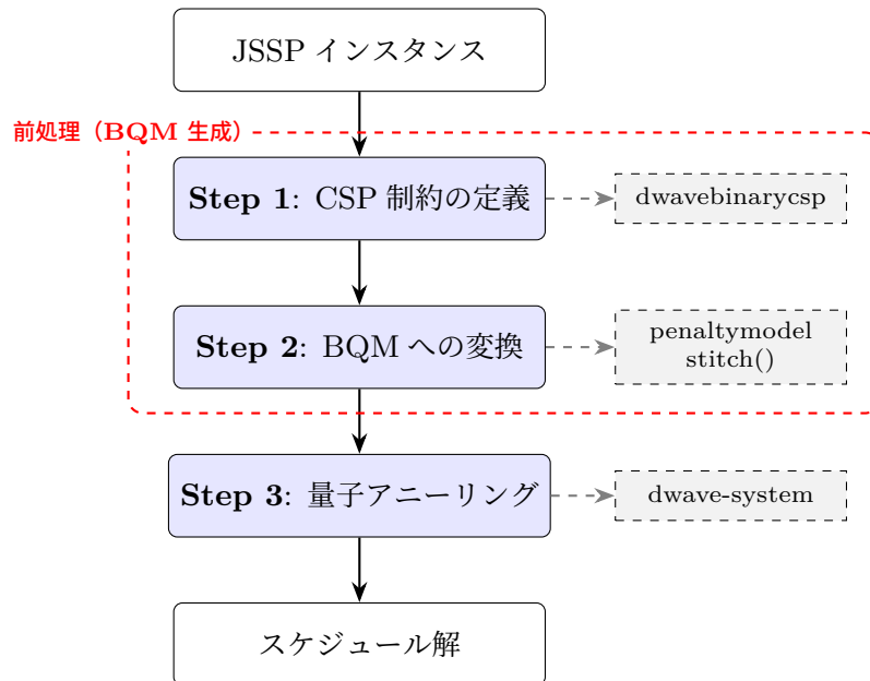
図 3.9 Carugno らの手法の全体フロー. JSSP インスタンスを CSP 形式で記述し, D-Wave のライブラリを用いて BQM に変換後, 量子アニーリングで求解する. 赤枠部分が前処理 (BQM 生成) であり, ボトルネックとなる.
