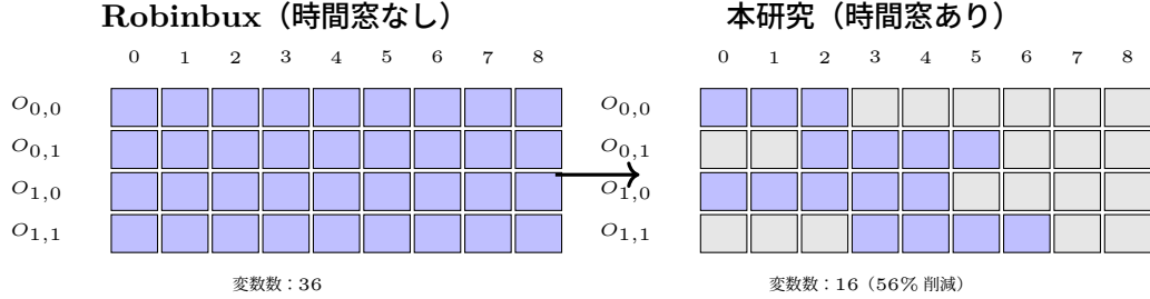
図 5.11 変数生成の比較. 左: Robinbux (全時刻に変数生成), 右: 本研究 (Venturelliらの時間窓計算に基づき時間窓内のみ生成)。
