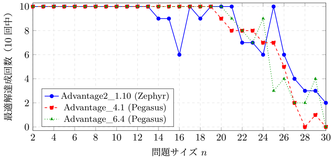
図 6.6 問題サイズに対する最適解達成回数の推移 ( n = 2 \sim 30 , 各 10 回試行)
