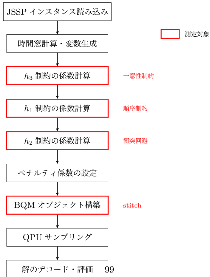
図 6.2 実験 1 の測定対象（赤枠：処理時間の測定箇所）
