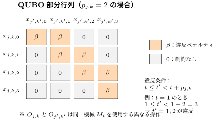
図 3.6 衝突回避制約における QUBO 部分行列の構造 ( p_{j,k} = 2 の場合)。行は操作 O_{j,k} の時刻変数、列は同一機械を使う別の操作 O_{j',k'} の時刻変数を表す。違反条件 t \leq t' < t + p_{j,k} を満たす (t, t') ペアに対して係数 \beta が設定される。
