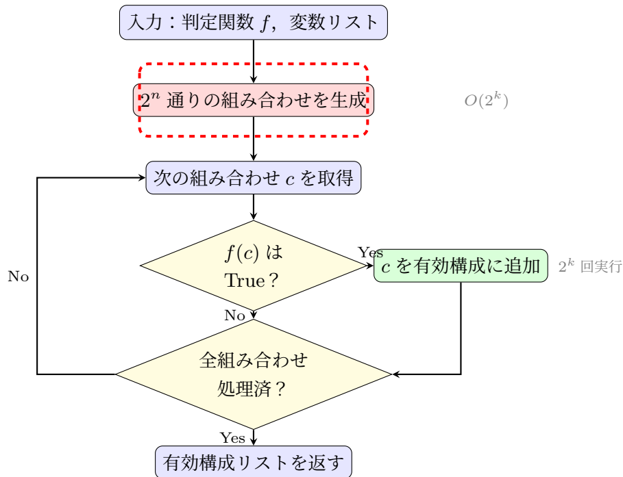
図 4.8 from_func メソッドの内部処理フロー. 赤破線部分で 2^k 通りの全列挙が発生し ( k は制約内変数数), 各組み合わせに対して判定関数が呼び出される.
