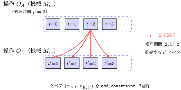
図 A.5 衝突回避制約のペア生成. 同一機械上の操作 O_A と O_B について, 処理期間が重複しうる時刻ペアに制約を登録する.
