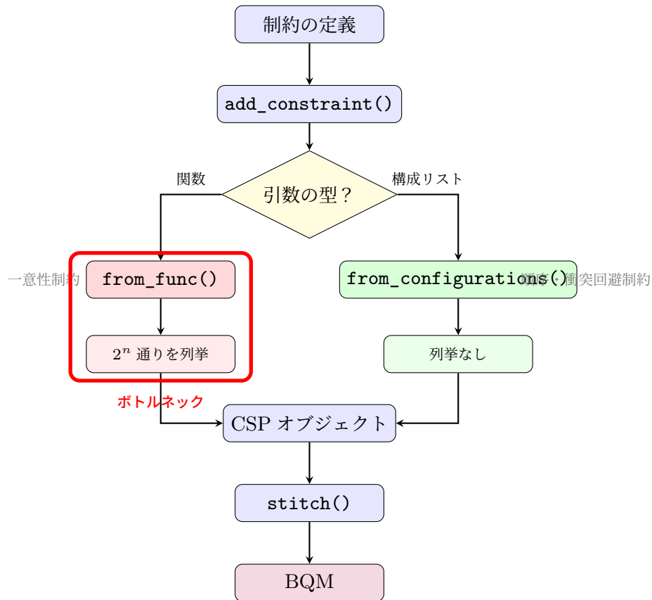
図 4.7 dwavebinarycsp による BQM 生成フロー。引数の型により内部処理が分岐する。 from_func (赤) は 2^n 列挙を伴い、 from_configurations (緑) は列挙なしで処理される。 n は制約に関係する変数の数であり、一意性制約では n = T (時刻変数の数) となる。実装箇所： from_func は dwavebinarycsp/core/constraint.py の 130–183 行目 (特に 179–181 行目で itertools.product による全列挙), from_configurations は同ファイル 186–232 行目, stitch は dwavebinarycsp/compiler/stitcher.py の 30–181 行目。
