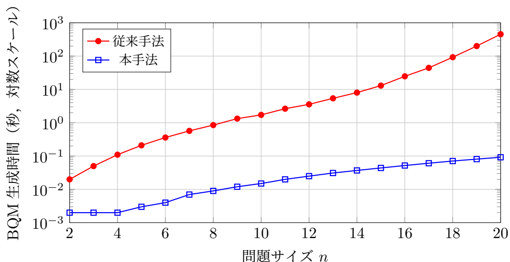
図 6.4 問題サイズと BQM 生成時間の関係 (対数スケール). 従来手法は指数的に増加するのに対し, 本手法は緩やかな増加にとどまる.
