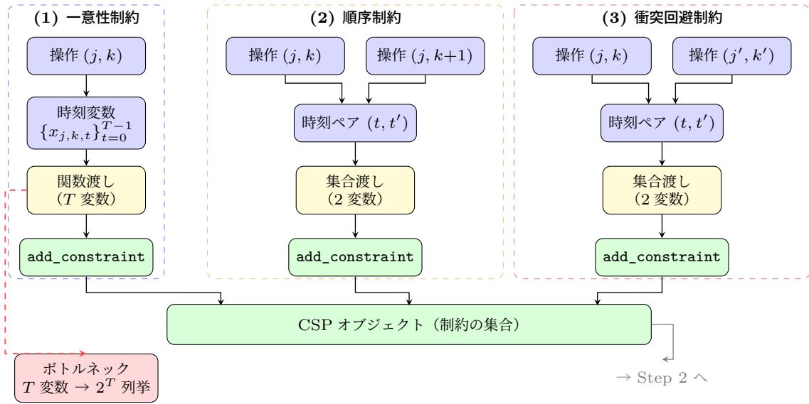
図 4.2 Step 1 の詳細フロー．(1) 一意性制約は T 個の変数を関数渡しで登録するため、後段で 2^T 列挙が発生しボトルネックとなる．(2)(3) は 2 変数の集合渡しで登録される．
