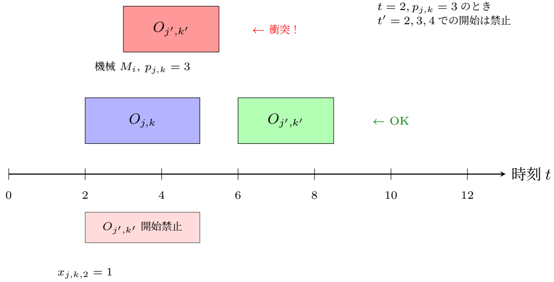
図 3.5 衝突回避制約の概念. 操作 O_{j,k} が時刻 t に開始し処理時間 p_{j,k} の場合, 同一機械を使う他の操作 O_{j',k'} は時刻 t から t + p_{j,k} - 1 の間は開始できない.
