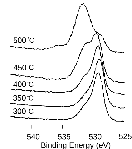
図 2: 基板温度と \text{O}(1s) XPS スペクトルの相関
