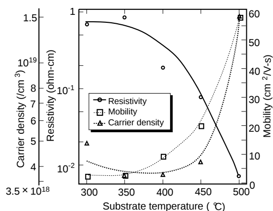
図 1: 基板温度と伝導特性の相関
