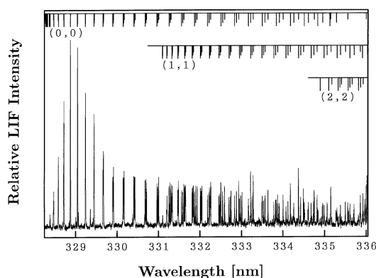
図 1: NH の LIF スペクトル
