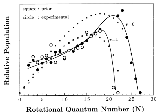
図 2: NH の回転・振動状態分布
