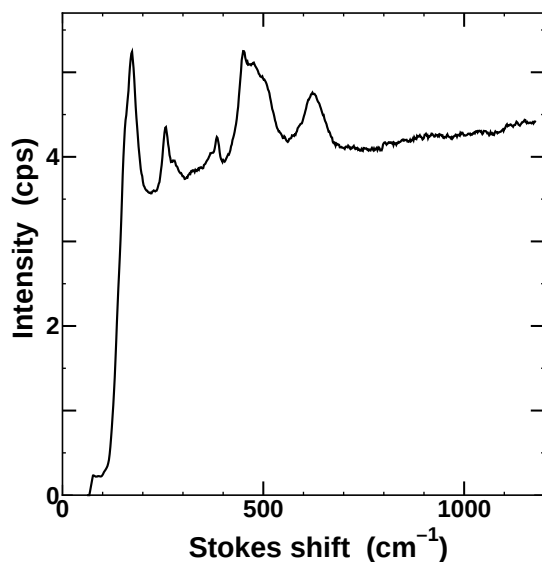
図 1: \alpha 型構造 \text{TiCl}_3 のラマンスペクトル
