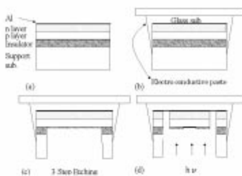
図 1: 薄膜 c-Si 太陽電池作製プロセス
