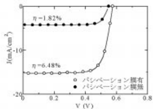
図 2: 薄膜 c-Si 太陽電池の電流電圧特性
