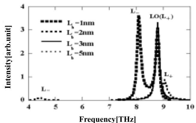
図 2. 縦振動電場のスペクトル強度
