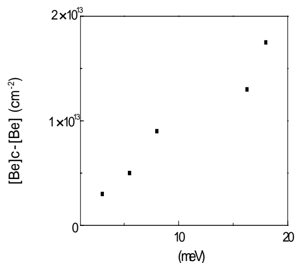
図1 デルタドーパ層のBe濃度[Be]の転移濃度[Be] c との差異と比抵抗の活性化エネルギーの関係
