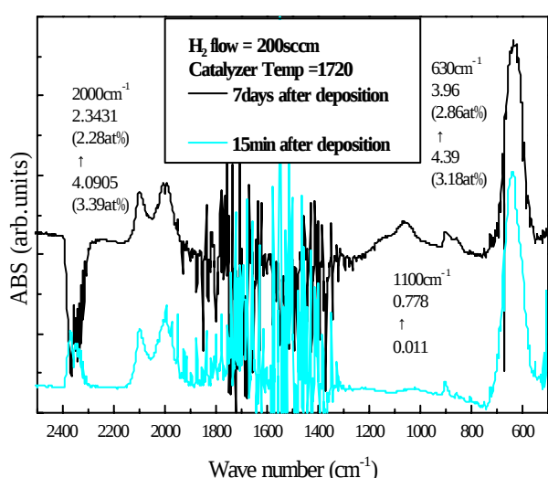
図1 赤外吸収スペクトルの時間変化とピーク面積の変化
