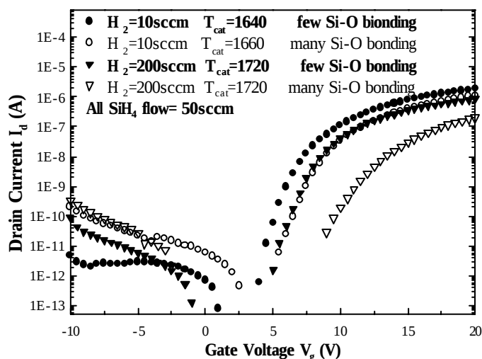
図2 処理工程による I_d - V_g 特性の変化と差異
