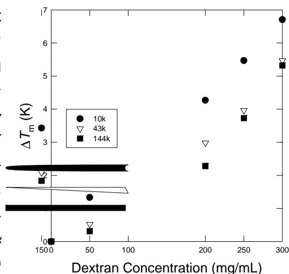
図 1 デキストラン濃度がリボヌクレアーゼ A の熱安定性に与える影響
