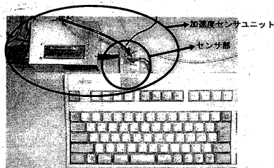
図 2: キーボードに取り付けた加速度センサ
