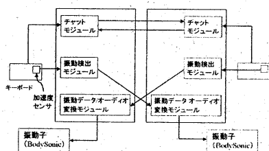
図 1: ソフトウェア構成
