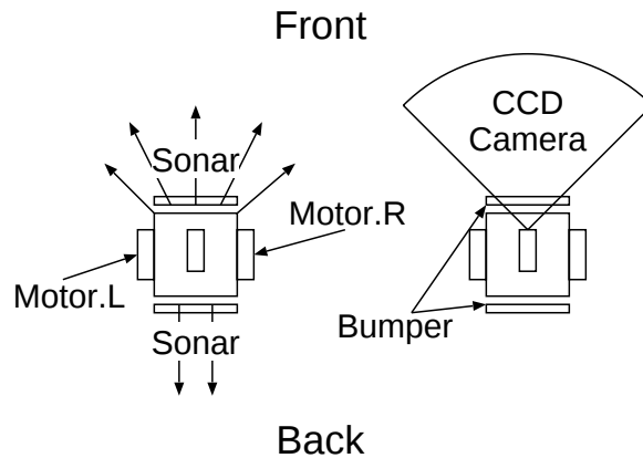
図 4.1: シミュレーション上のロボット
