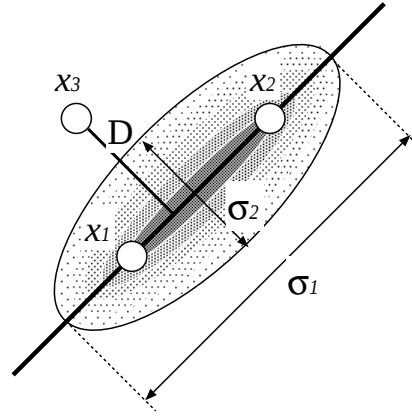
図 A.1: UNDX による交叉
