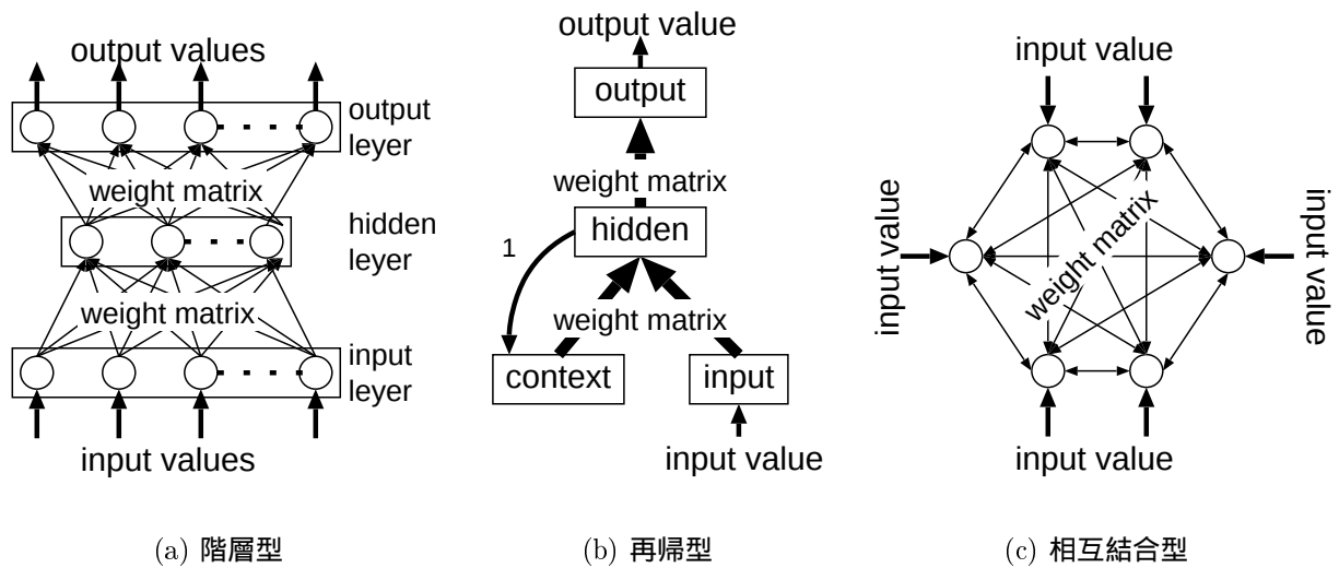
図 2.4: ネットワーク構造
