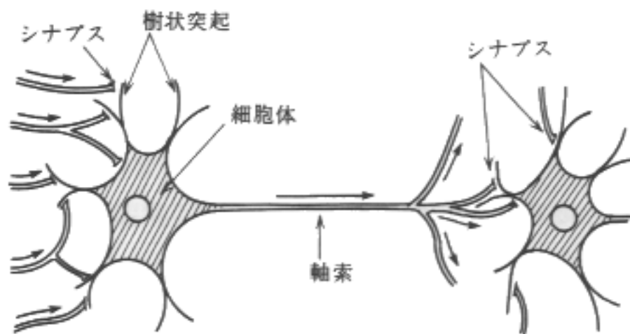
図 2.1: 生体ニューロンの構成
