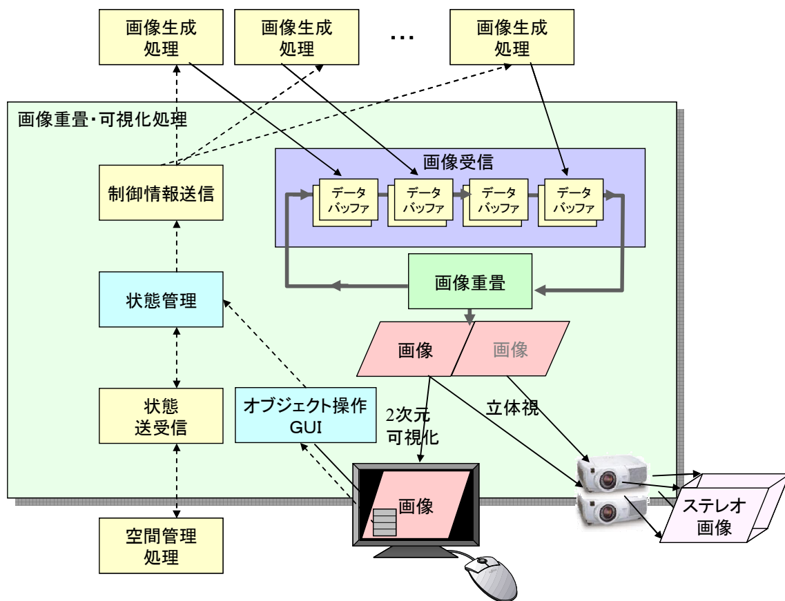
図 4.14 画像重畳・表示処理フロー
