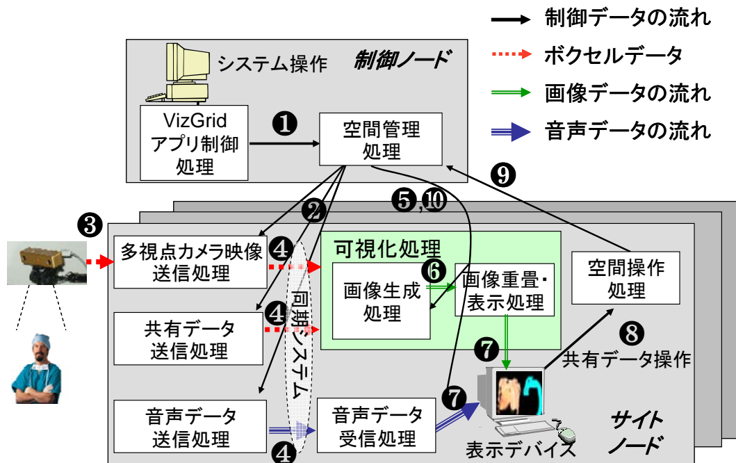
図 4.17 VC 手法による会議制御処理の流れ
