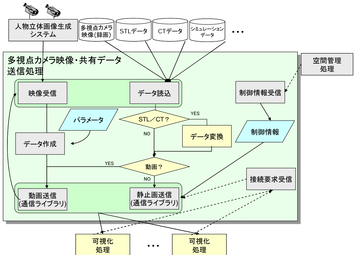
図 4.6 多視点カメラ映像・共有データ送信処理フロー
