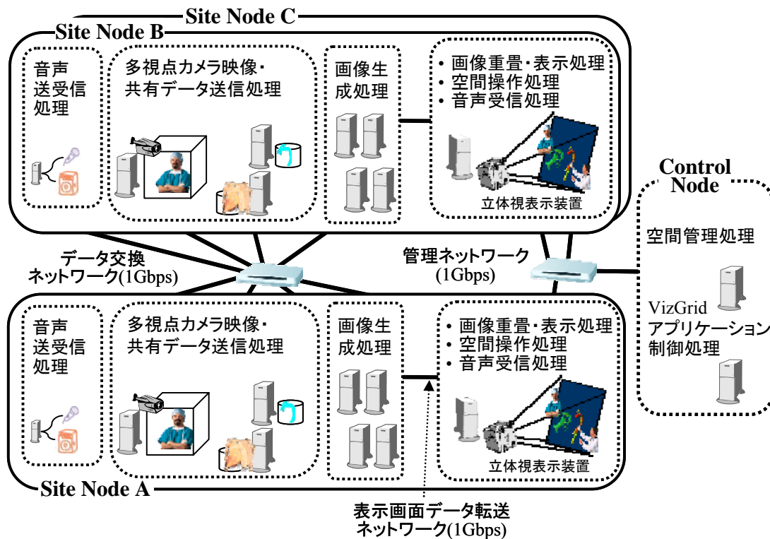
図 5.2 処理の計算機システムへの配置
