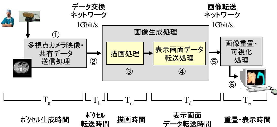
図 6.1 可視化処理とデータの流れ
