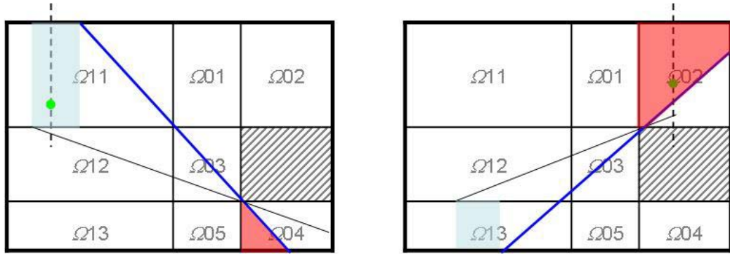
図 3-7 制限付け遷移の対処法
