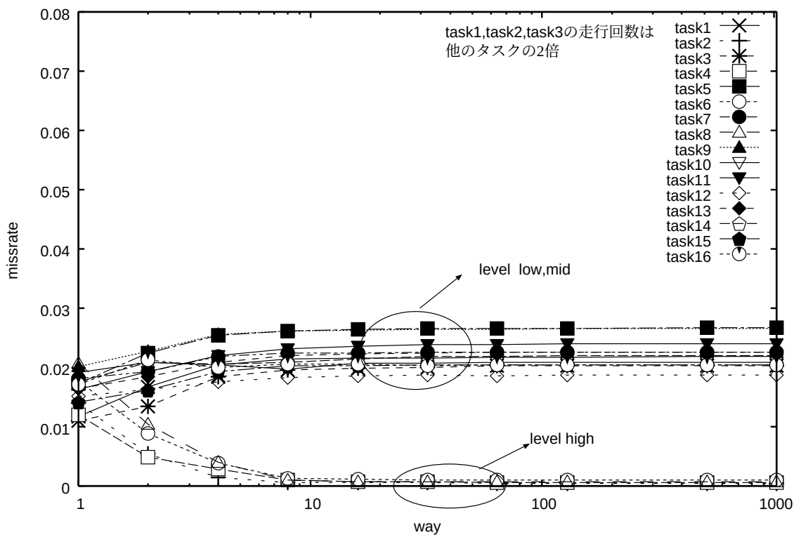
図 8.4: 静的な優先度に基づいた置換制御を行った場合のミス率
