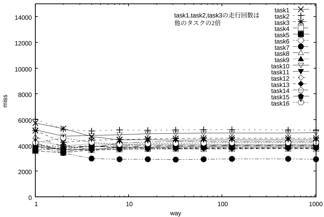
図 8.1: 通常の LRU で置換制御を行った場合のミス回数
