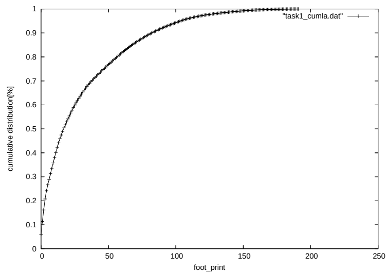
図 6.2: タスク 1 のアクセス回数の累積分布
