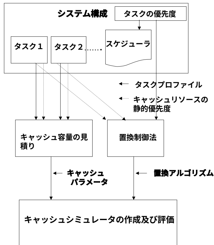
図 6.1: 実験の全体図
