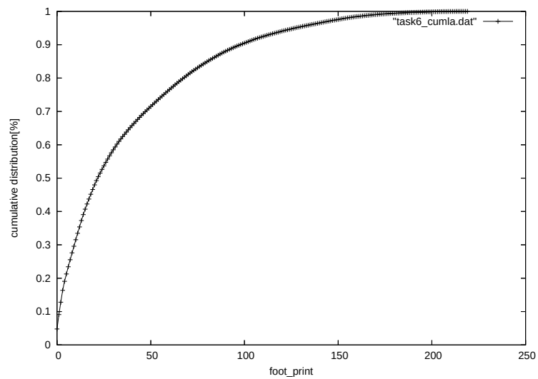
図 6.7: タスク 6 のアクセス回数の累積分布
