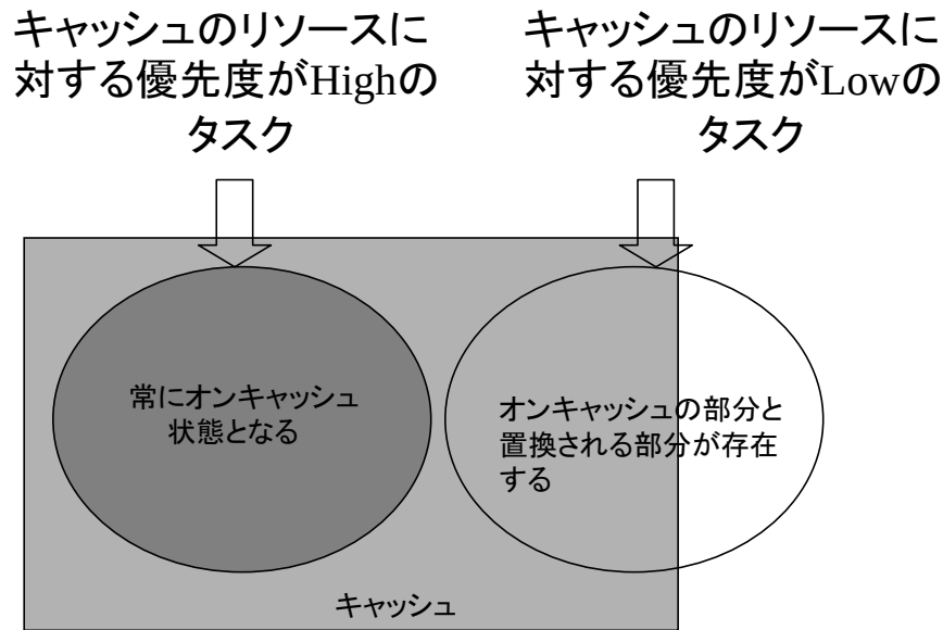
図 5.2: 高い優先度を割りあてられたタスクのキャッシュ内での様子
