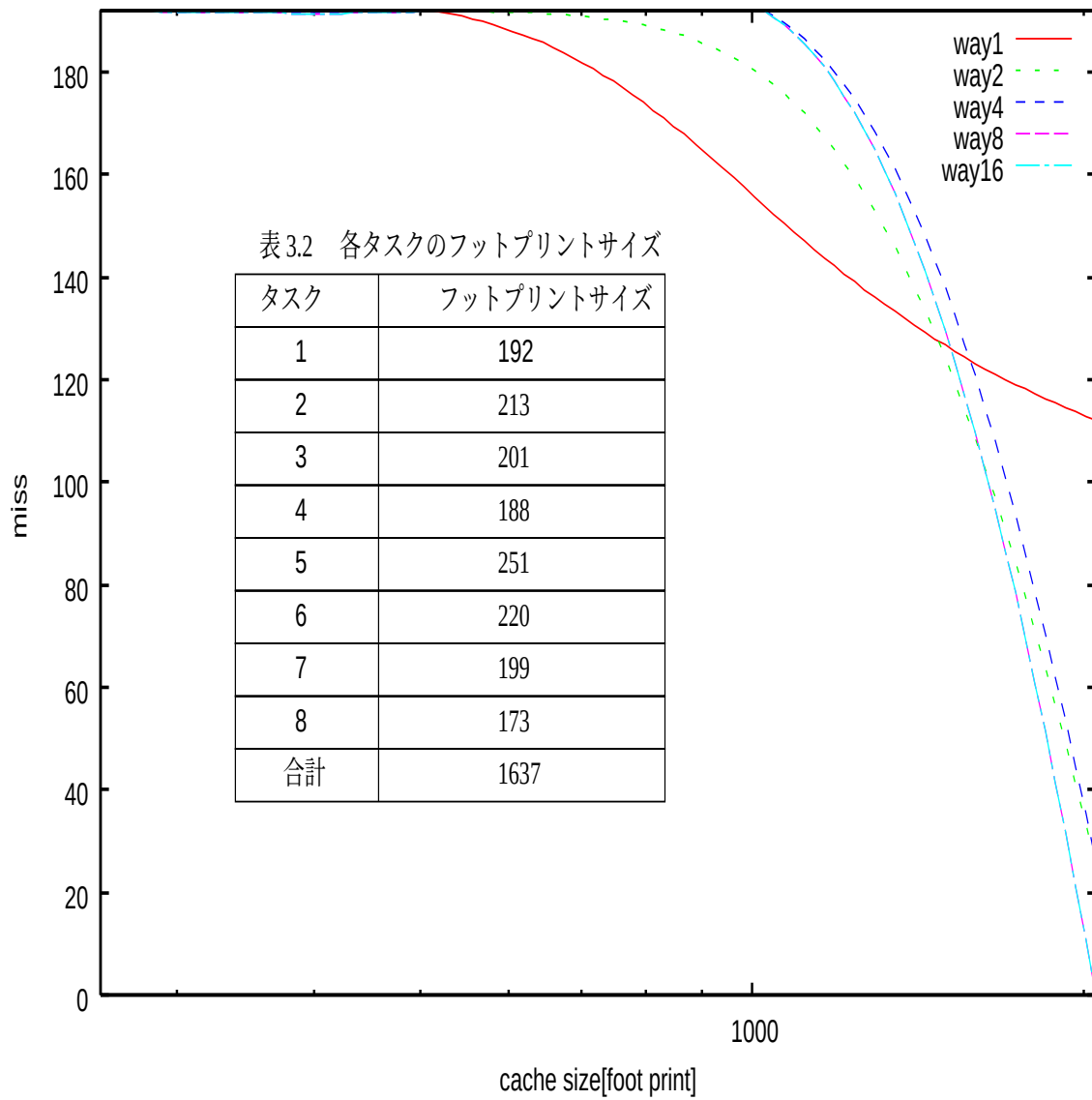
図 3.3: シミュレーションによるキャッシュの再ロード過渡状態
