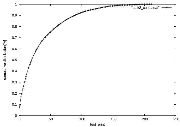
図 6.3: タスク 2 のアクセス回数の累積分布
