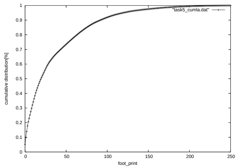
図 6.6: タスク 5 のアクセス回数の累積分布
