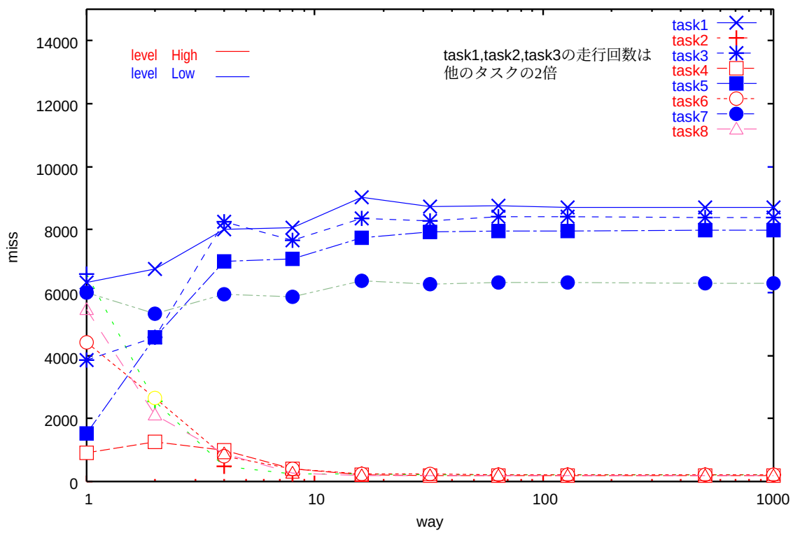
図 6.13: 静的な優先度に基づいた置換制御を行った場合のミス回数
