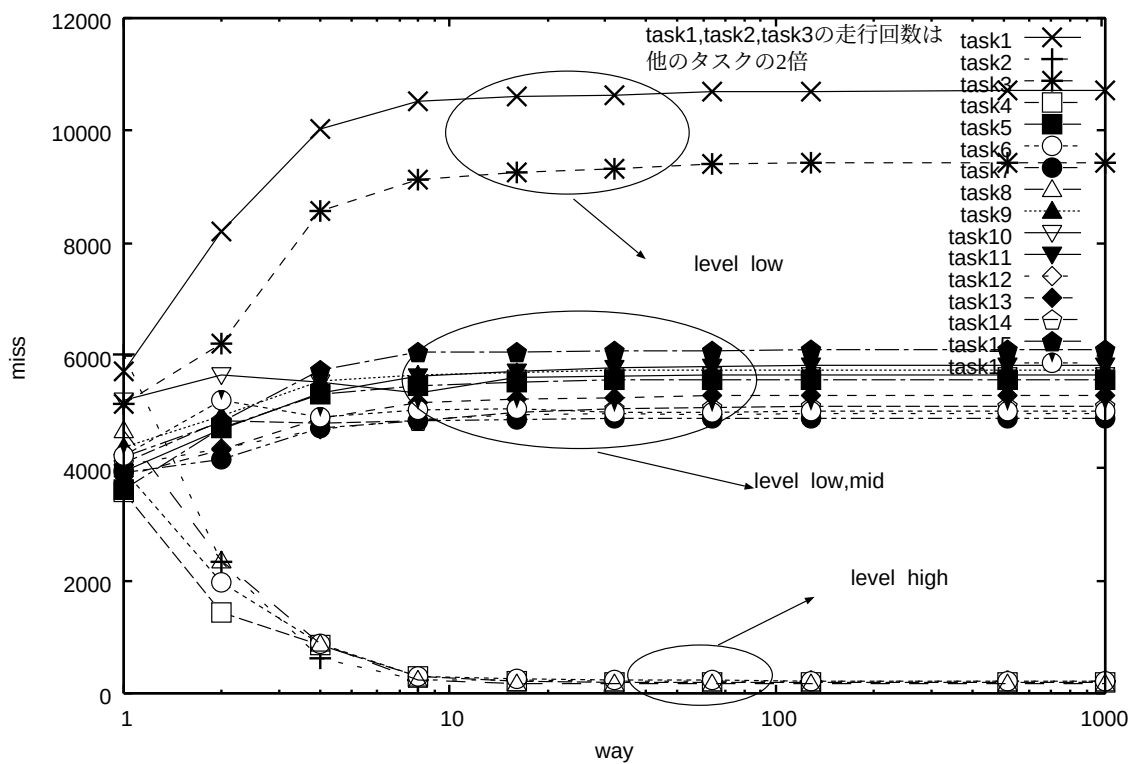
図 8.3: 静的な優先度に基づいた置換制御を行った場合のミス回数
