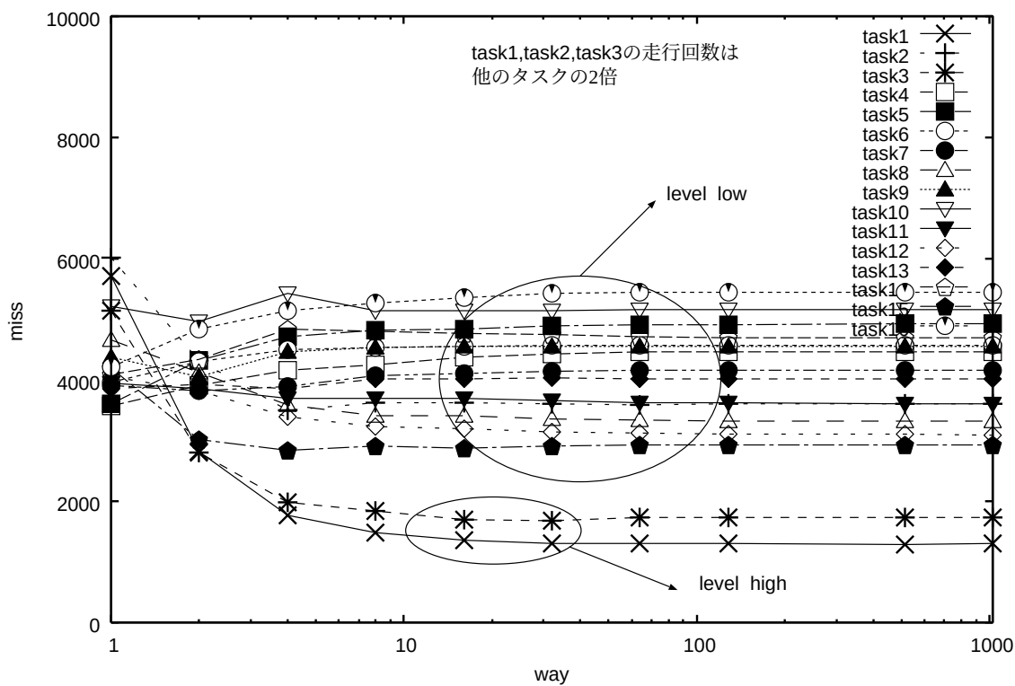
図 8.5: 動的優先度に基づいた置換制御を行った場合のミス回数
