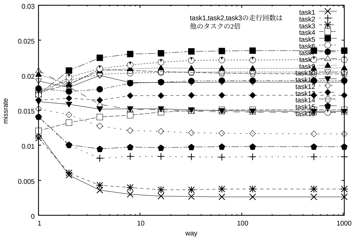
図 8.6: 動的優先度に基づいた置換制御を行った場合のミス率
