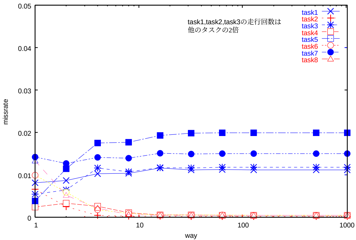
図 6.14: 静的な優先度に基づいた置換制御を行った場合のミス率
