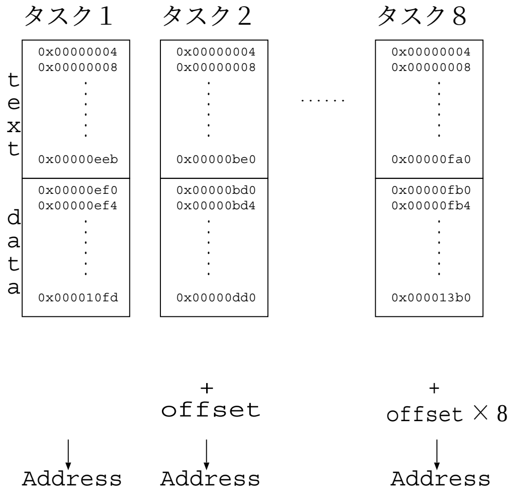
図 6.10: メモリ内の各タスク配置
