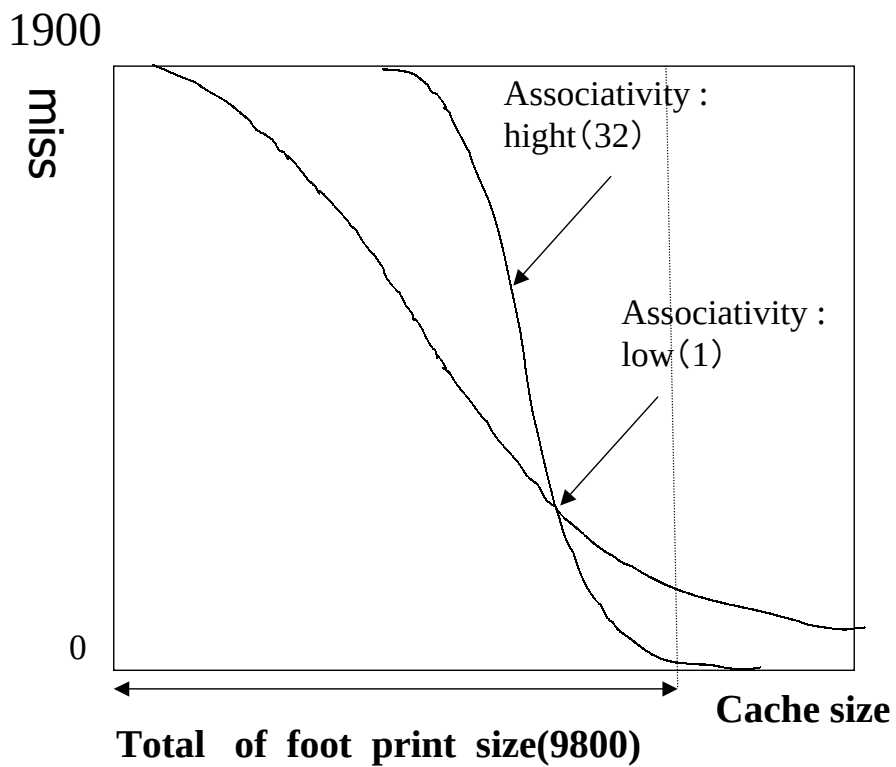
図 3.2: キャッシュの再ロード過渡状態
