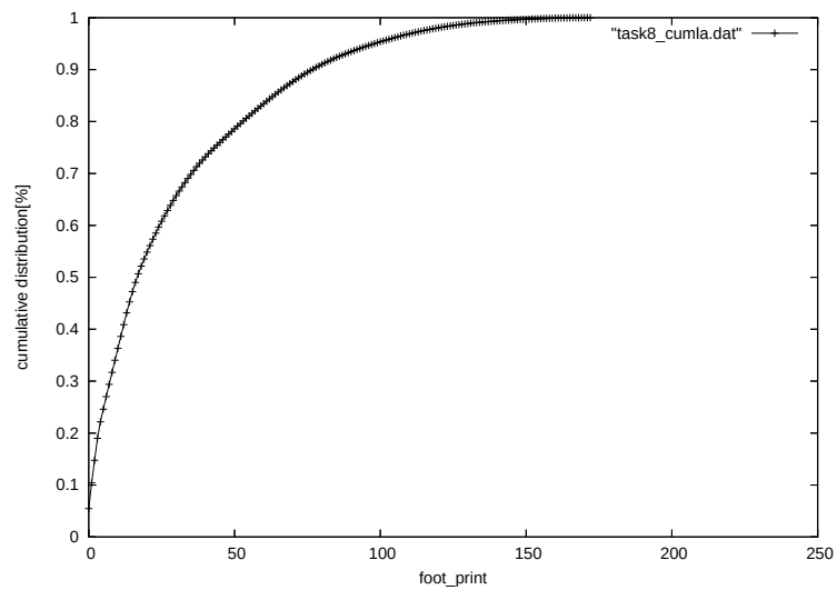
図 6.9: タスク 8 のアクセス回数の累積分布
