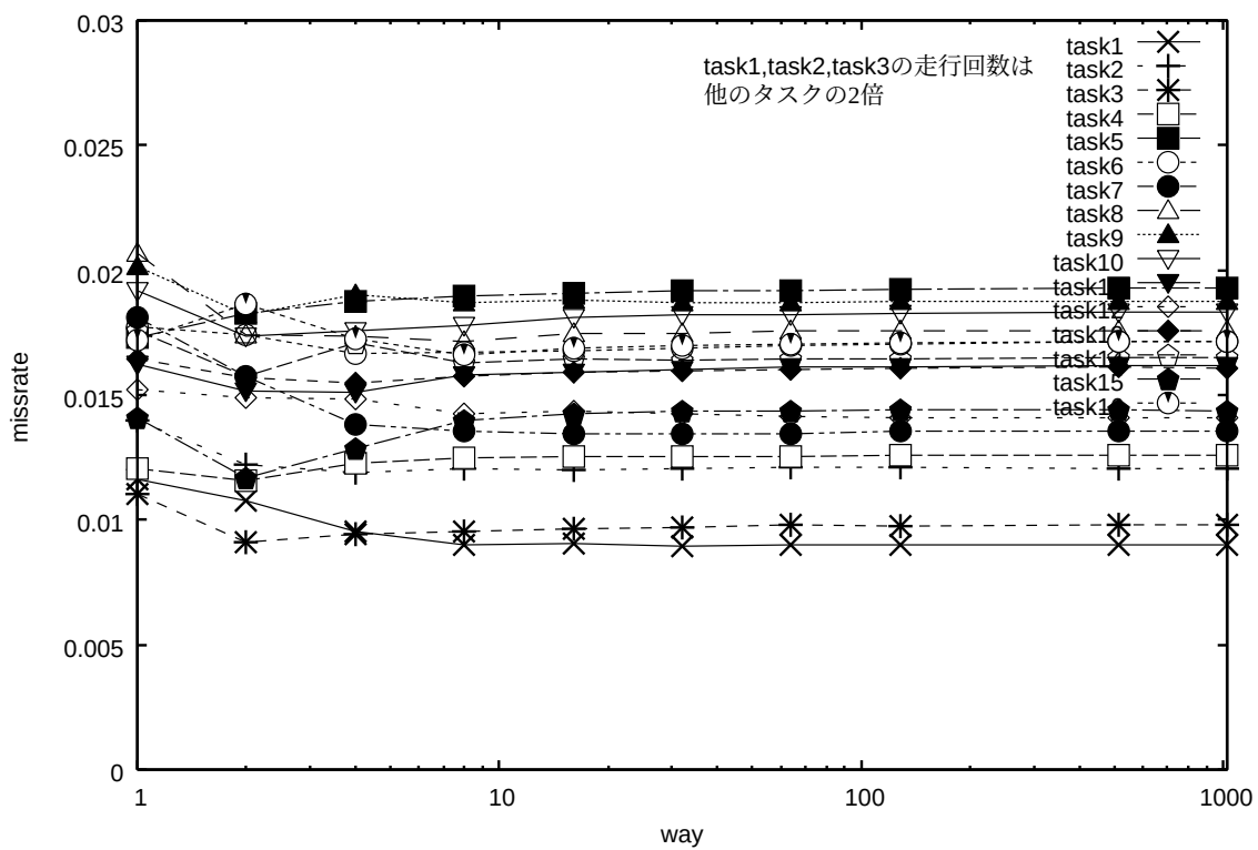
図 8.2: 通常の LRU で置換制御を行った場合のミス率
