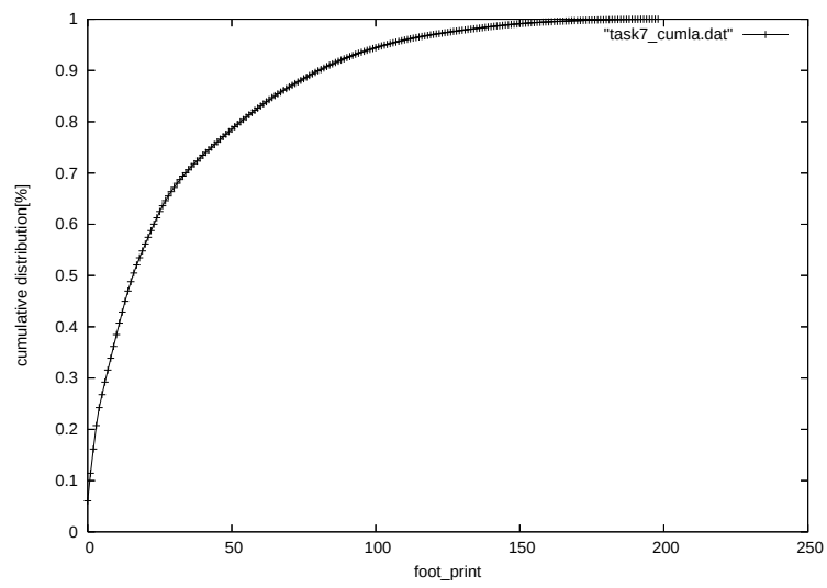
図 6.8: タスク 7 のアクセス回数の累積分布
