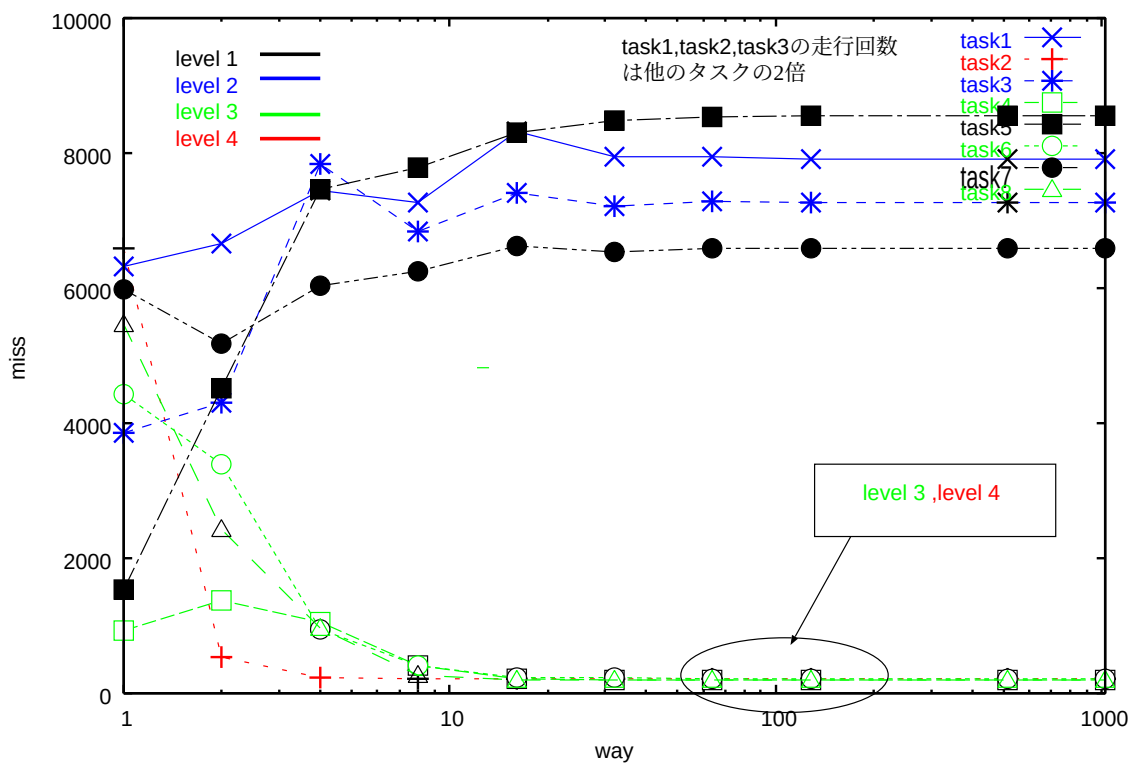
図 6.17: 動的な優先度と静的な優先度の組み合わせに基づいた置換制御を行った場合のミス回数
