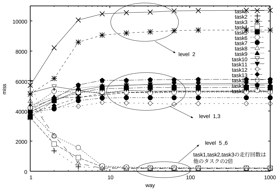
図 8.7: 動的な優先度と静的な優先度の組み合わせに基づいた置換制御を行った場合のミス回数
