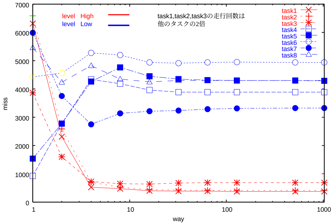
図 6.15: 動的な優先度に基づいた置換制御を行った場合のミス回数
