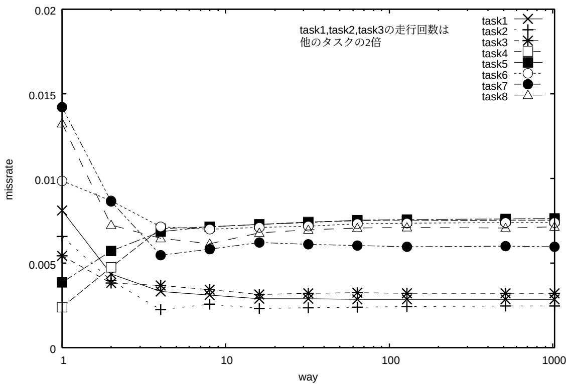
図 6.12: 通常の LRU で置換制御を行った場合のミス率
