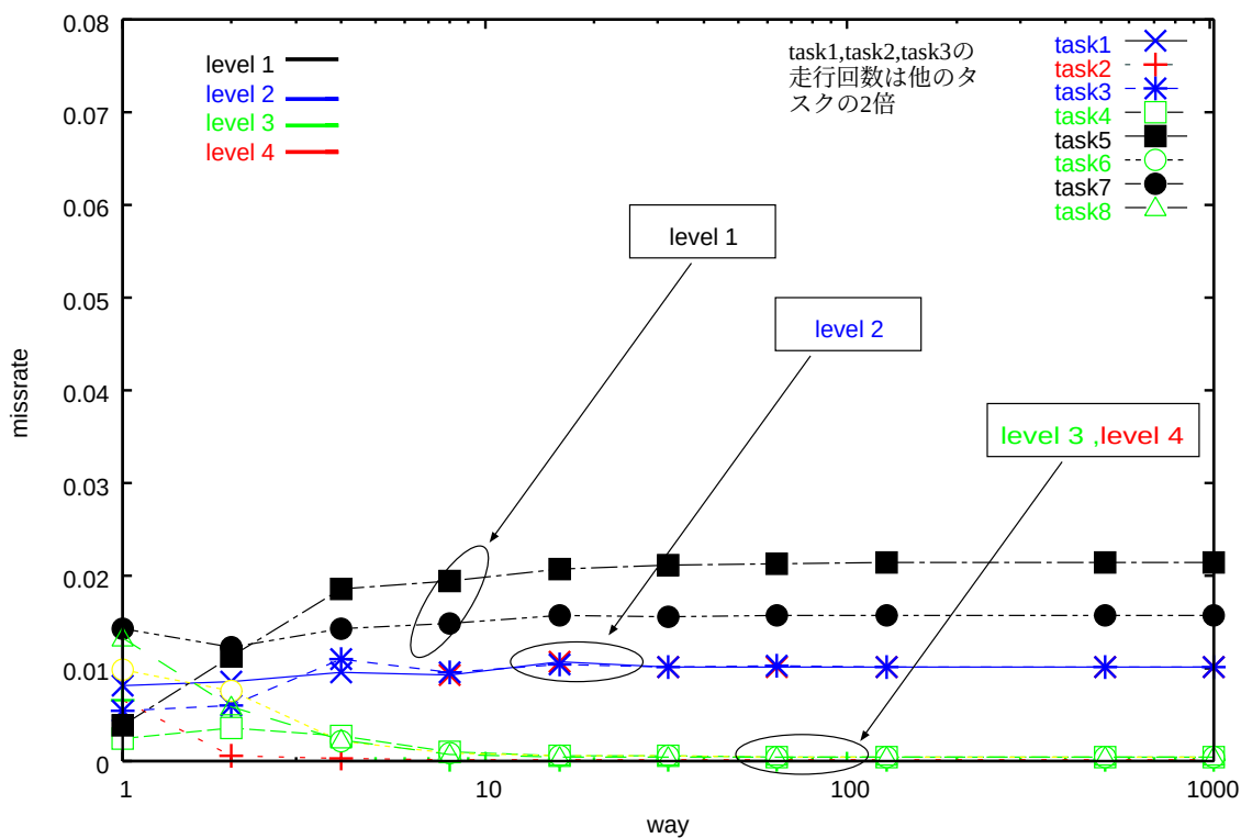
図 6.18: 動的な優先度と静的な優先度の組み合わせに基づいた置換制御を行った場合のミス率
