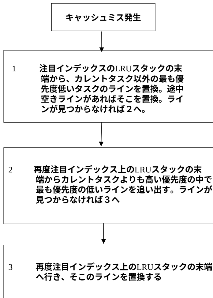
図 5.3: 置換アルゴリズム
