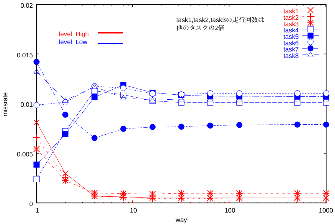
図 6.16: 動的な優先度に基づいた置換制御を行った場合のミス率
