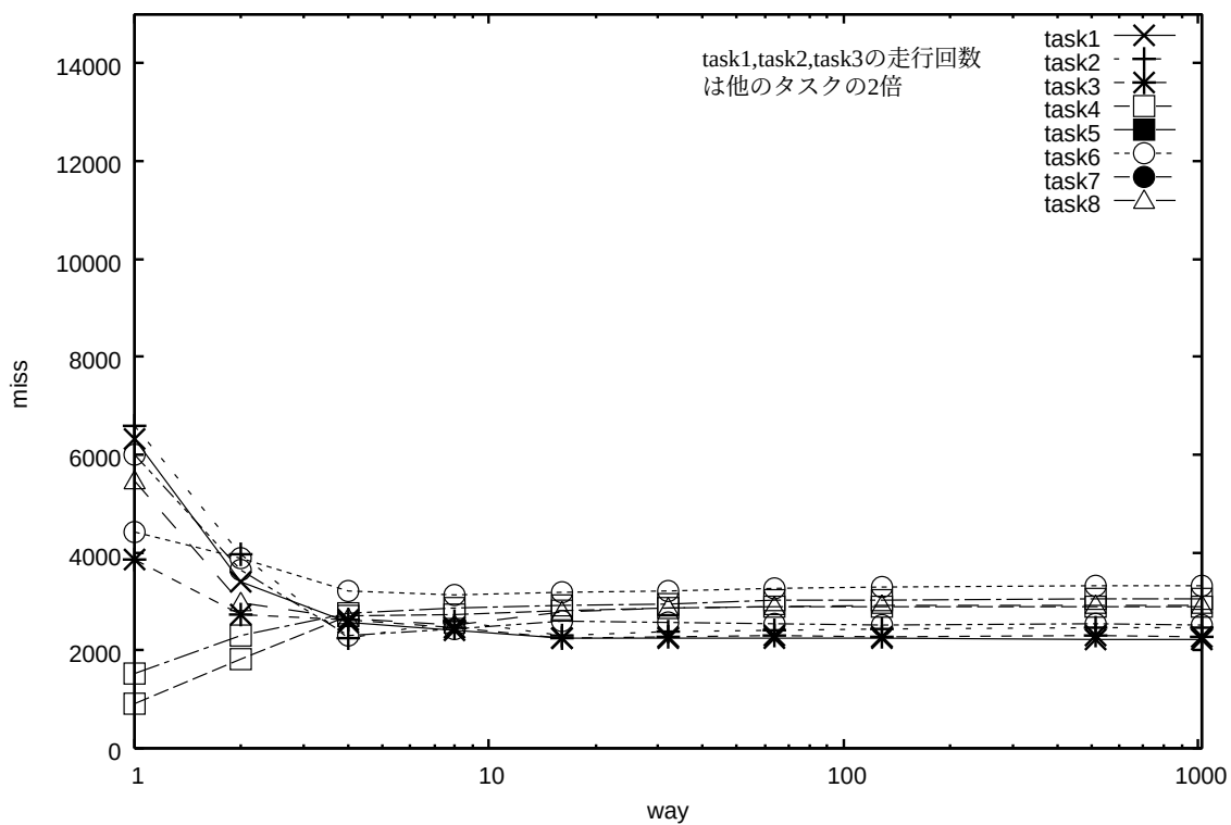
図 6.11: 通常の LRU で置換制御を行った場合のミス回数
