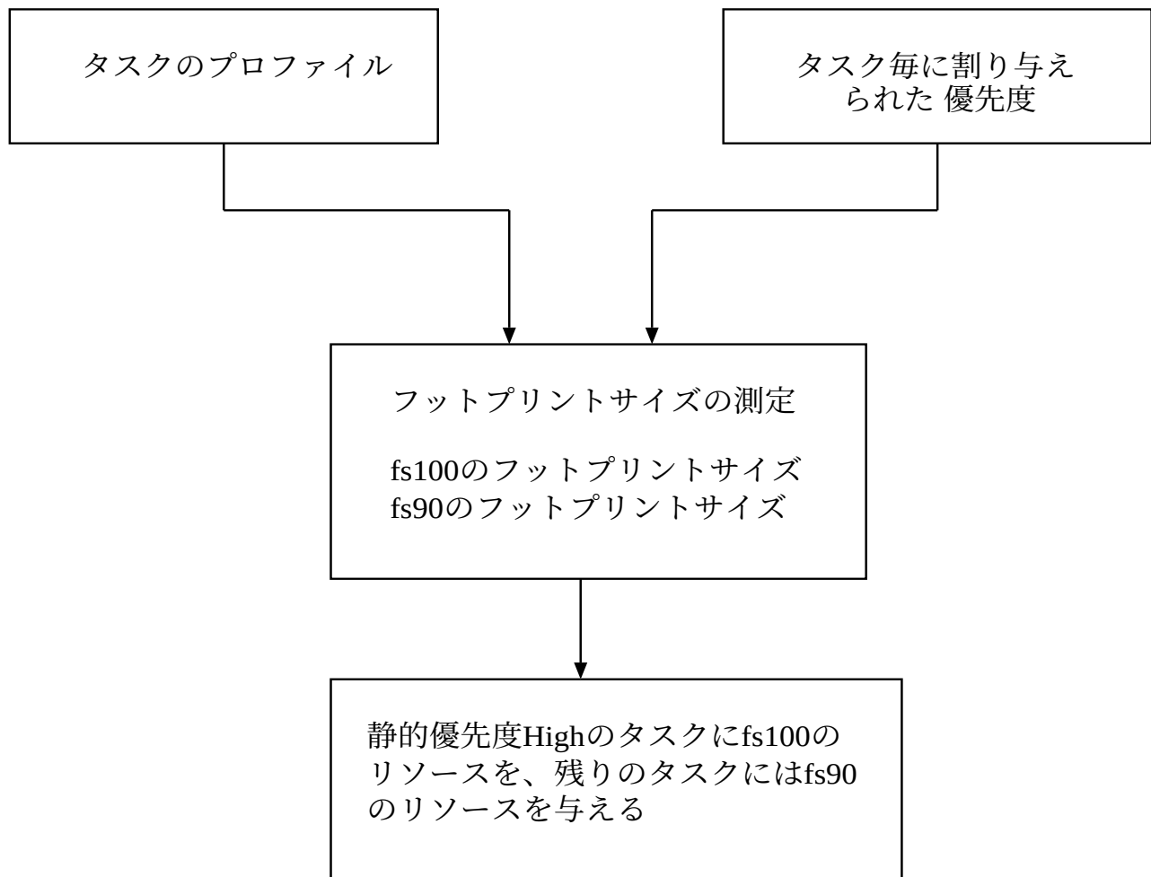
図 5.1: キャッシュ容量の見積り
