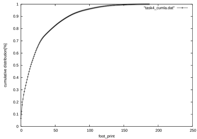
図 6.5: タスク 4 のアクセス回数の累積分布
