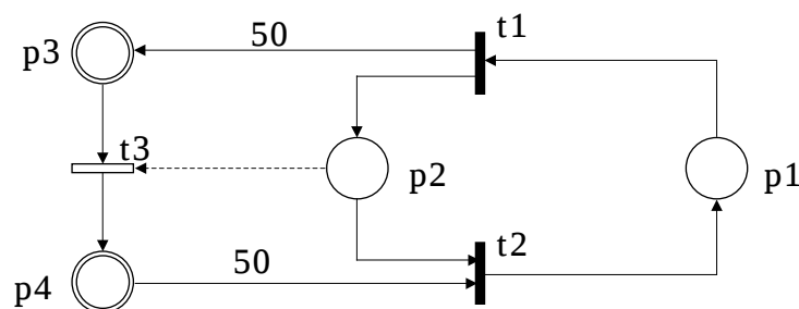
図4.3 ハイブリッドペトリネットの例
