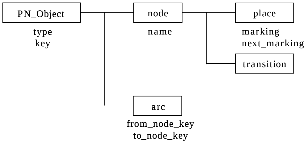
図3.1 クラス相関図
