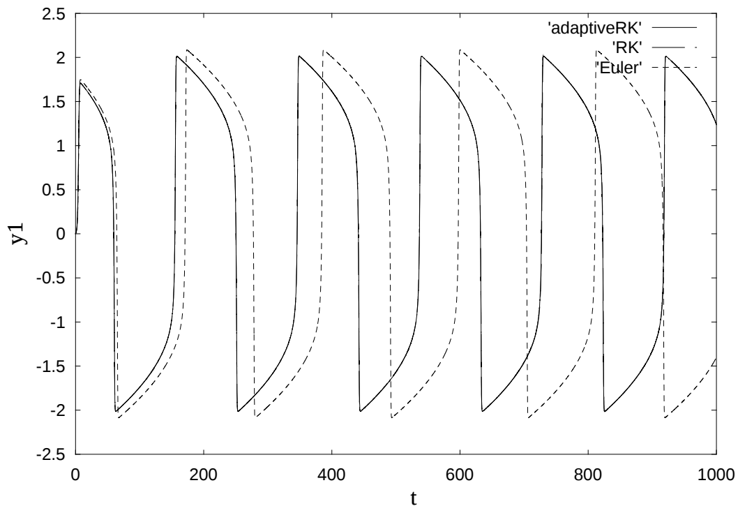
図 4.13 硬い系の計算結果 ( y_1 の時系列)
