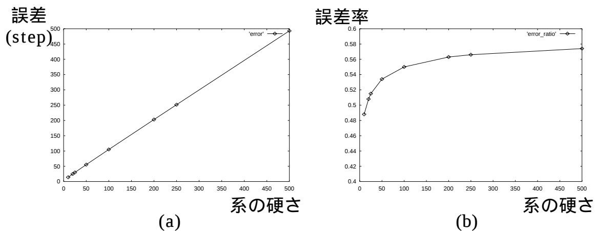
図 4.14 系の硬さを変えたときオイラー法とルンゲ・クッタ法の誤差と誤差率 (誤差としてオイラー法とルンゲ・クッタ法の第 5 周期の極大値が何ステップ目に表れるかの差をとった。誤差率はそれぞれの系の硬さに応じた周期の長さで誤差を割ることにより求めたものである。)
