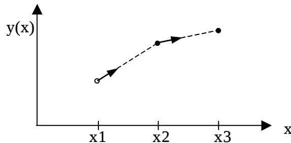
図4.5 オイラー法
