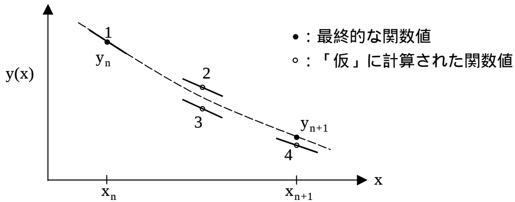
図4.7 4次のルンゲ・クッタ法
