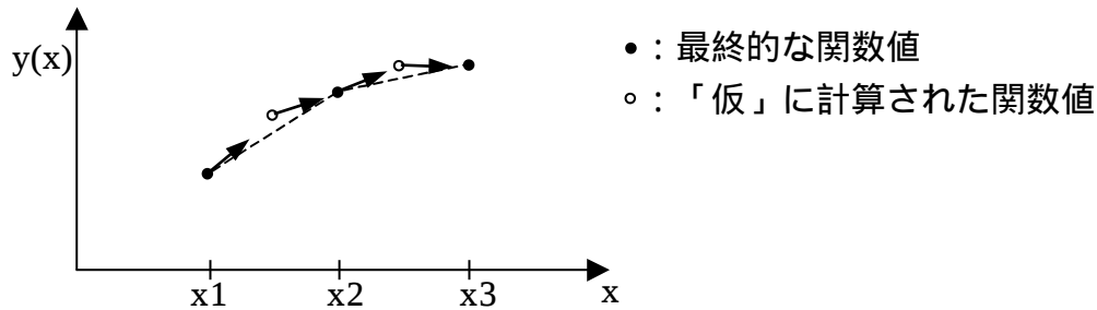
図4.6 2次のルンゲ・クッタ法(中点法)
