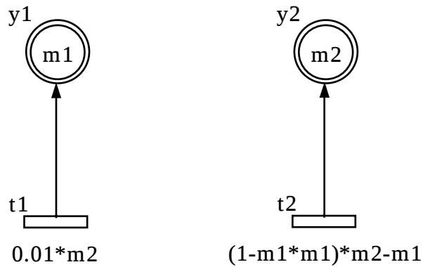
図4.12 ペトリネットを用いた硬い系(van der Pol方程式)の表示
