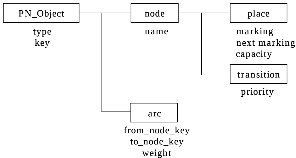
図3.4 クラス相関図
