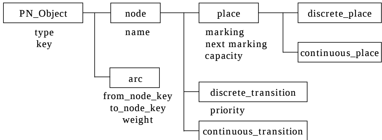
図4.2 クラス相関図
