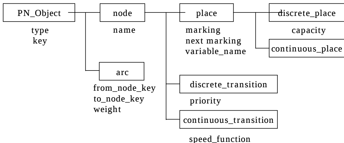
図4.8 クラス相関図
