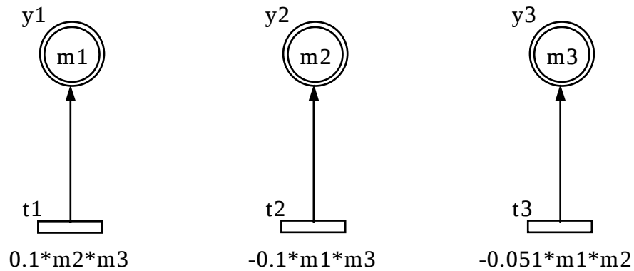
図4.9 ペトリネットを用いた外力のない剛体の挙動についての微分方程式系の表現
