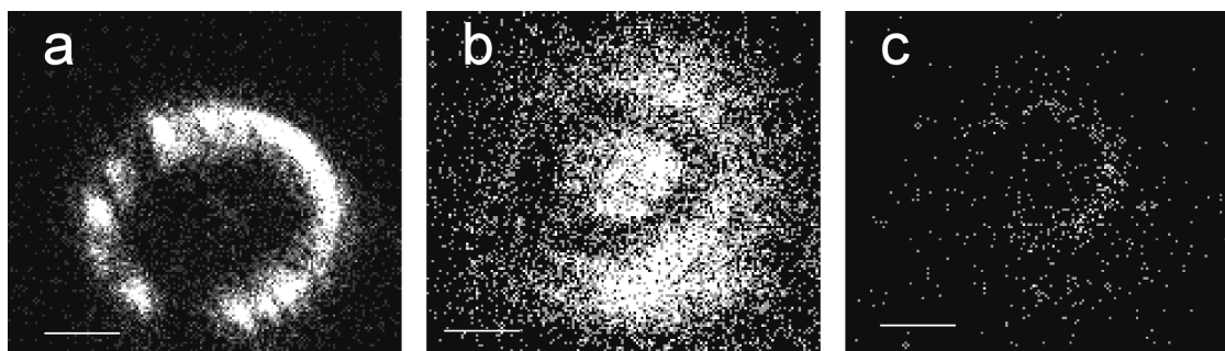
図 1. マイクロ秒のパルス幅の赤外光を照射した H-Si(111)表面の SH、SF 顕微像 (a) SH 顕微像、(b)SF 顕微像(2080 \text{cm}^{-1} )、(c) SF 顕微像(2092 \text{cm}^{-1} ) Scale bars: 200 \mu\text{m}
