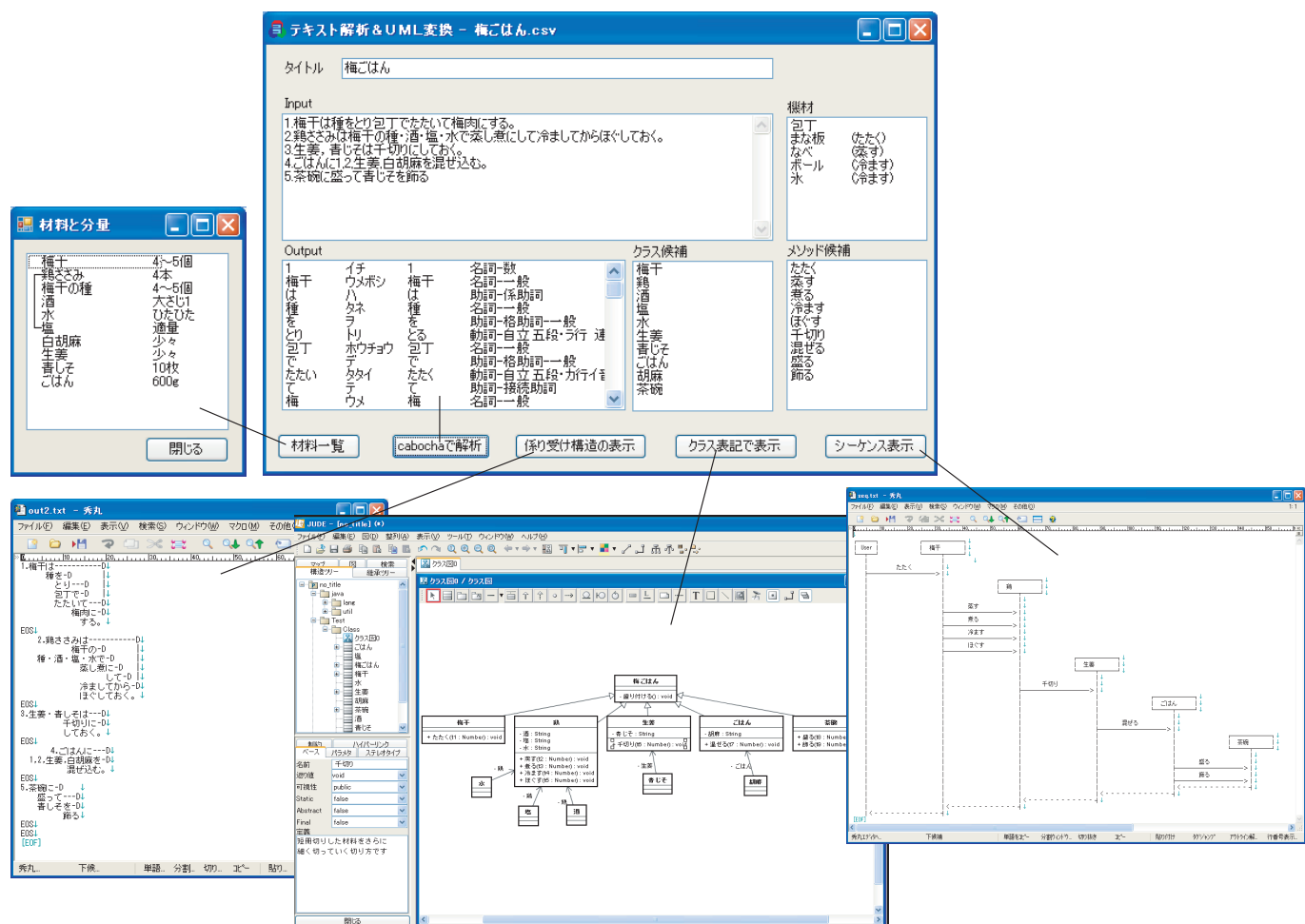
図 5.7: 料理レシピの UML 変換の全体像
