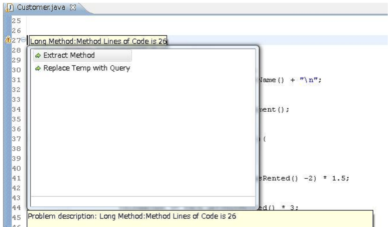
図 5.4: BadSmell を解消するためのリファクタリング操作候補の表示
