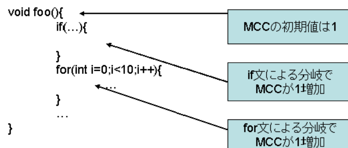
図 2.11: MCC の測定例
