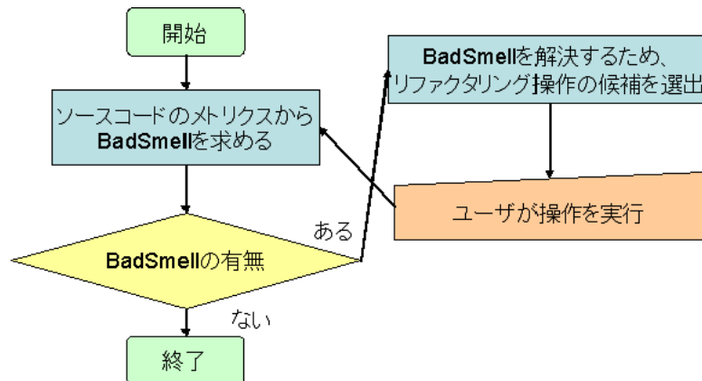
図 3.1: 支援の自動化によるリファクタリングの流れ
