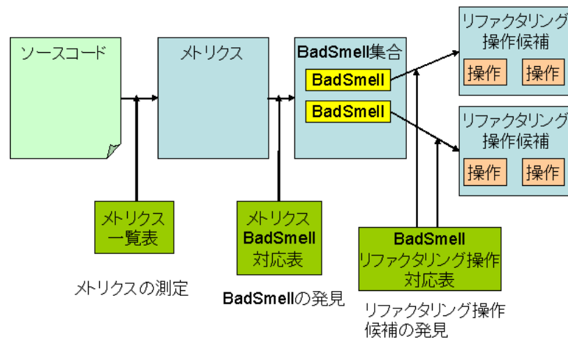
図 4.2: リファクタリング操作候補を求めるまでの流れ
