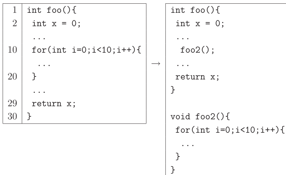
図 2.12: Long Method に対してメソッドの抽出を行った場合
