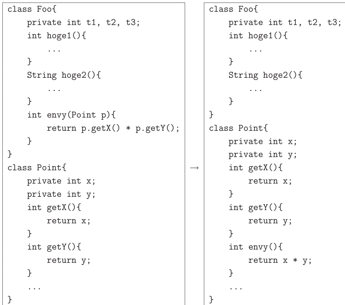
図 2.6: メソッドの移動の例
