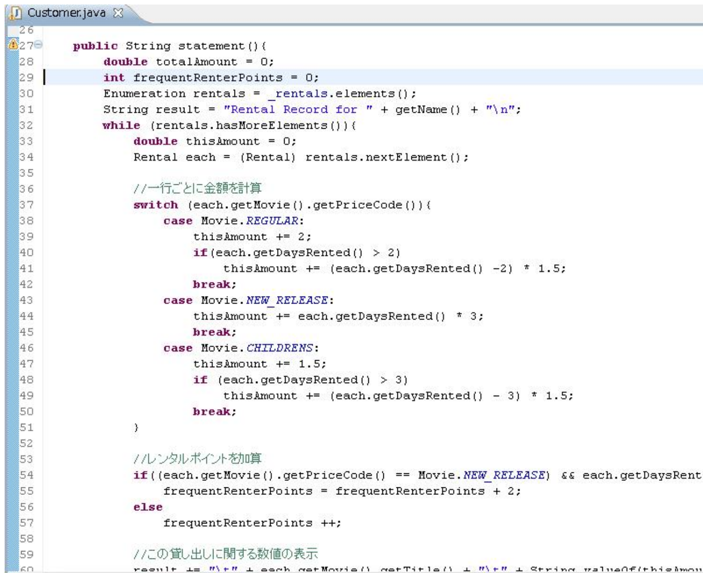
図 5.3: エディタ部分に対しての BadSmell の視覚的表現
