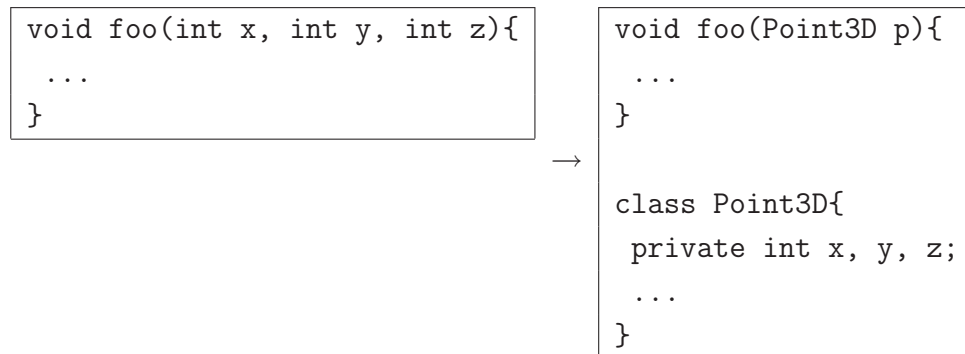
図 2.10: 引数オブジェクトの導入の例
