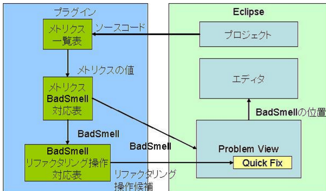
図 5.1: ツールによる支援の全体構成図
