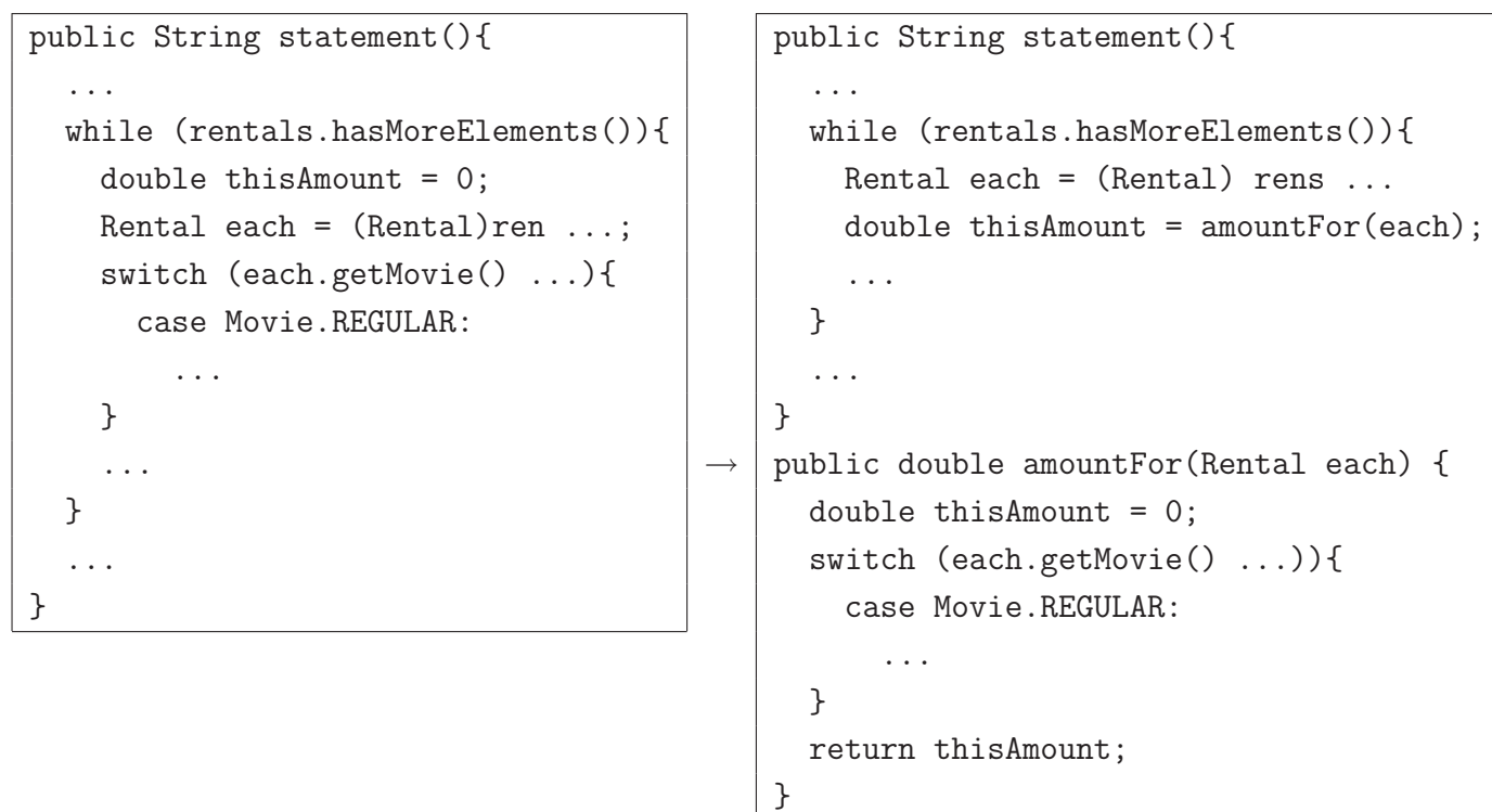
図 6.4: amountFor メソッドを抽出
