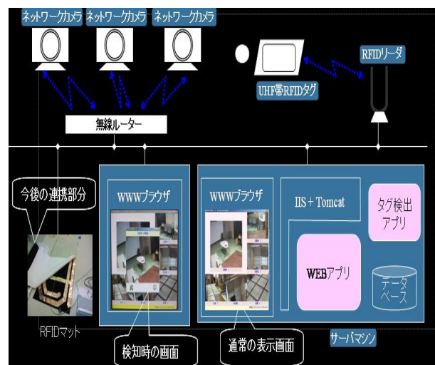
図 9 実験用協調介護支援システム
