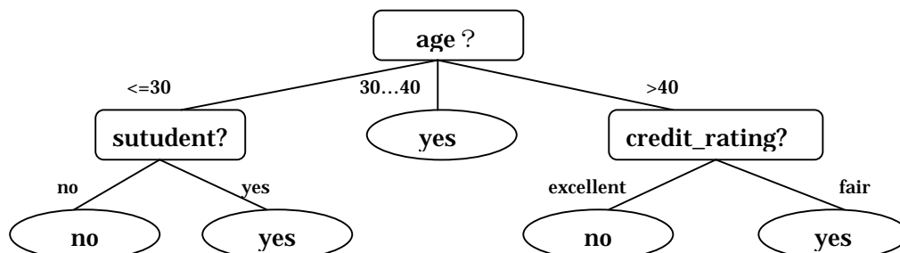
図 2.2 決定木
