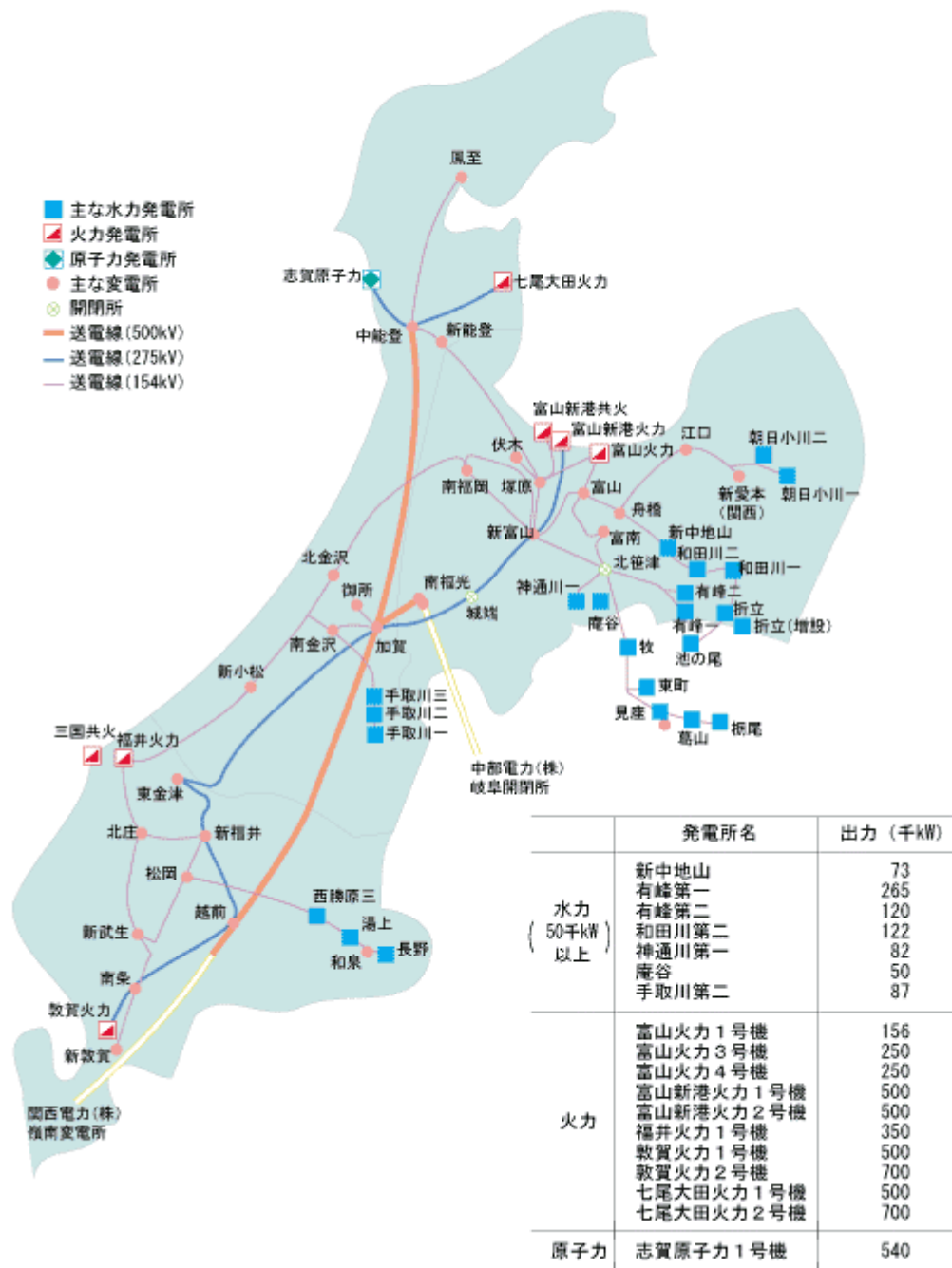
図 2.3 : 北陸地域の電力系統図
