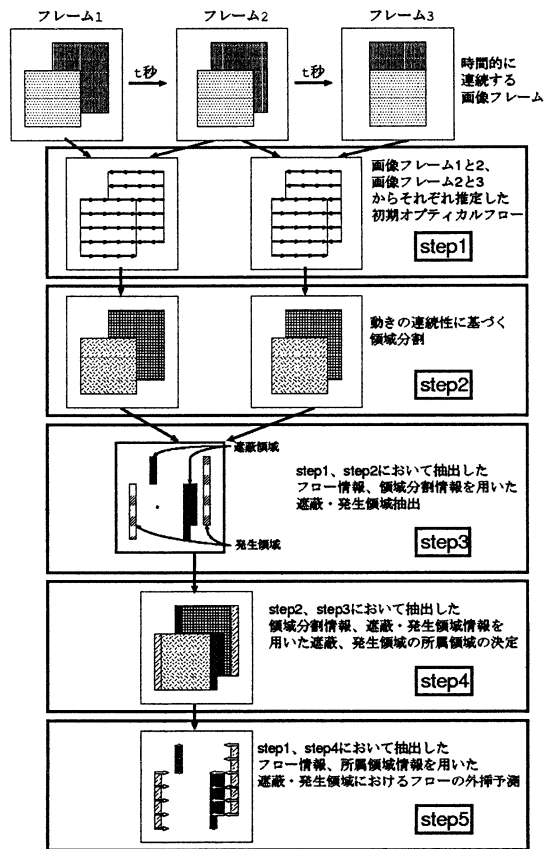
図 3 遮へい・発生領域におけるフローの外挿予測の処理過程
