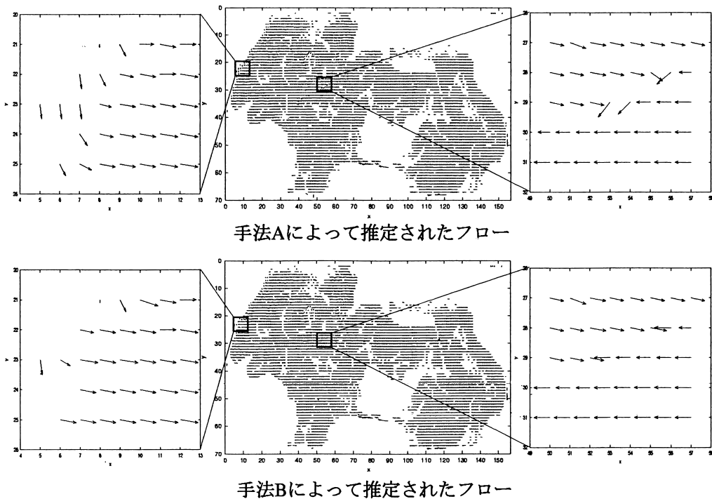
図 14 手法 A、手法 B による実画像に対するフロー推定結果
