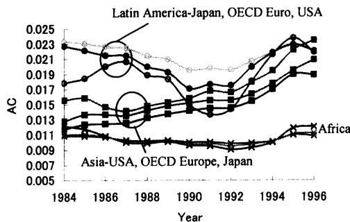
図6-1 各国・地域間の同化能力
