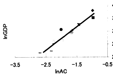
図4 同化能力とGDP
