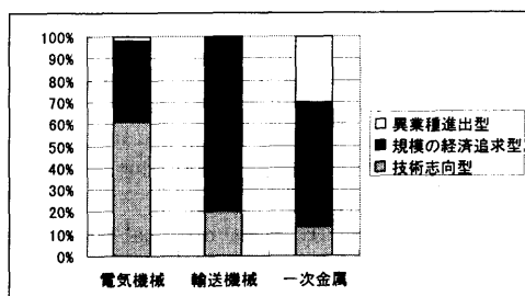
図3 各業種の提携パターンの割合 (1984-1999)
