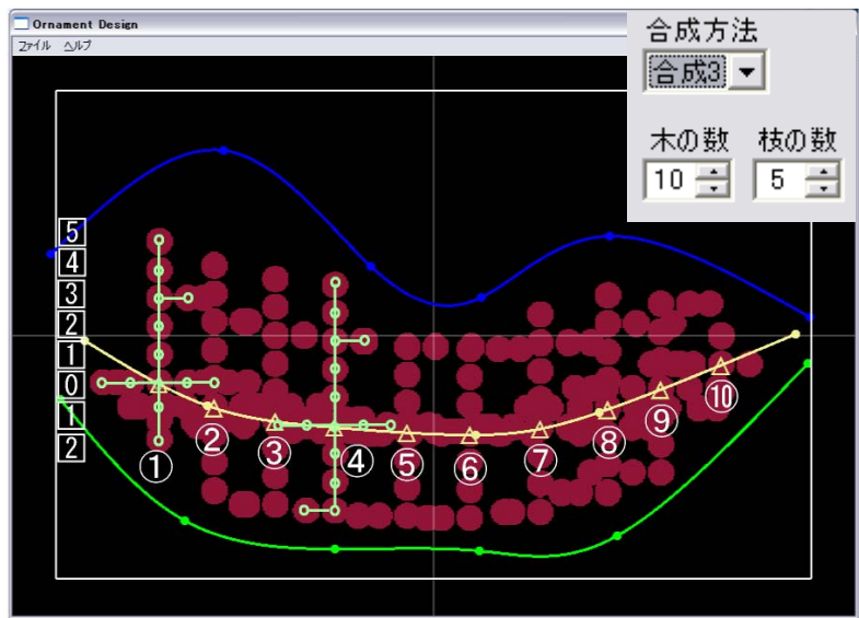
図 4.41 合成 3
