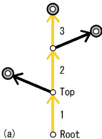
(a)世代数
