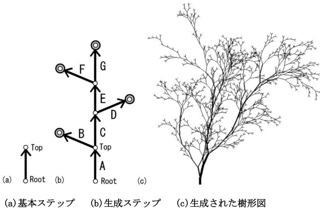
図 3.1 L-System
