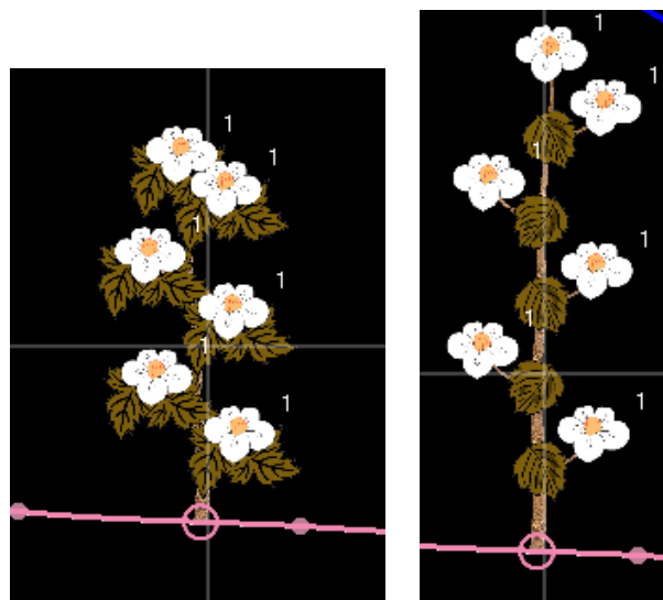
(a)葉 1
