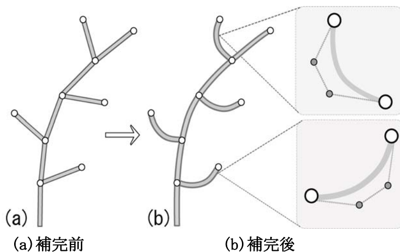
図 3.18 補完木
