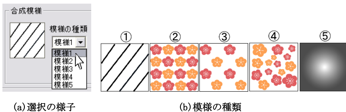
図 4.49 模様の選択
