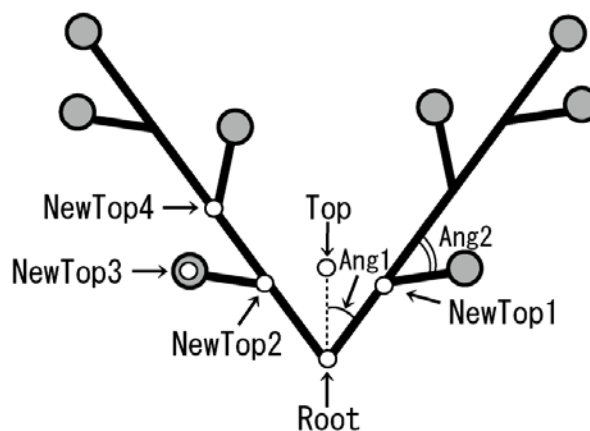
図 3.11 Tree7
