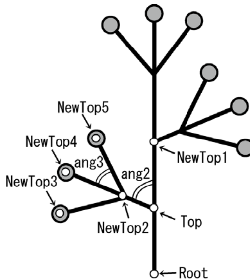
図 3.8 Tree4
