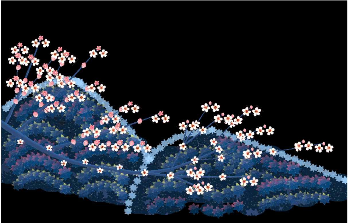
図 6.2 結果模様 2
