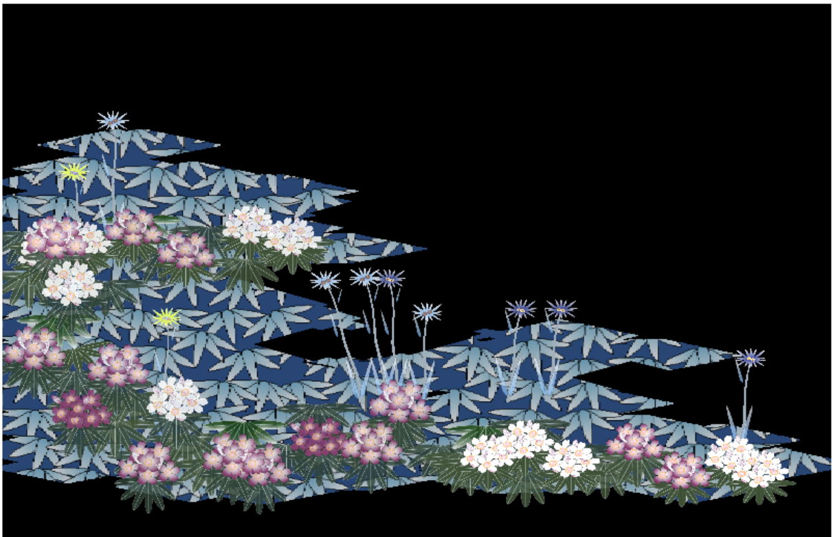
図 6.5 結果模様 5
