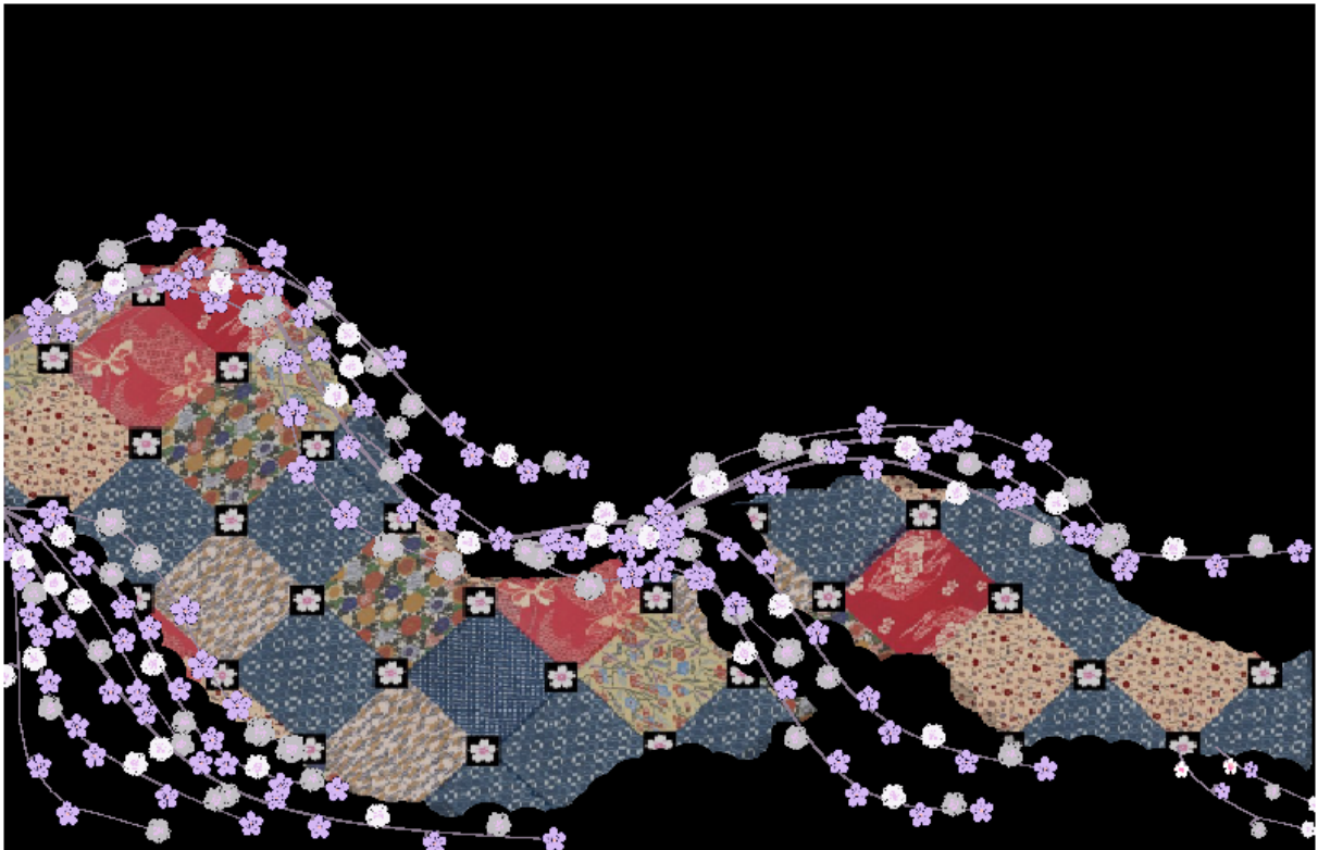
図 6.4 結果模様 4
