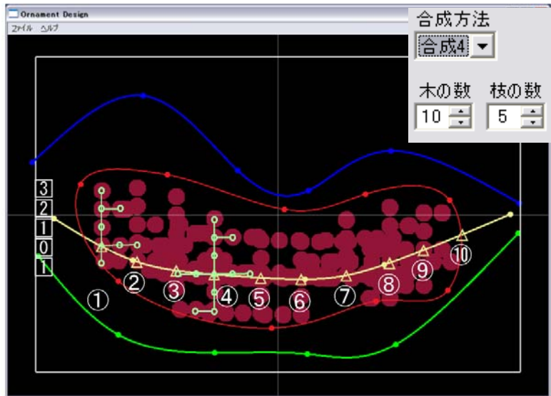
図 4.42 合成 4
