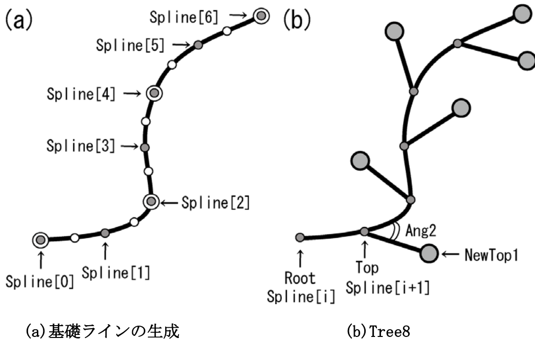
図 3.12 Tree8
