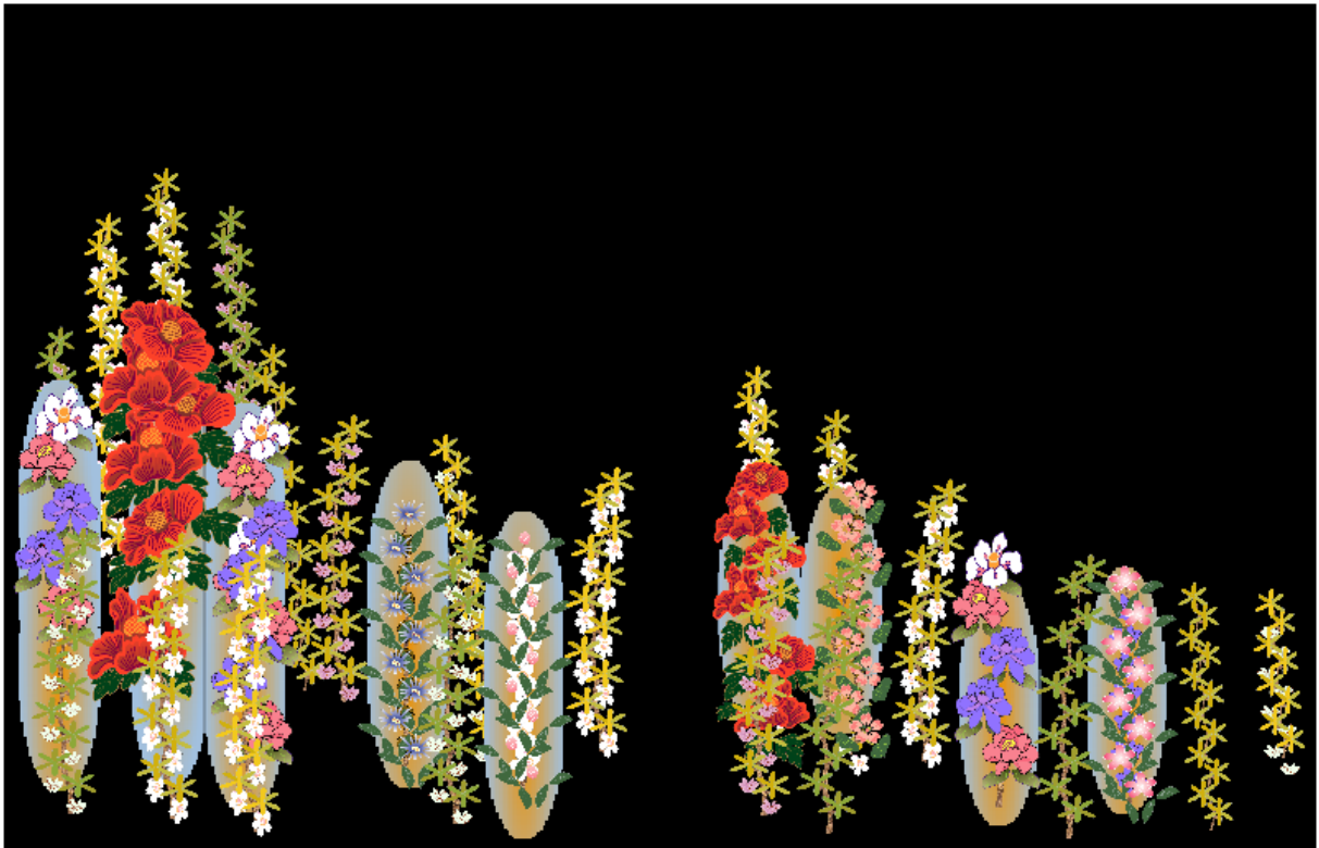
図 6.3 結果模様 3
