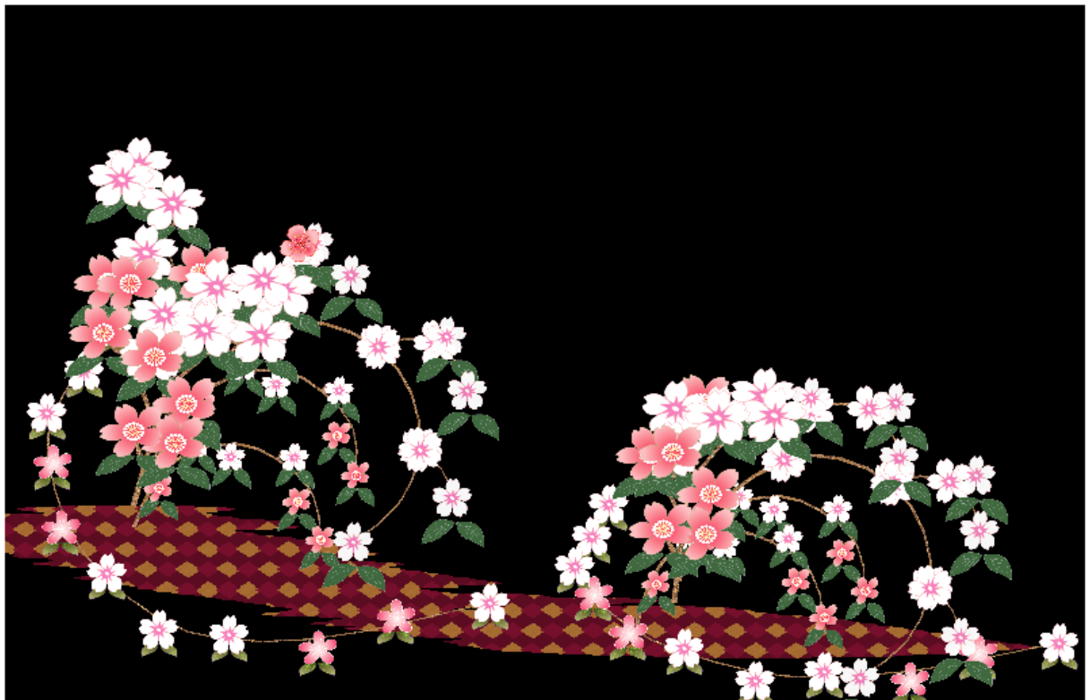
図 6.7 結果模様 7
