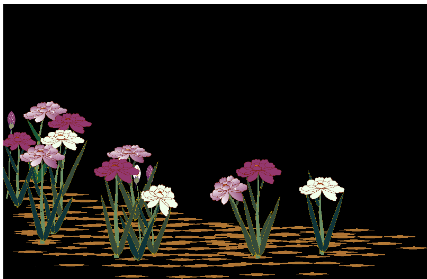
図 5.12 保存画像
