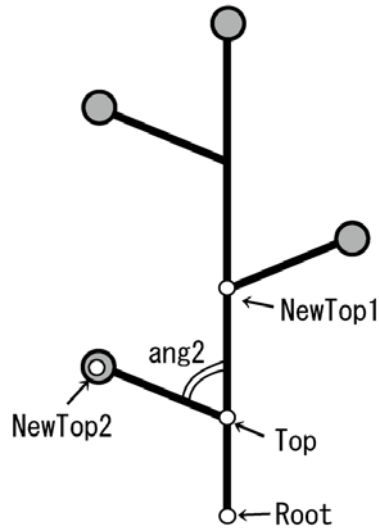
図 3.6 Tree2
