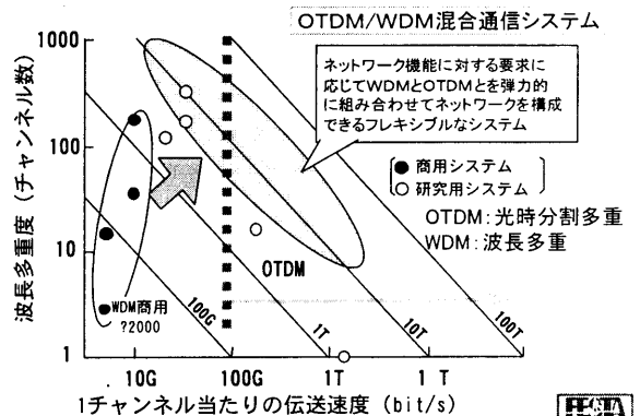
図1 将来の通信システム展望(FESTAの提案)
