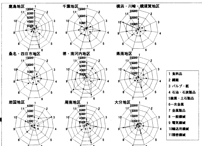
図7 コンビナートにおける技術フローマトリックス(化学産業のみ)
