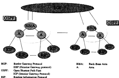
インターネット・ルーティング体系概念図
