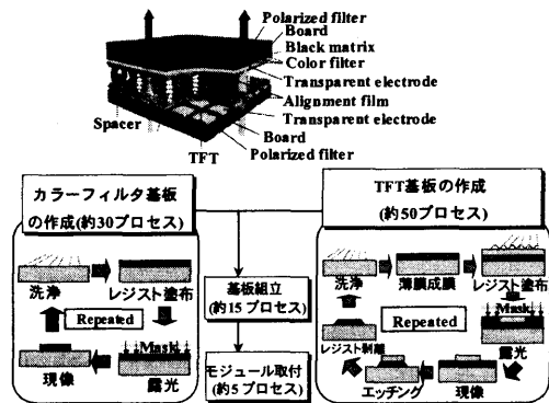
Fig. 4 液晶パネル構造と主要製造工程の概要
