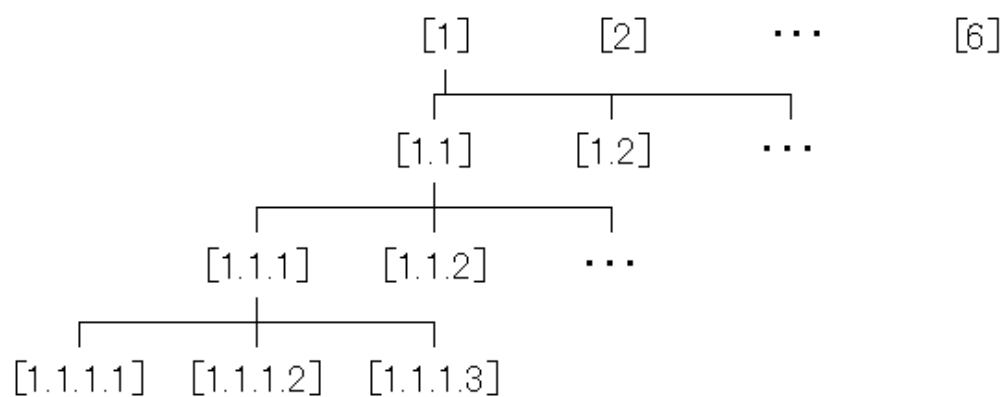
図 5.7: EC 番号の階層構造
