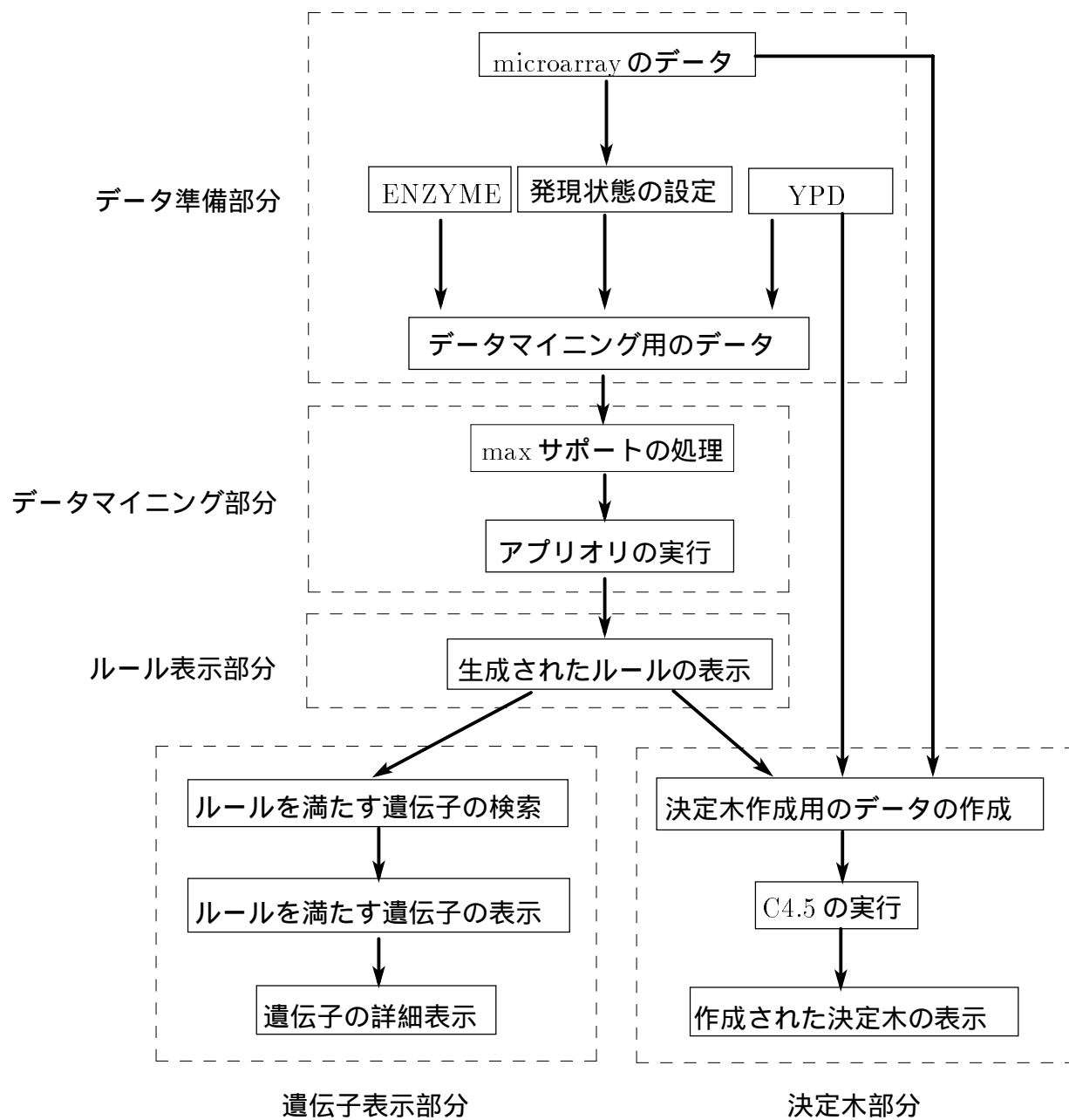
図 5.1: 本システムの概容
