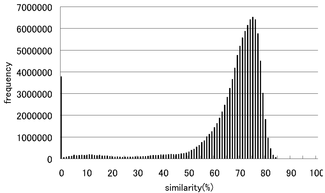
図 6.4: 全ルールの類似度
