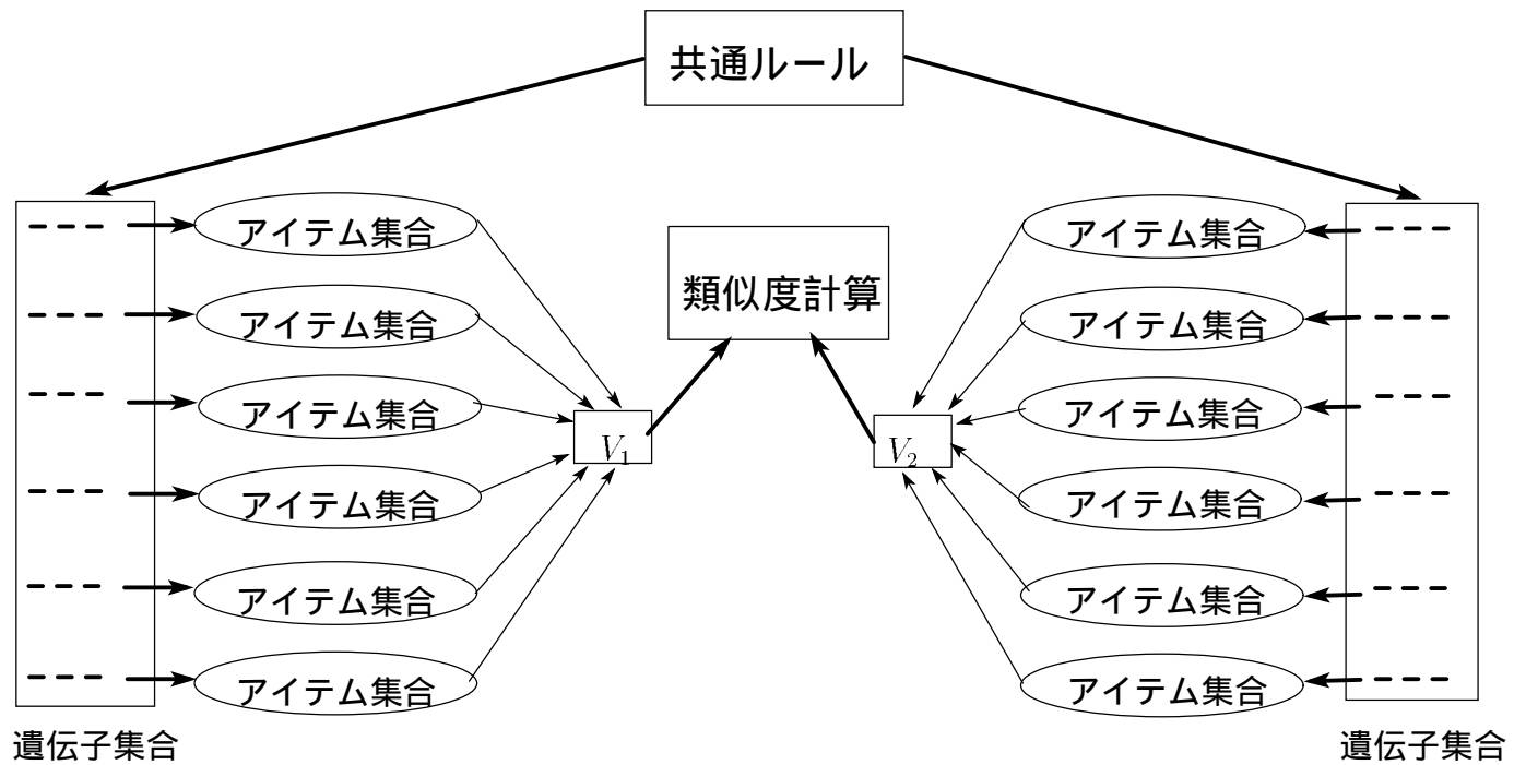
図 6.2: 類似度計算
