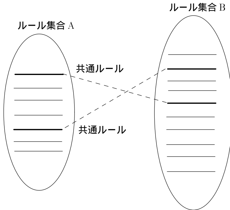
図 6.1: 共通ルール
