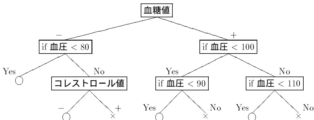
図 4.6: 決定木
