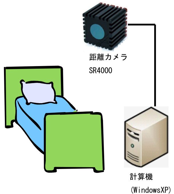
図 4 ベッド転落検知システムの機器構成
