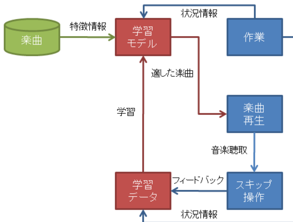
図 3.3 LISWO: 自動選曲アルゴリズム
