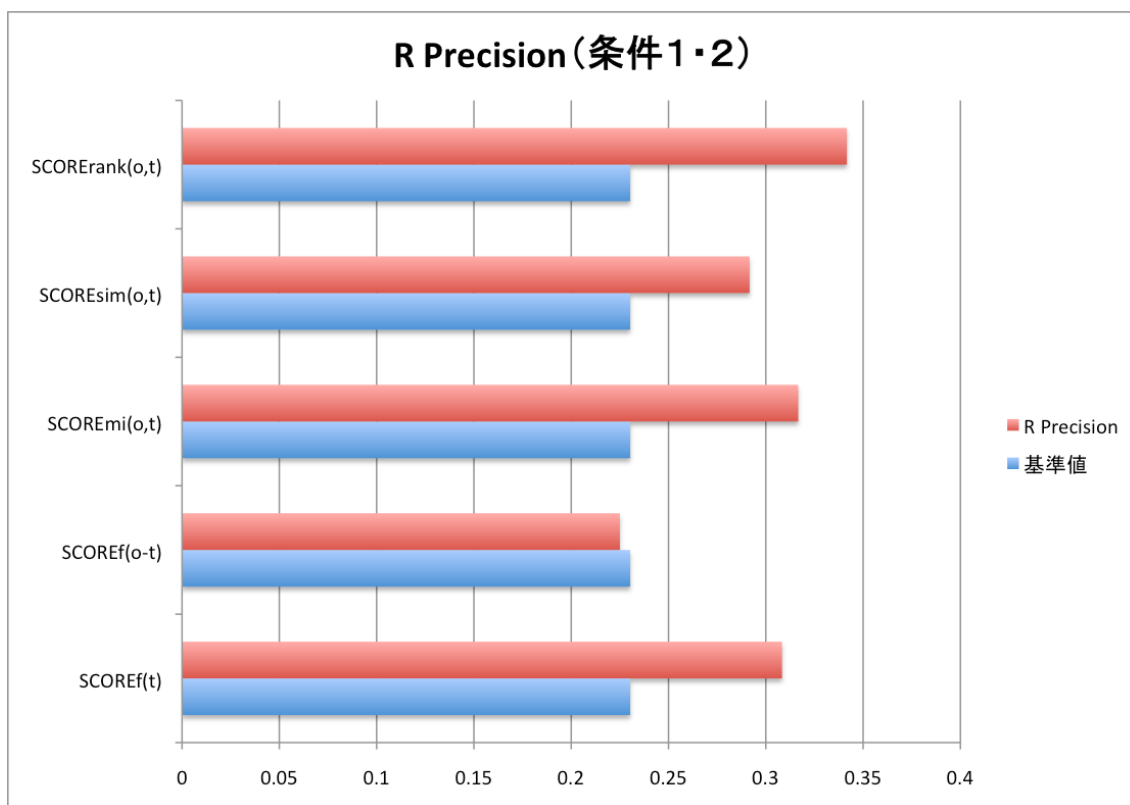
図 4.5: R Precision (条件1・2)
