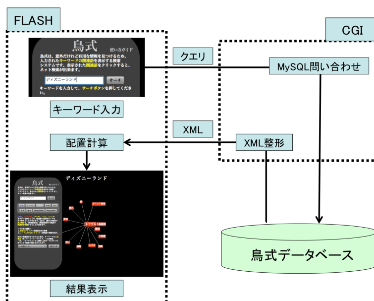
図 3.1: FLASH 版鳥式の動作概要
