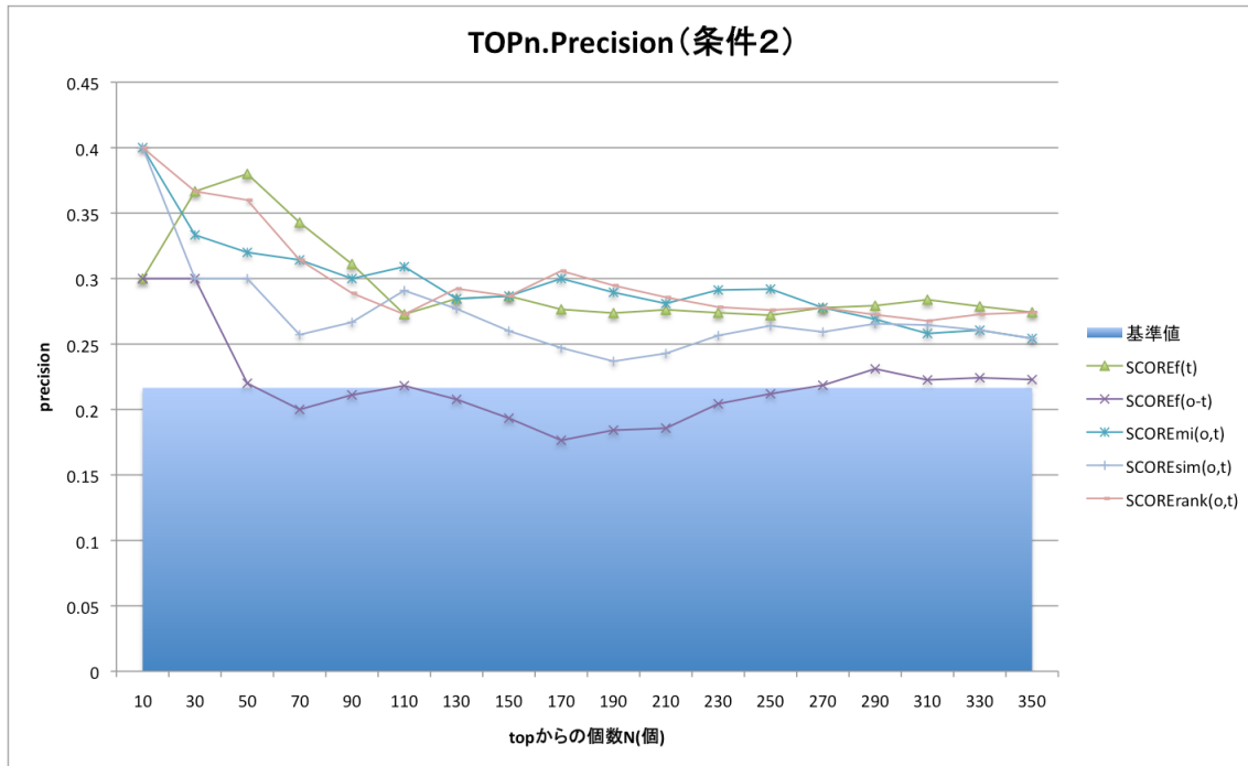
図 4.2: TOPn Precision (条件 2)
