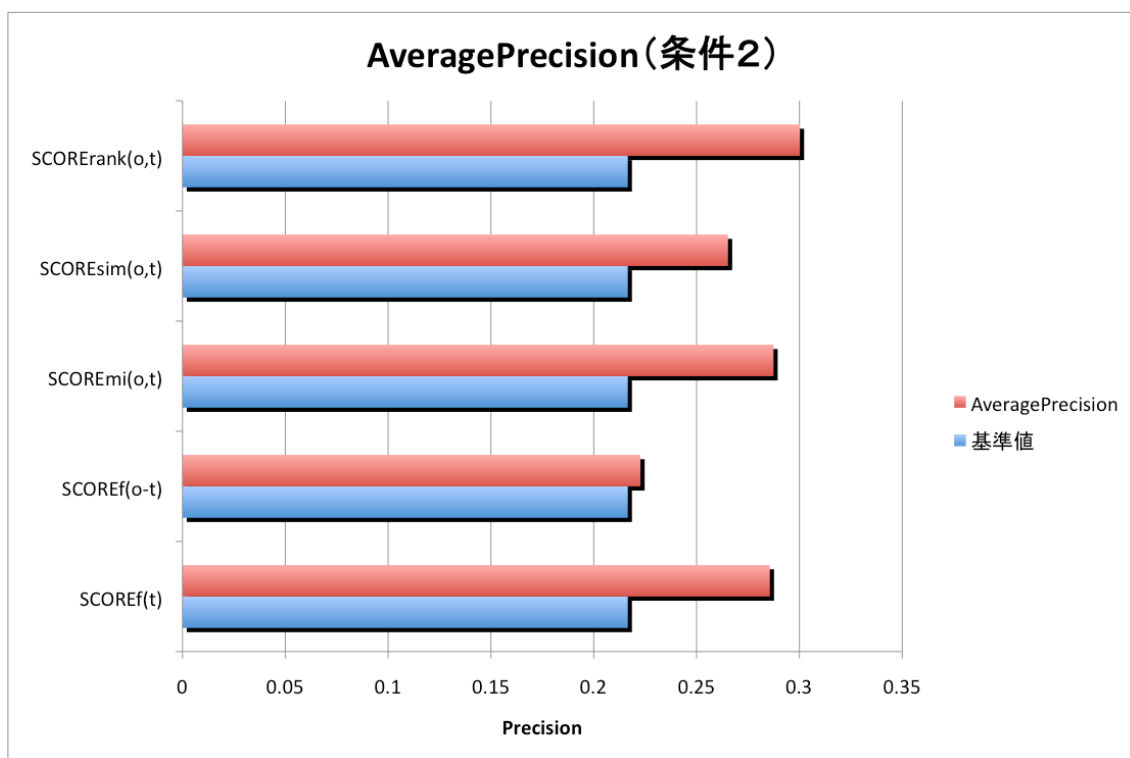
図 4.4: Average Precision (条件 2)
