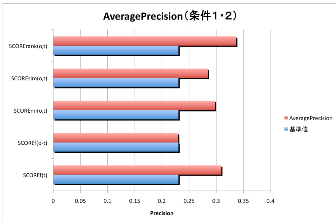
図 4.3: Average Precision (条件 1 ・ 2 )
