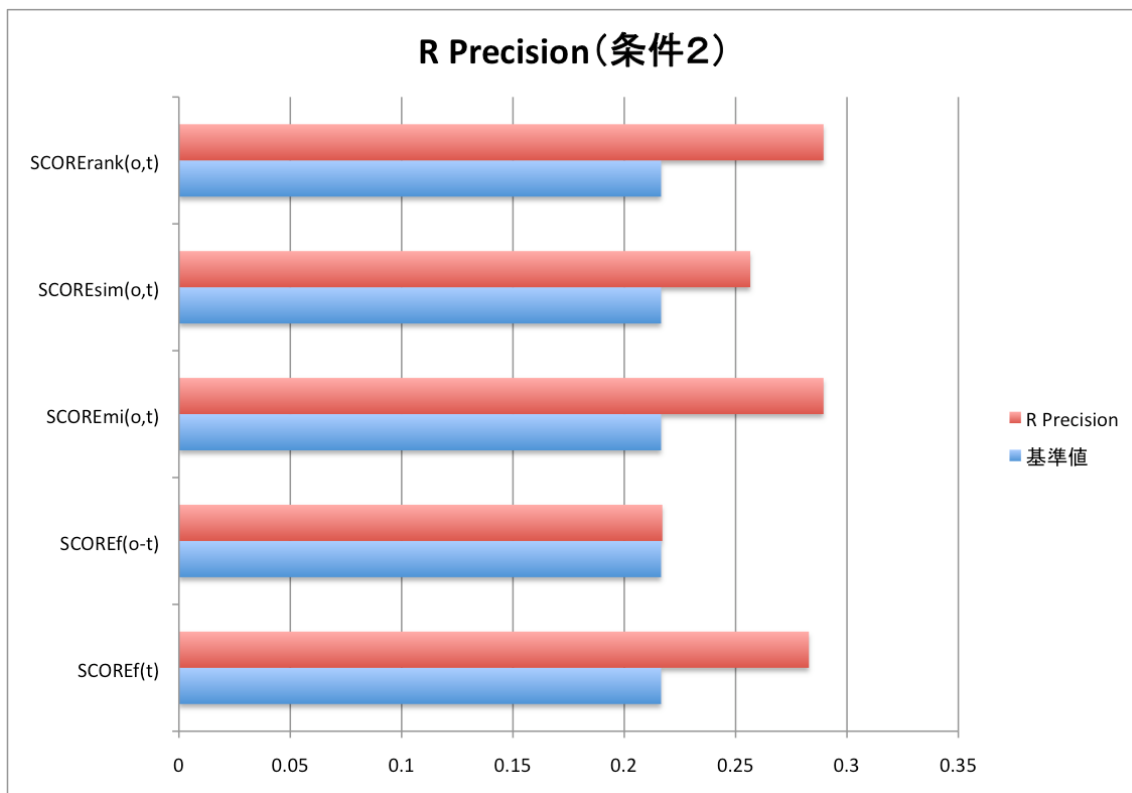
図 4.6: R Precision (条件 2)
