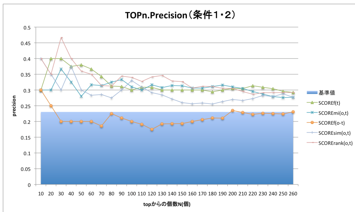
図 4.1: TOPn Precision (条件 1 ・ 2)
