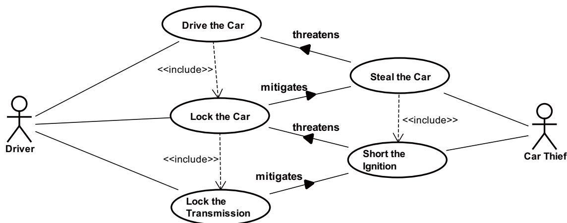
図 2.1: ミスユースケース図の例
