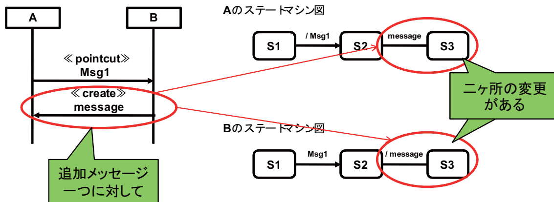
図 4.9: メッセージ追加によるステートマシン図への影響
