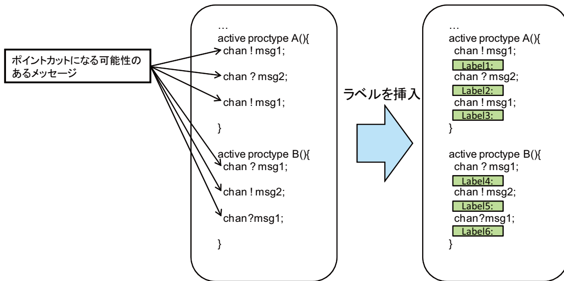
図 5.4: ポイントカットになる可能性のあるラベルの挿入
