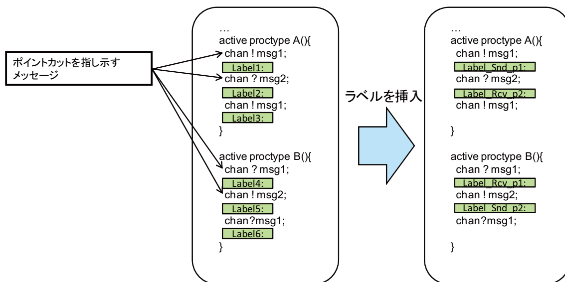
図 5.6: ポイントカットを指し示すラベルの挿入
