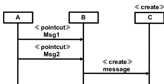
図 4.8: 追加ライフラインの指定
