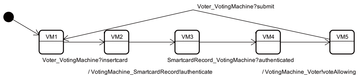
図 6.3: 例題の仕様 (VotingMachine)
