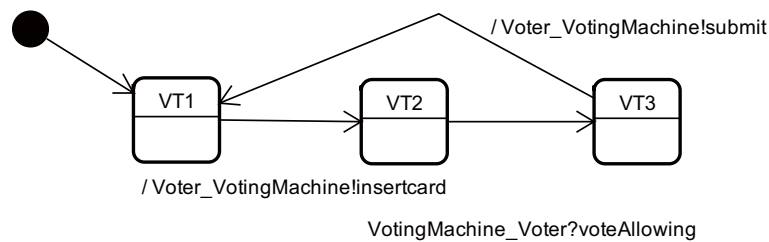
図 6.2: 例題の仕様 (Voter)
