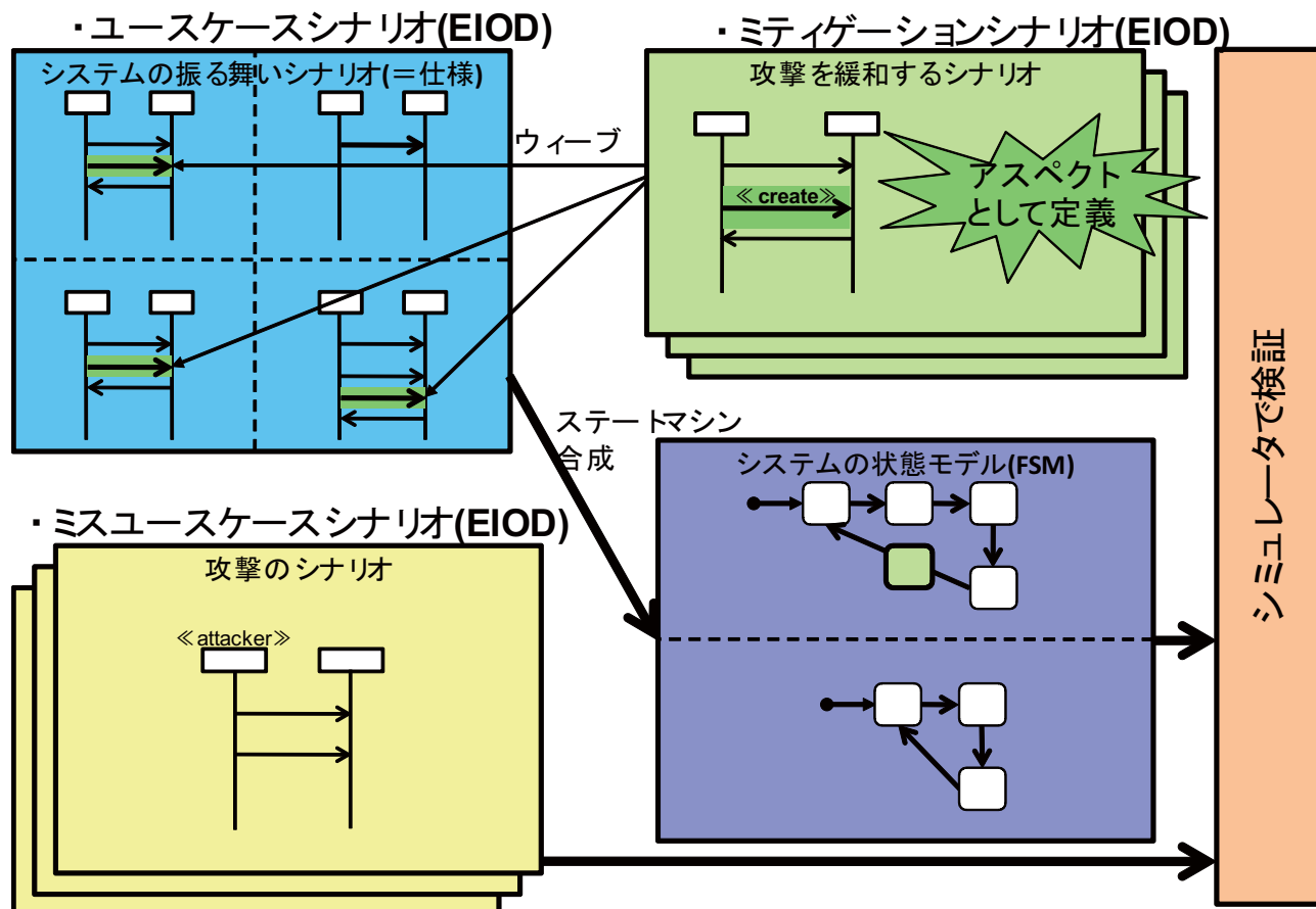
図 2.2: 関連論文の全体図
