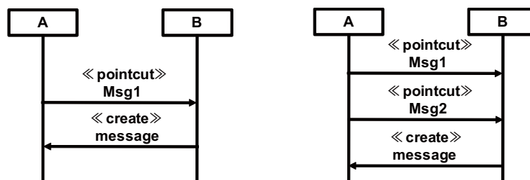
図 4.7: 追加メッセージの指定
