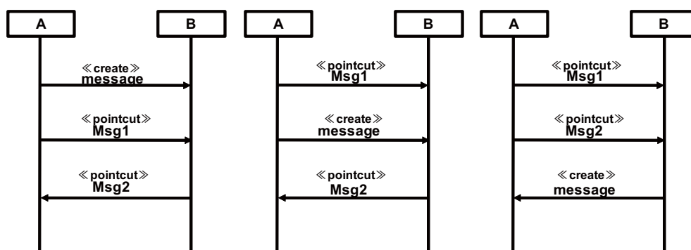
図 4.4: (any フラグメントなし) ミティゲーションモデルの例
