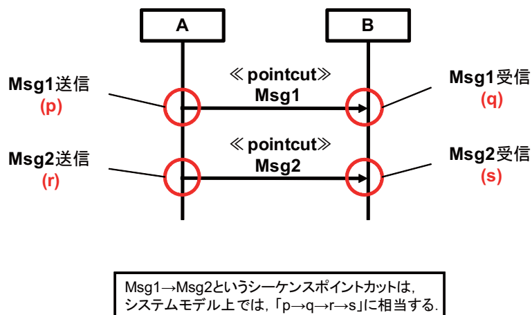
図 5.5: 検査対象のシーケンス
