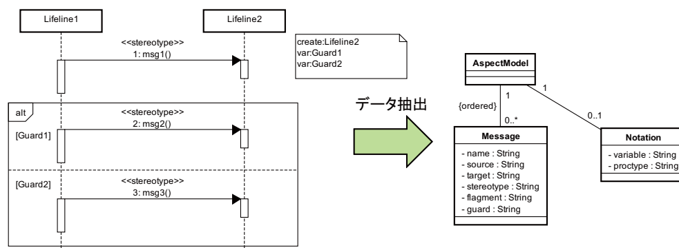
図 5.2: アスペクトモデルから抽出されたデータ構造
