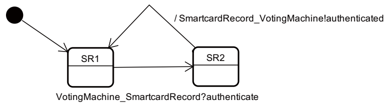
図 6.4: 例題の仕様 (SmartcardRecord)
