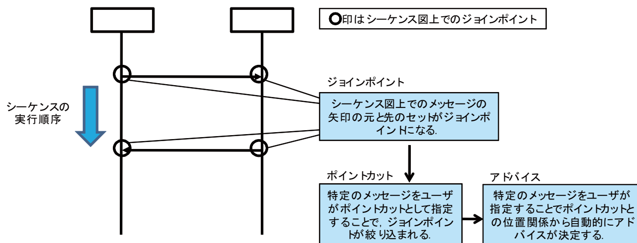
図 4.3: 提案手法のジョインポイントモデル
