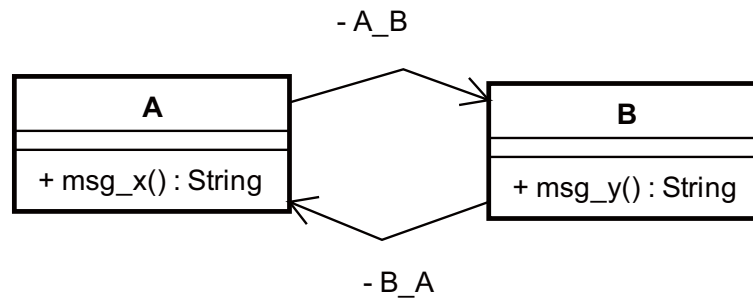
図 4.10: システムのクラス図
