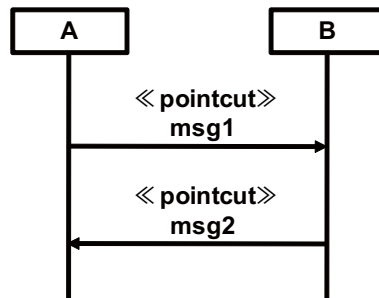
図 5.3: アスペクトモデル ( \text{msg1} \rightarrow \text{msg2} のポイントカットの指定時)
