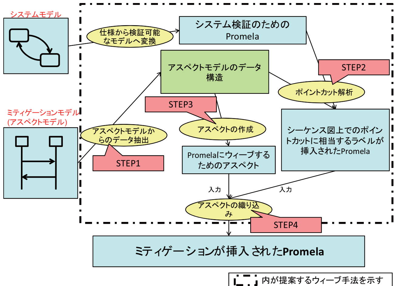
図 5.1: 提案するウィーブ手法の全体図
