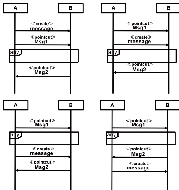
図 4.5: (any フラグメントあり) ミティゲーションモデルの例
