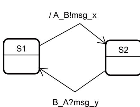
図 4.11: システムのステートマシン図 (A)
