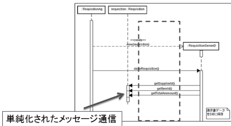
図 5.13: 階層の分離後のシーケンス図
