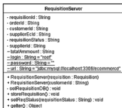
図 4.5: データベースアクセス
