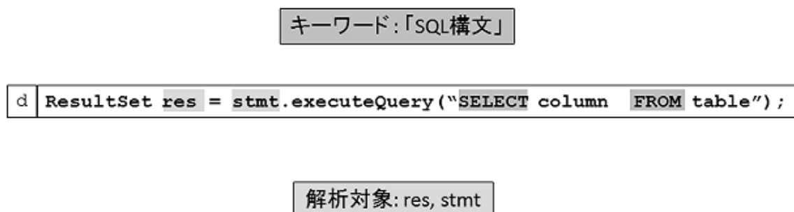
図 5.2: 特徴的な文字列を含む行の検出
