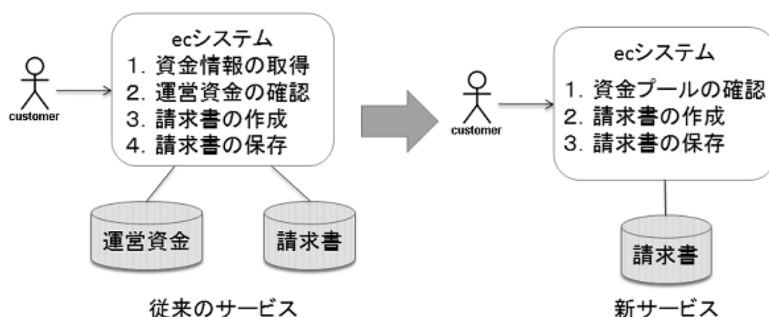
図 5.1: 新サービスの概要図
