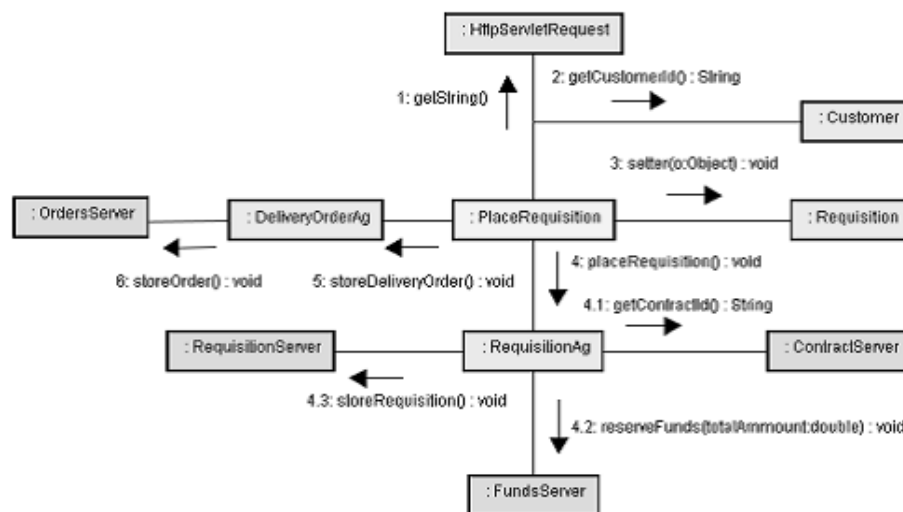
図 4.6: 商品の購入サービスのコミュニケーション図
