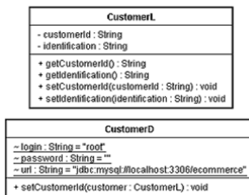
図 5.11: 階層の分離後のクラス図
