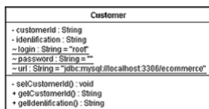
図 5.10: 再構成前のクラス図
