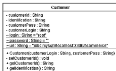
図 4.4: エンティティクラス
