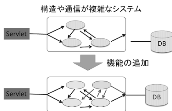
図 2.1: レガシーシステムの構成
