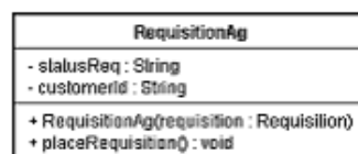
図 4.3: ビジネスロジッククラス
