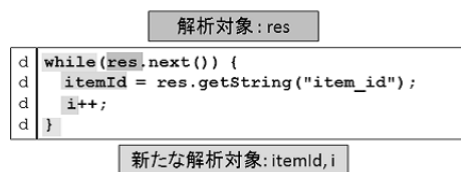
図 4.9: 制御ブロックに含まれる変数のフロー解析例
