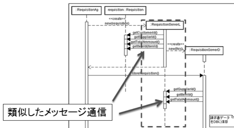
図 5.12: 階層の分離後のシーケンス図
