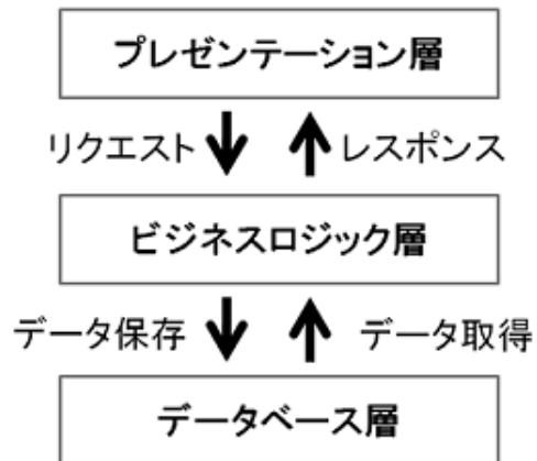
図 3.1: 3 階層アーキテクチャの構成
