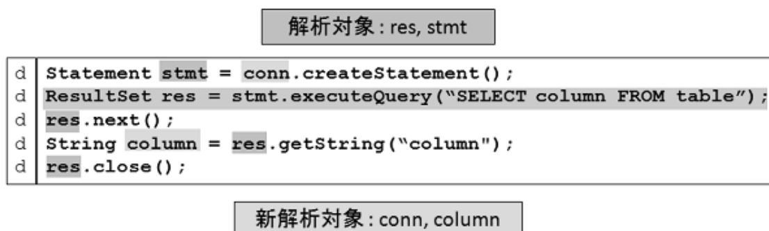
図 5.3: 代入文の右辺に出現する変数 res, stmt を始点とするフロー解析
