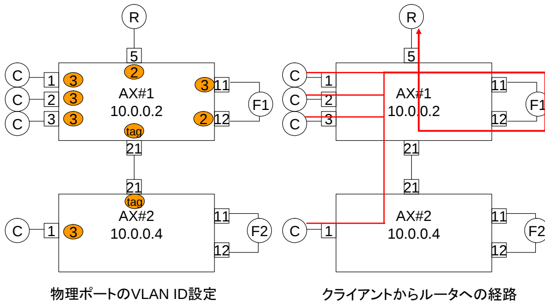
図 6.3: 通信ログ監視機能を提供するトポロジー
