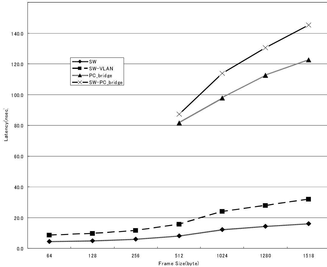
図 6.12: レイテンシー測定値のグラフ
