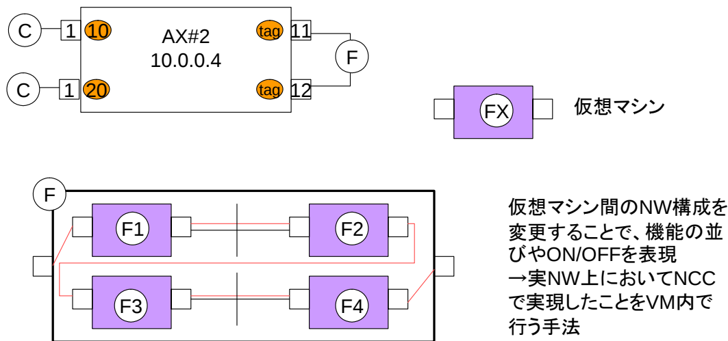
図 7.3: FunctionBox の VM 化
