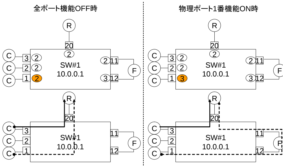
図 5.2: GUI アプリケーションによる機能の選択制御と構築される論理トポロジー
