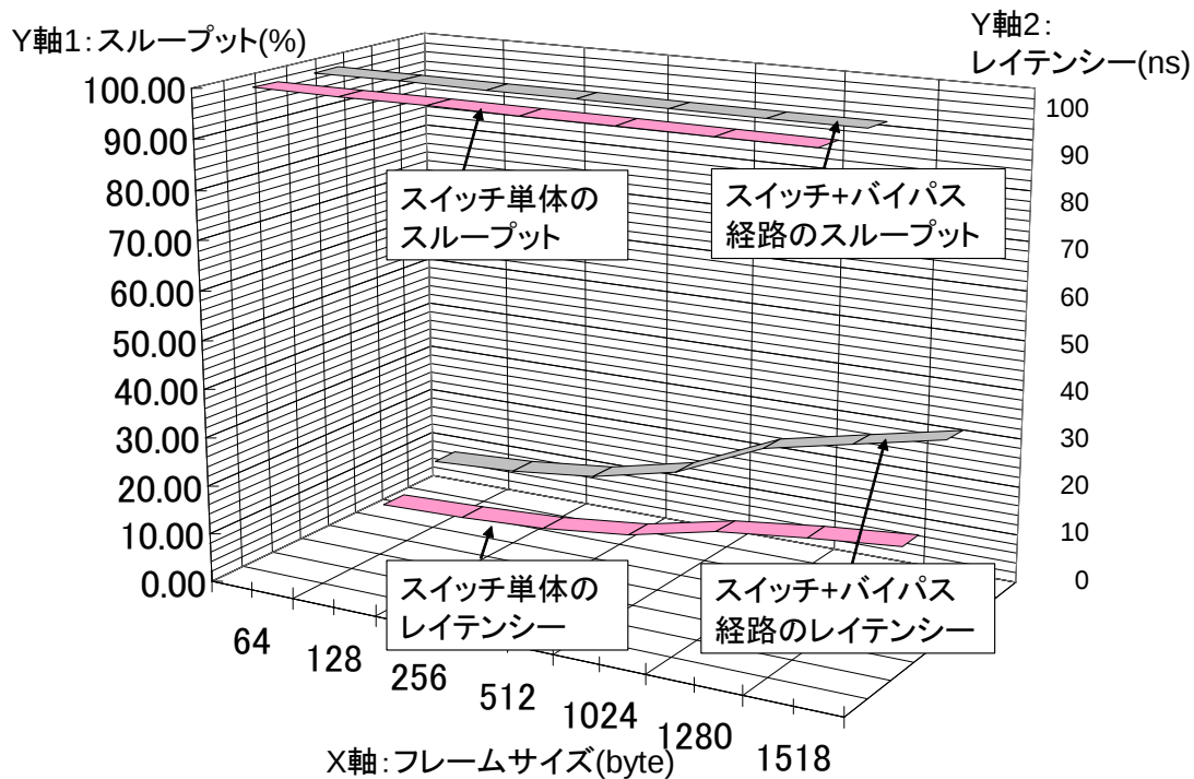
図 6.14: スイッチ単体、およびバイパス経路構成の比較
