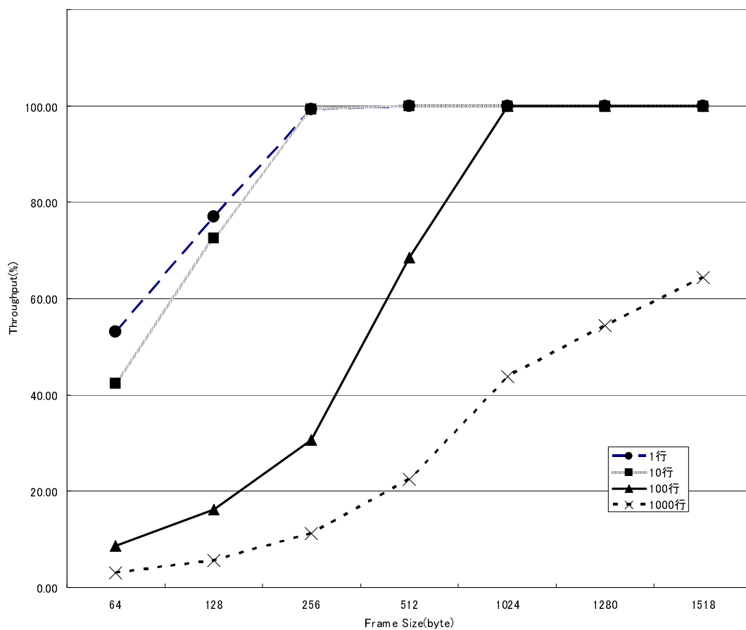
図 6.9: フィルタ設定数ごとのスループット測定値のグラフ
