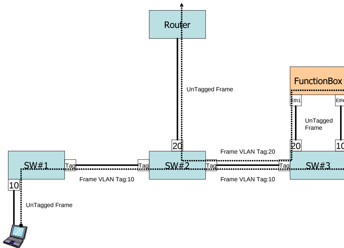
図 4.9: TagVLAN による通信経路の構築
