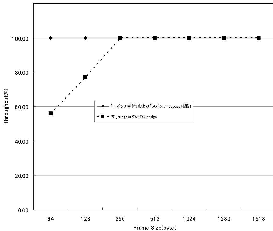
図 6.8: スループット測定値のグラフ
