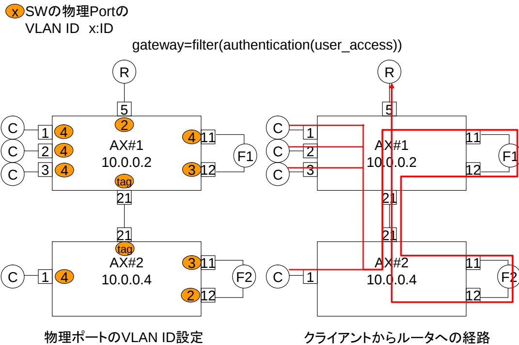
図 5.13: NCC により構築される論理ネットワーク図
