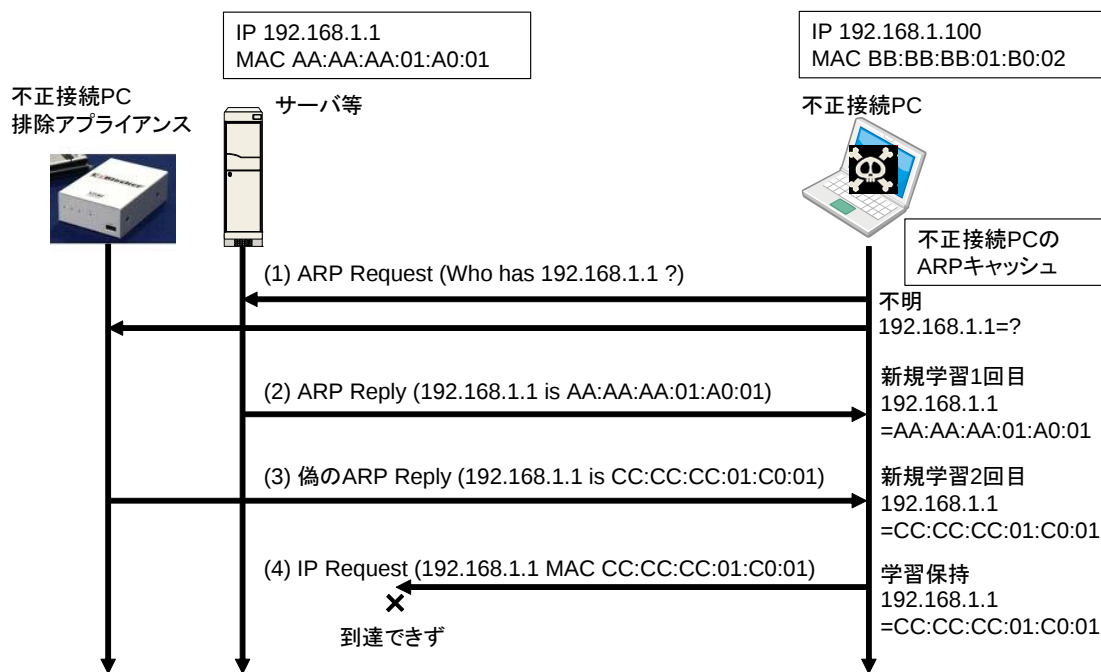
図 3.2: 不正接続 PC 排除システムによる不正接続 PC 排除の様子
