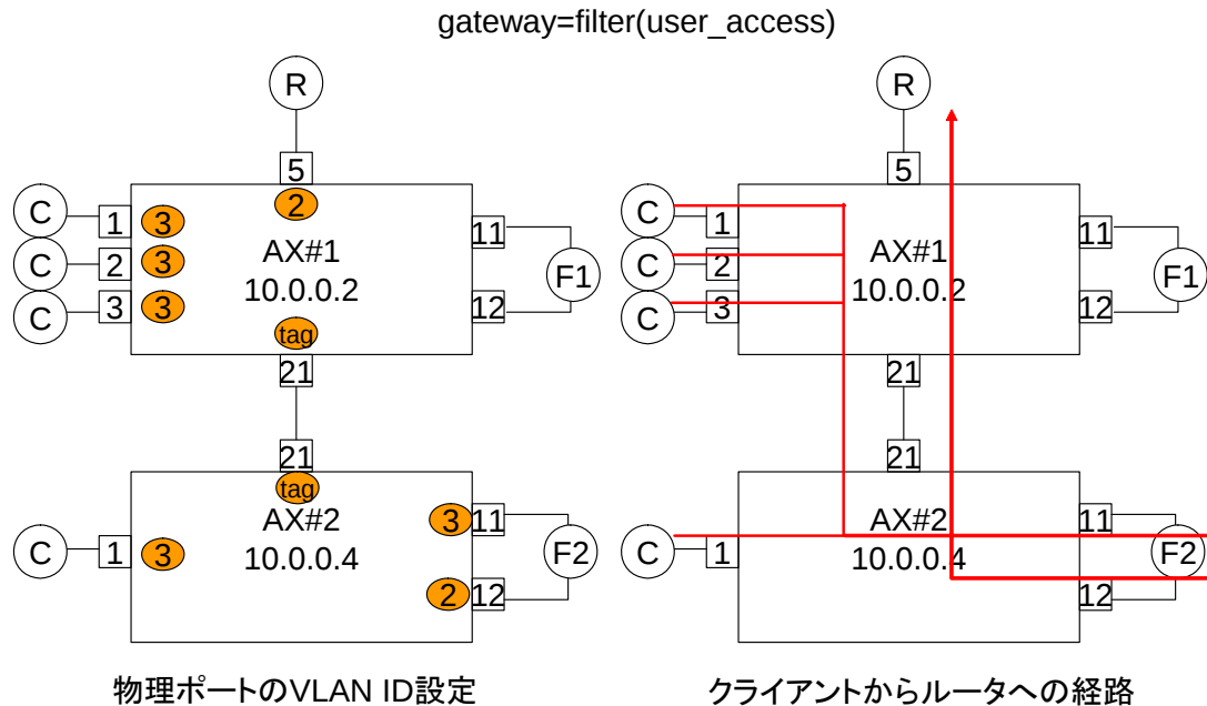
図 6.2: フィルタ機能を提供する論理トポロジー
