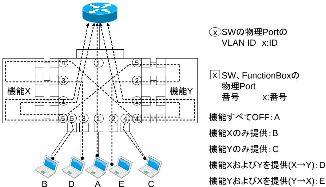
図 5.6: インタフェース増設によるパスの拡張
