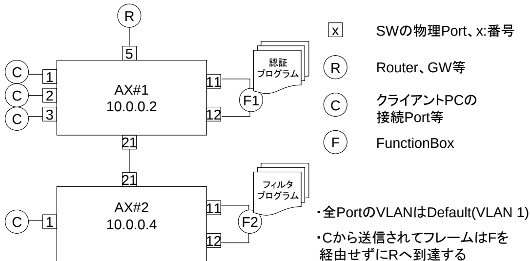
図 5.12: 例に用いる物理ネットワーク構成図
