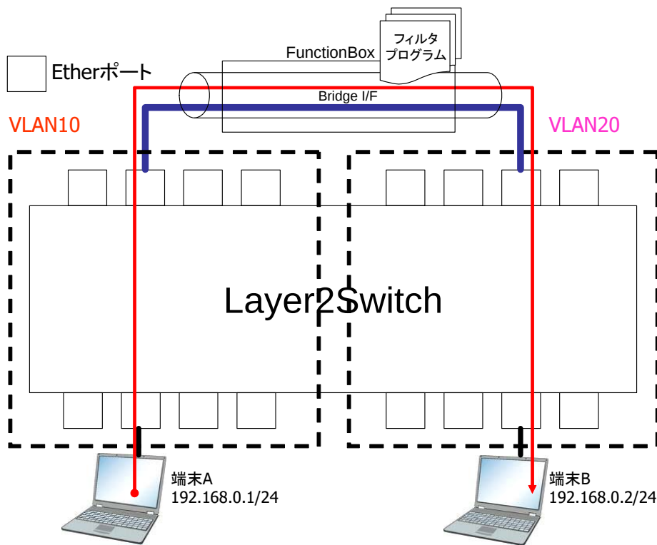
図 4.8: 既設レイヤ 2 スイッチへのフィルタリング機能の追加
