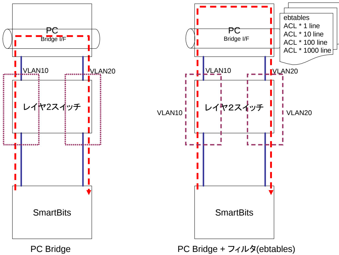
図 6.11: レイテンシー測定対象トポロジー 2
