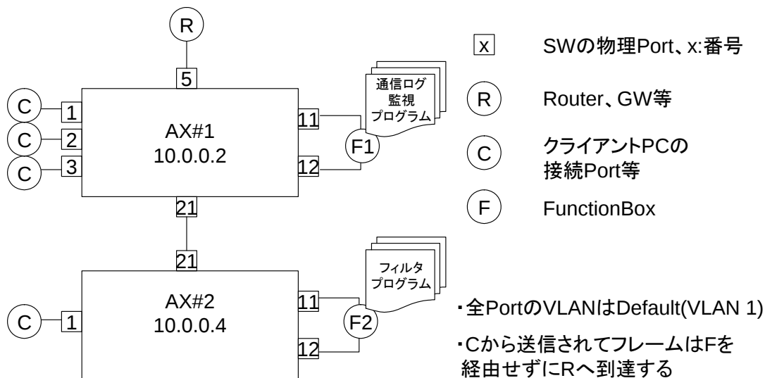
図 6.1: 実験に用いる物理ネットワーク
