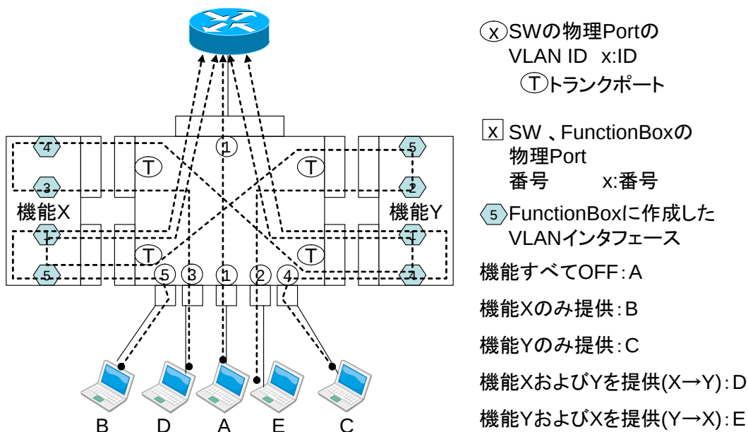
図 5.7: VLAN インタフェースによるパスの拡張
