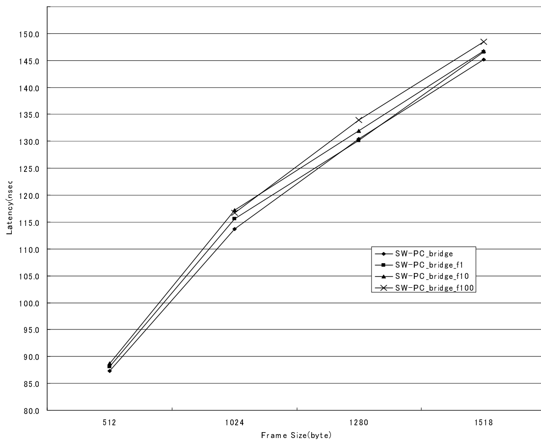
図 6.13: フィルタ設定数ごとのレイテンシー測定値のグラフ
