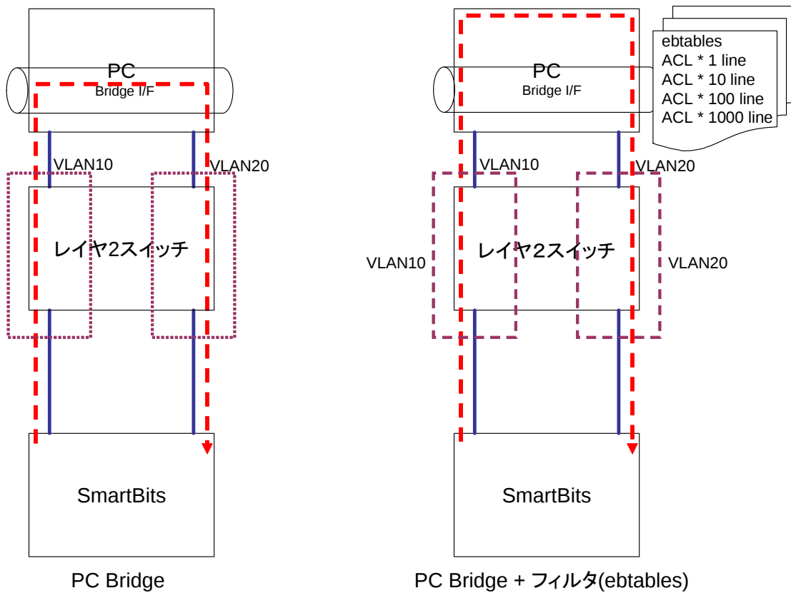
図 6.7: スループット測定対象トポロジー 2
