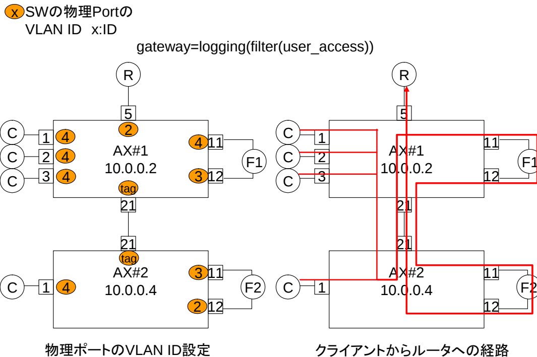
図 6.4: 通信ログ監視、フィルタの順で機能を提供する論理トポロジ
