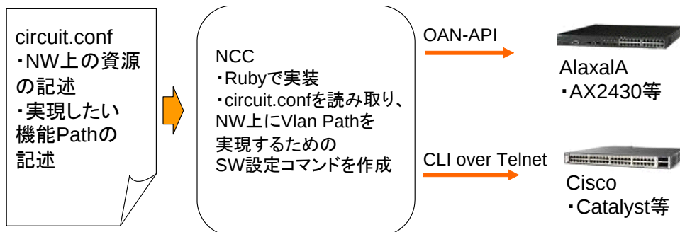
図 5.10: NCC の動作概要
