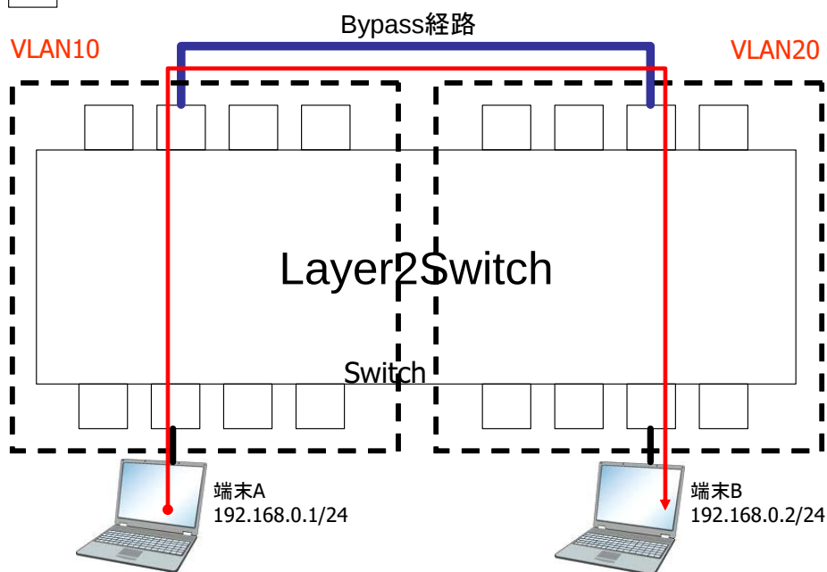
図 4.6: VLAN 間を接続する bypass 経路を経由する通信
