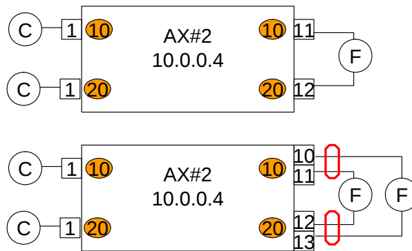
図 7.2: Link-Aggregation によるスループットの改善
