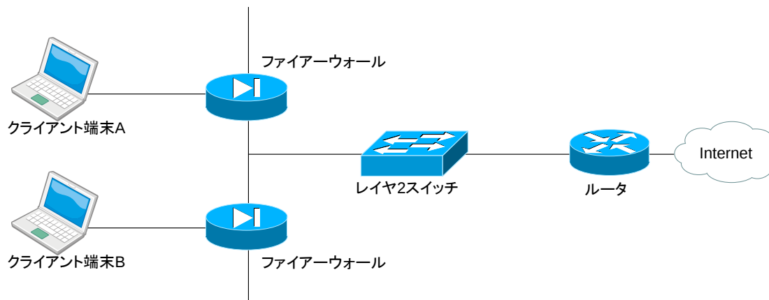
図 4.2: MiddleBox の分散配置
