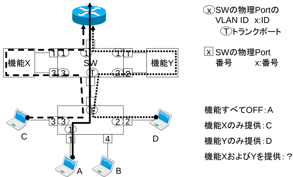
図 5.4: 機能を提供するトポロジー 1
