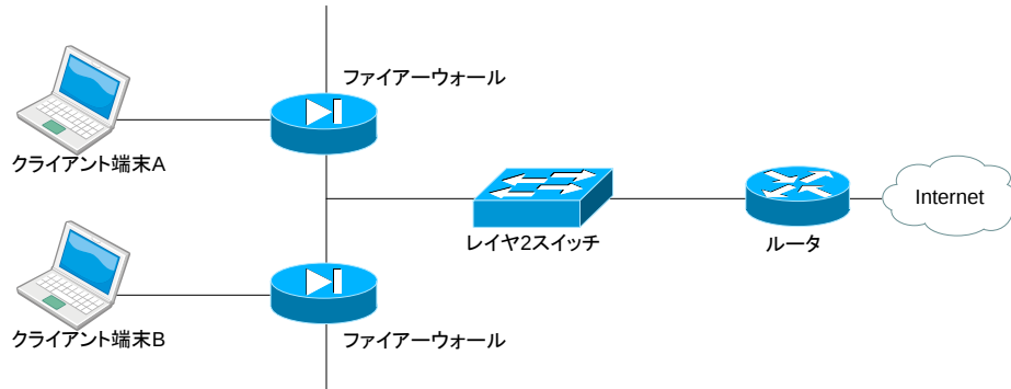
図 7.7: MiddleBox の分散配置
