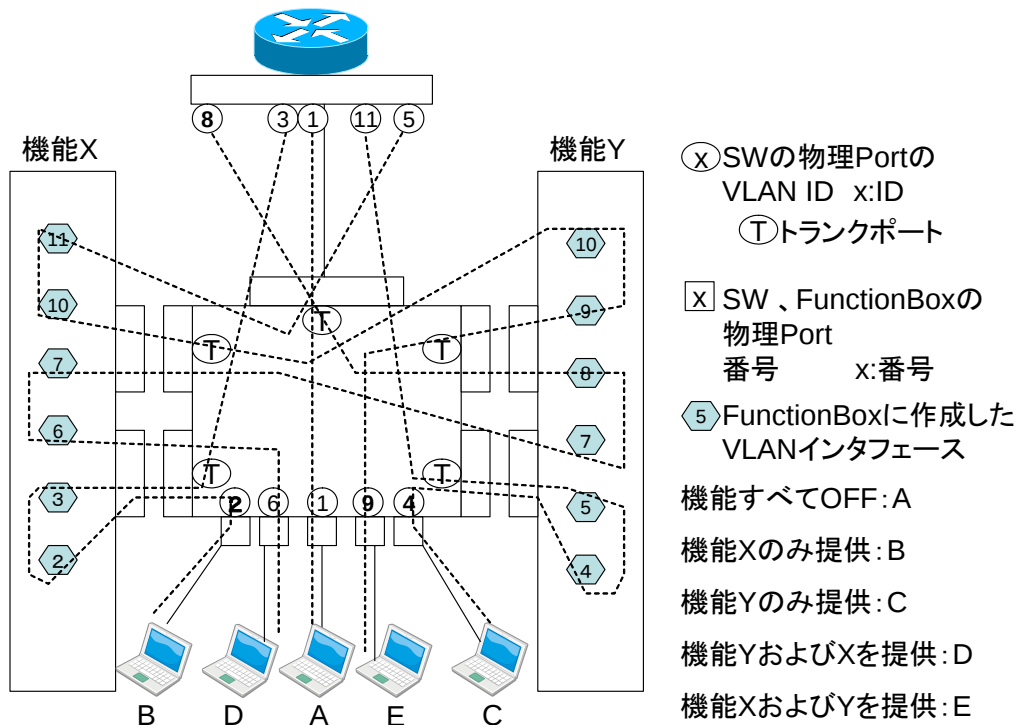
図 5.8: セグメントを分けるパス構築
