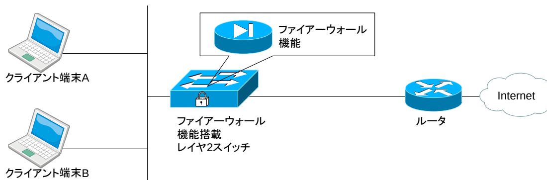
図 4.1: 高機能スイッチの導入
