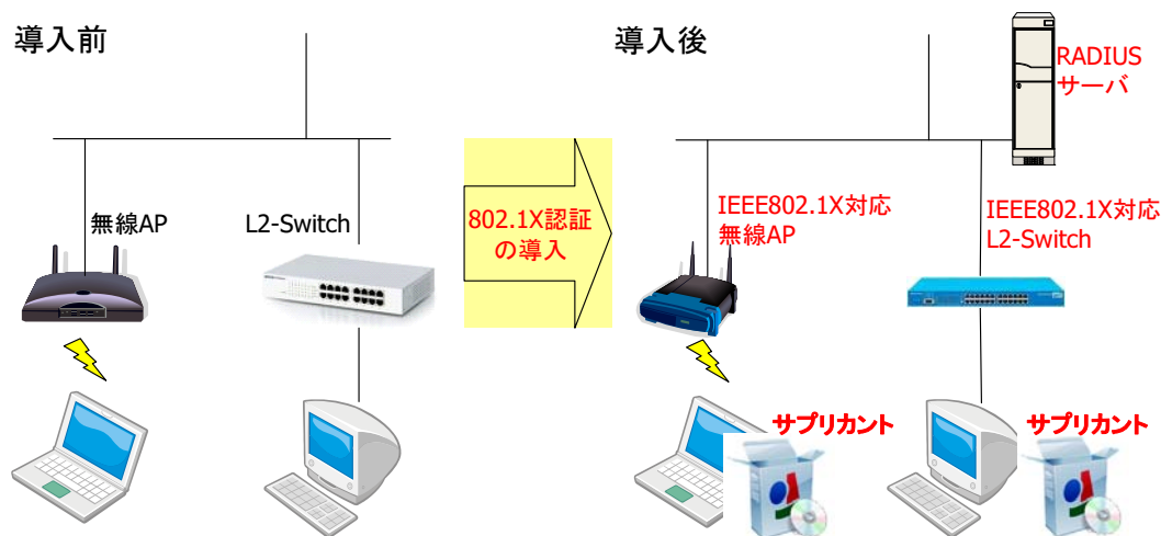
図 2.1: IEEE802.1X 機能導入のための既設機器のリプレイス
