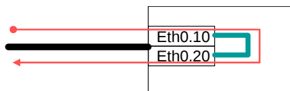
図 7.1: 1port-bridge による使用物理ポートの節約
