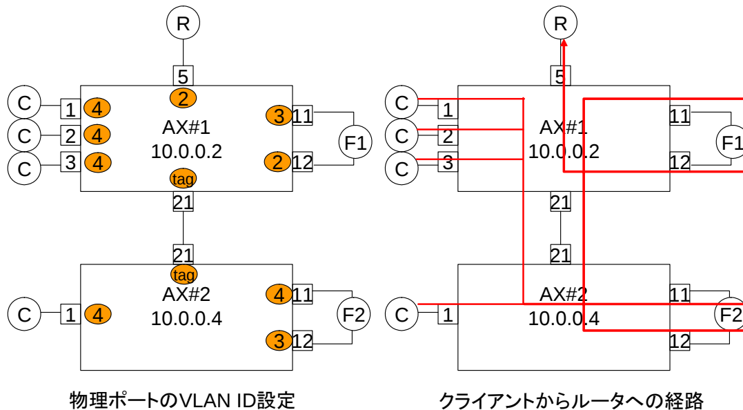
図 6.5: フィルタ、通信ログ監視の順で機能を提供する論理トポロジー
