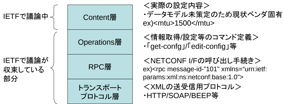
図 5.1: NETCONF のレイヤ構造
