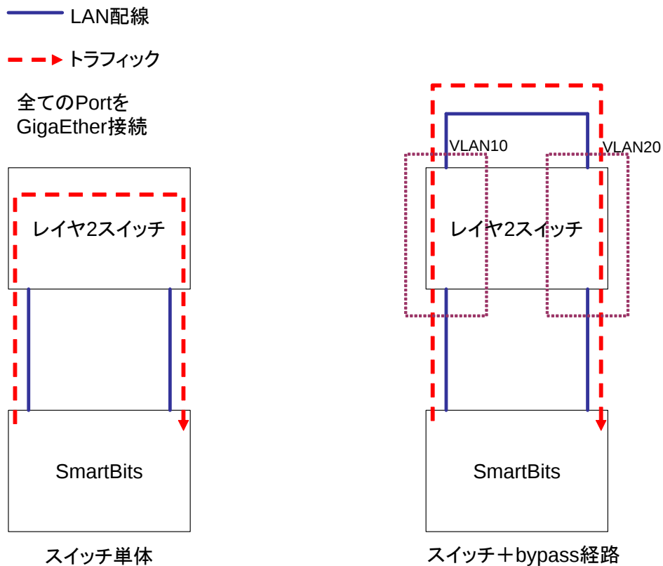
図 6.6: スループット測定対象トポロジー 1
