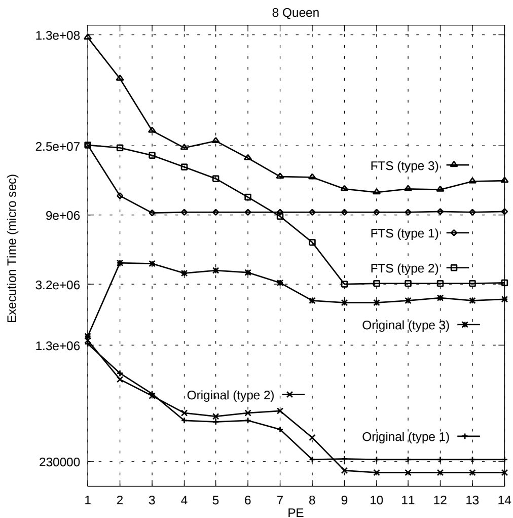
図 10.15: 8 Queen プログラム ( 並列実行における処理性能変化 )
