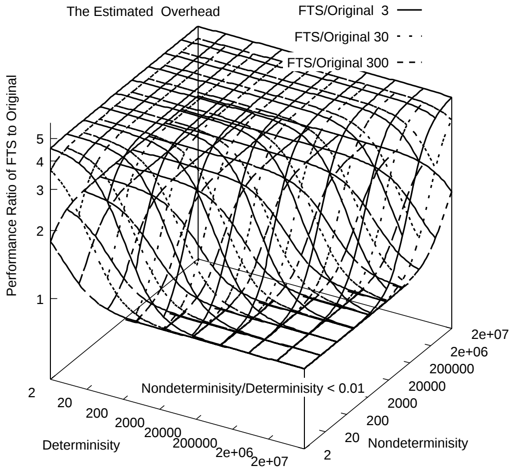
図 9.1: 単一プロセッサでの非決定性/決定性に対する推定オーバーヘッド
