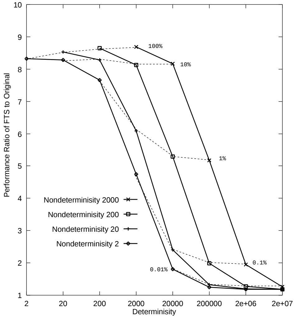
図 10.8: ベンチマークプログラム (非決定性/決定性比による処理性能変化)
