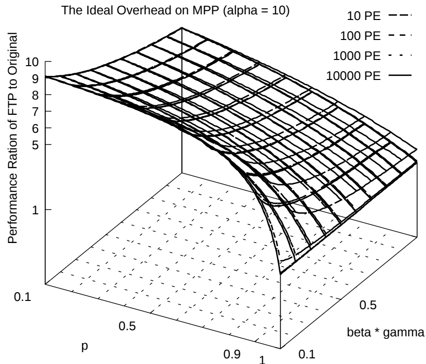
図 9.4: マルチプロセッサでの推定オーバーヘッド ( 0.1 < p < 1 )
