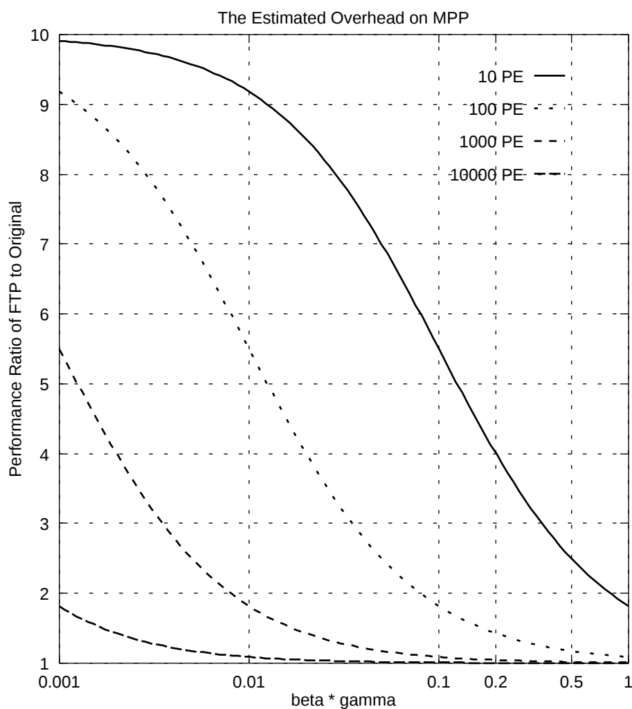
図 9.3: マルチプロセッサでの推定オーバーヘッド ( p = 1 )
