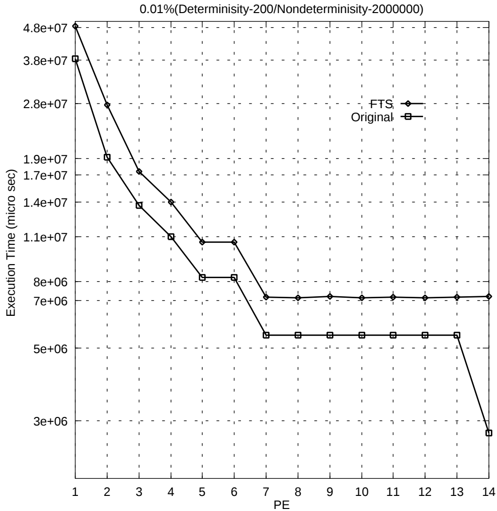
図 10.13: ベンチマークプログラム ( 並列実行における処理性能変化 2 (1) )
