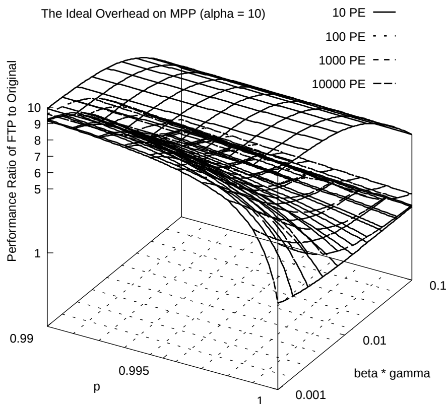
図 9.5: マルチプロセッサでの推定オーバーヘッド ( 0.99 < p < 1 )
