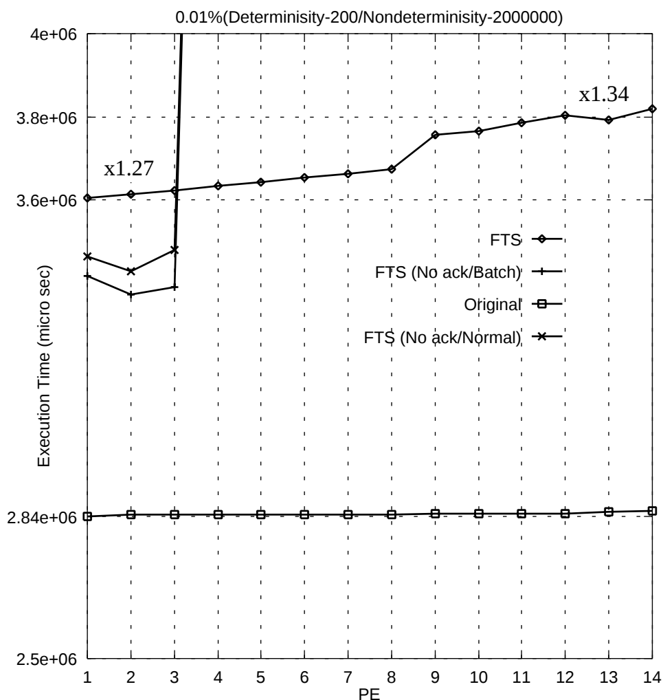
図 10.10: ベンチマークプログラム ( 並列実行における処理性能変化 1 )
