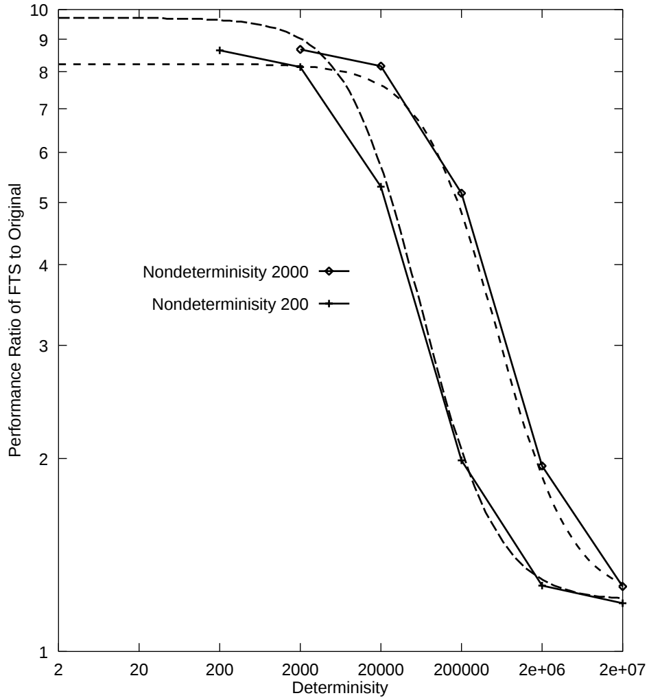
図 10.9: ベンチマークプログラム (見積りオーバーヘッドとの比較)
