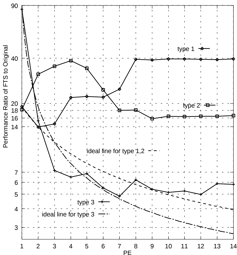
図 10.17: 8 Queen プログラム ( 並列実行における処理時間比 )
