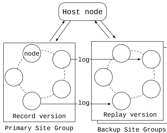
図 7.1: 耐故障並列ソフトウェアの動的構成
