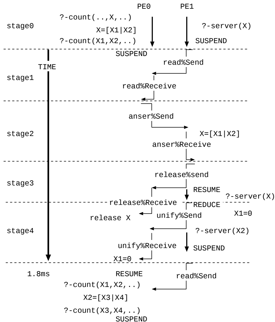
図 10.6: 基礎データの測定 ( コミュニケーション )
