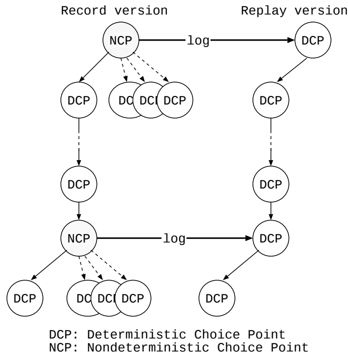
図 6.1: Instant Replay 実行の概念
