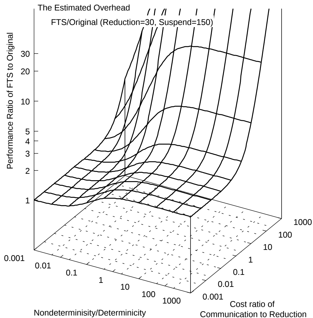
図 9.2: 単一プロセッサでの通信コストを考慮した推定オーバーヘッド
