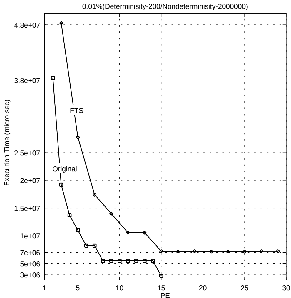
図 10.14: ベンチマークプログラム ( 並列実行における処理性能変化 2 (2) )
