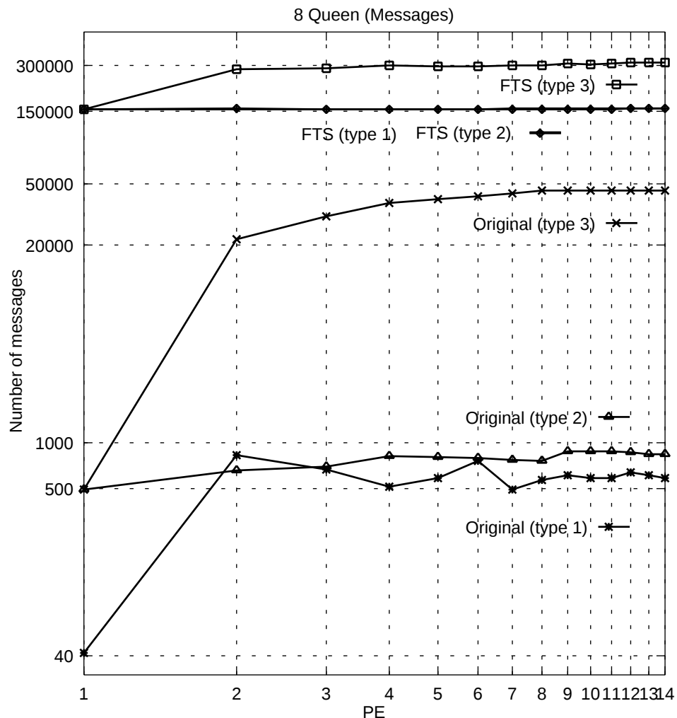
図 10.16: 8 Queen プログラム ( 並列実行におけるメッセージ数 )
