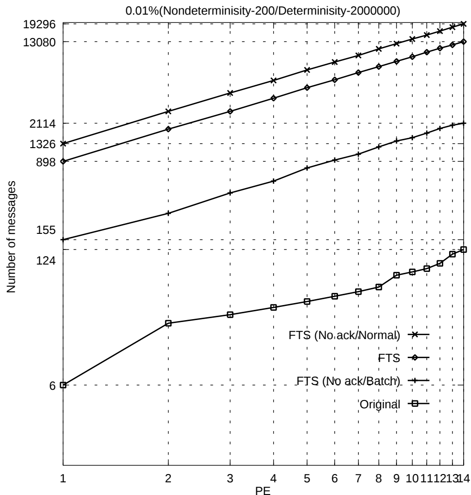
図 10.11: ベンチマークプログラム ( 並列実行時のシステム総メッセージ数 )
