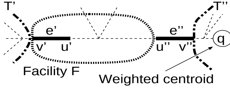
図 5.6: 木 T の重心 q を含まない設備 F と長さ \epsilon の部分辺 e' , e''
