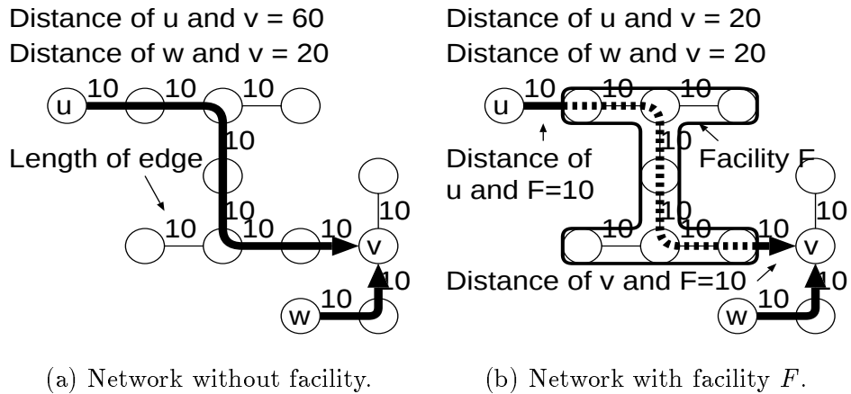
図 5.1: 設備配置と全対距離和
