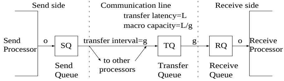
図 2.3: LogPQ モデルの構造
