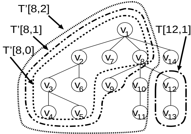
図 5.13: 部分木 T[j, t] と T'[j, t]
