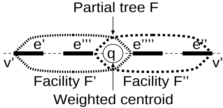
図 5.7: 木 T の重心 q を含む，最適な連続木形状設備 F' と距離和最小の連続木形状設備 F''
