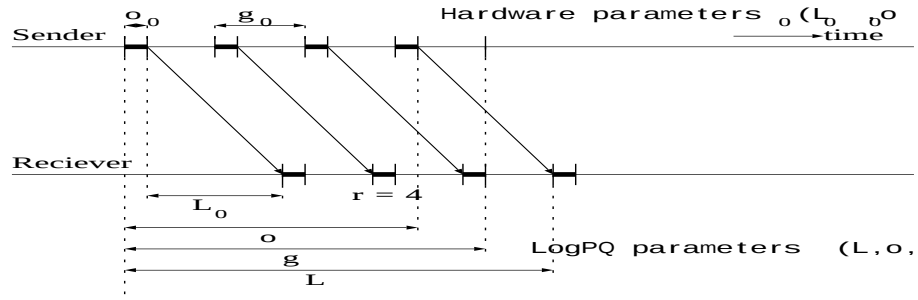
図 2.4: LogPQ モデルの通信動作
