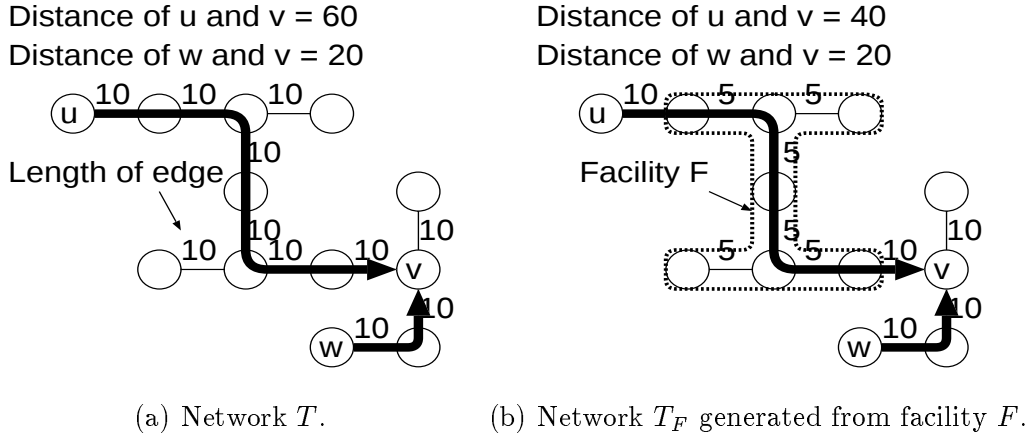
図 5.11: 設備配置と全対コスト
