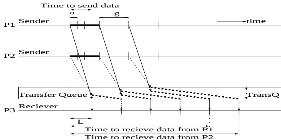
図 2.7: 2 プロセッサ ( P1, P2 ) が同一プロセッサ ( P3 ) にメッセージ送信した場合の通信動作
