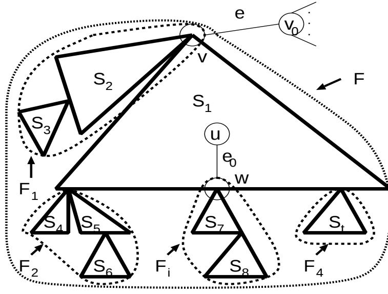
図 4.9: 等分割可能設備の部分設備と残余部分木
