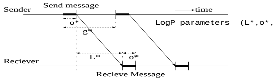
図 2.1: LogP モデルの通信動作
