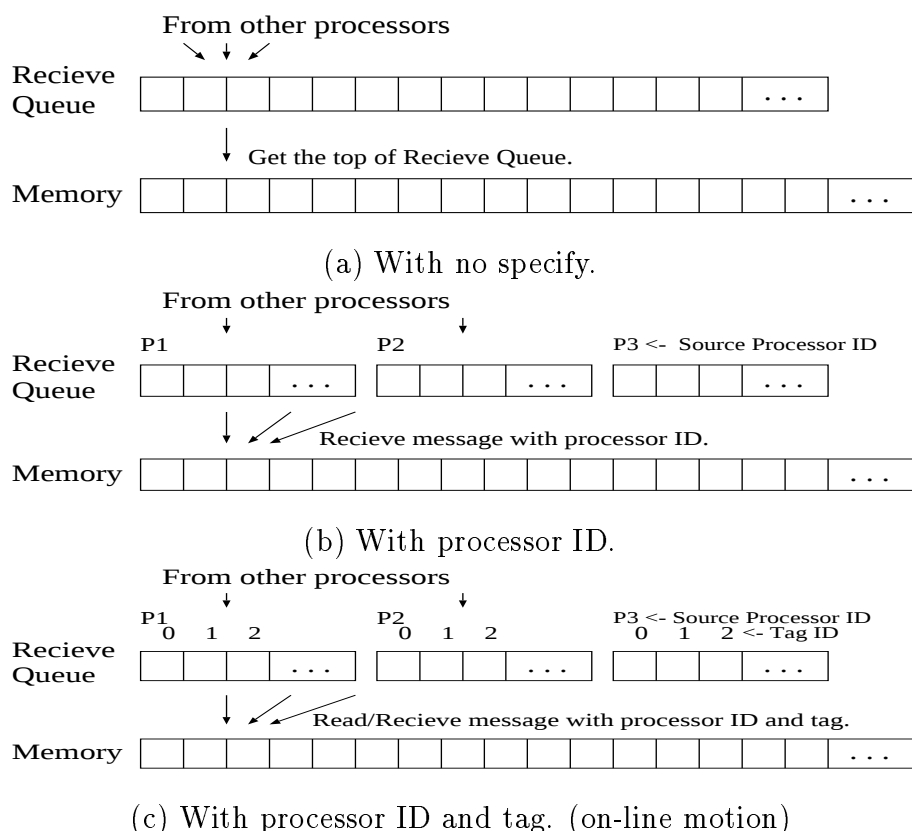
図 2.11: LogPQ モデルの受信部
