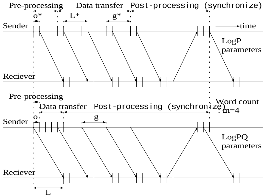
図 2.9: m ワードメッセージのプロトコル通信動作 ( m = 4 )
