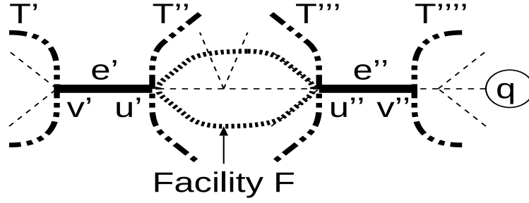
図 5.4: 木 T の設備 F と隣接する長さ \epsilon の部分辺 e' , e'' (重心 q \in V(T''') )
