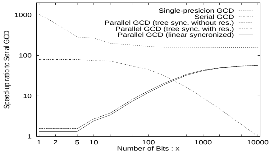
図 3.8: 並列多倍長 GCD アルゴリズムの高速化率 ( L=32, o=4, g=8 ; 線型同期: P=84, s=6 , 木状同期: P=101, s=5 )
