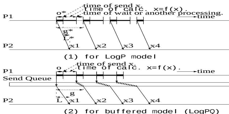
図 2.2: 繰り返し通信の動作
