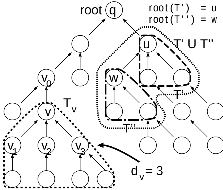
図 4.15: 根が中点 q である有向木 T_q
