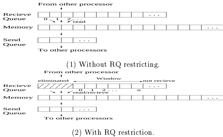
図 2.10: LogPQ モデルの RQ 制限
