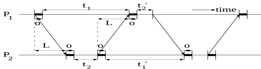
図 2.6: LogPQ モデルの繰り返し通信動作
