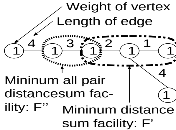
図 5.8: 木 T のサイズ l = 3 の最適な離散木形状設備 F' と距離和最小の離散木形状設備 F''
