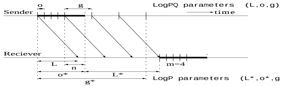
図 2.5: LogP モデルと LogPQ モデルの関係
