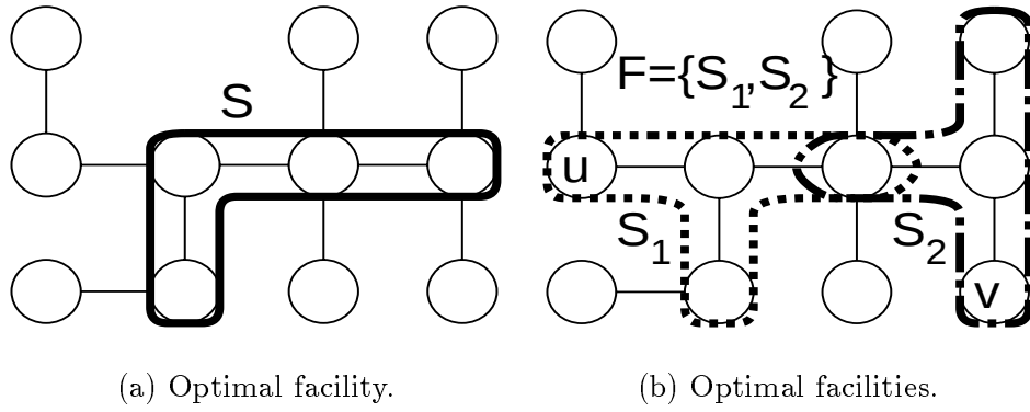
図 4.14: 最適な複数設備
