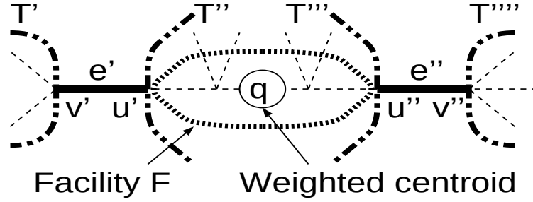
図 5.5: 木 T の設備 F と隣接する長さ \epsilon の部分辺 e' , e'' ( 重心 q \in V(T'' \cap T''') )
