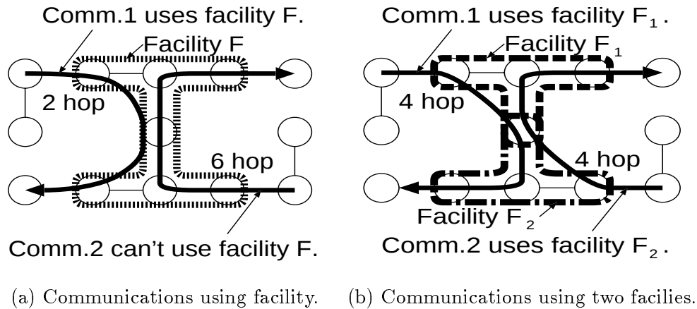
図 4.4: 複数個の設備による通信コスト削減
