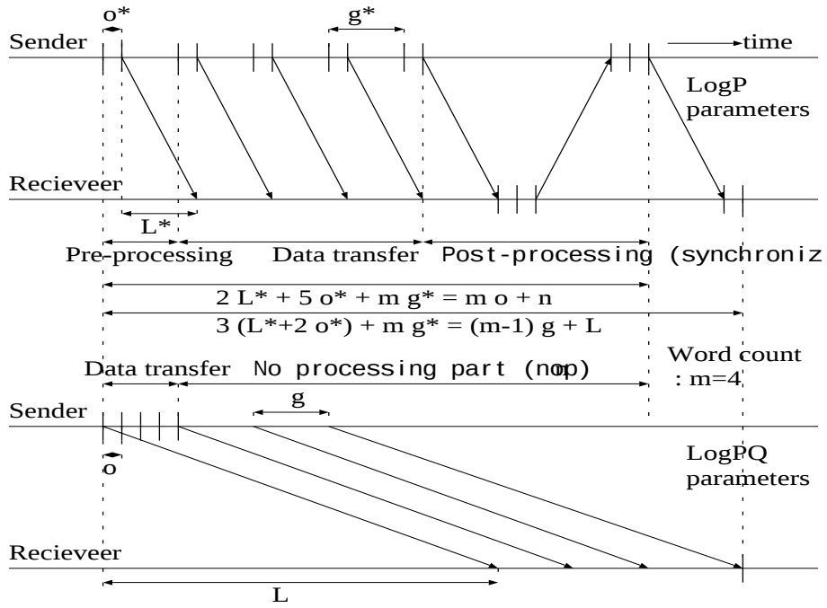
図 2.8: m ワードメッセージの同期通信動作 ( m = 4 )
