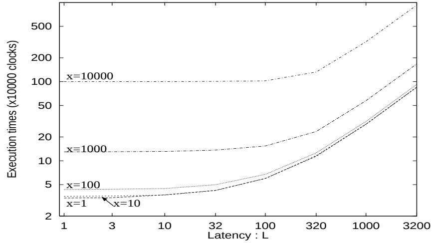
図 3.10: レイテンシ L と並列多倍長 GCD アルゴリズムの実行時間 ( o=4, g=8, s=6 )
