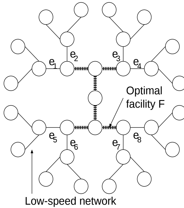
図 4.1: 平衡二分木上の最適な設備 F
