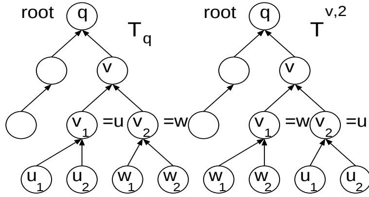
図 4.8: 有向木 T_q と T^{v,2}
