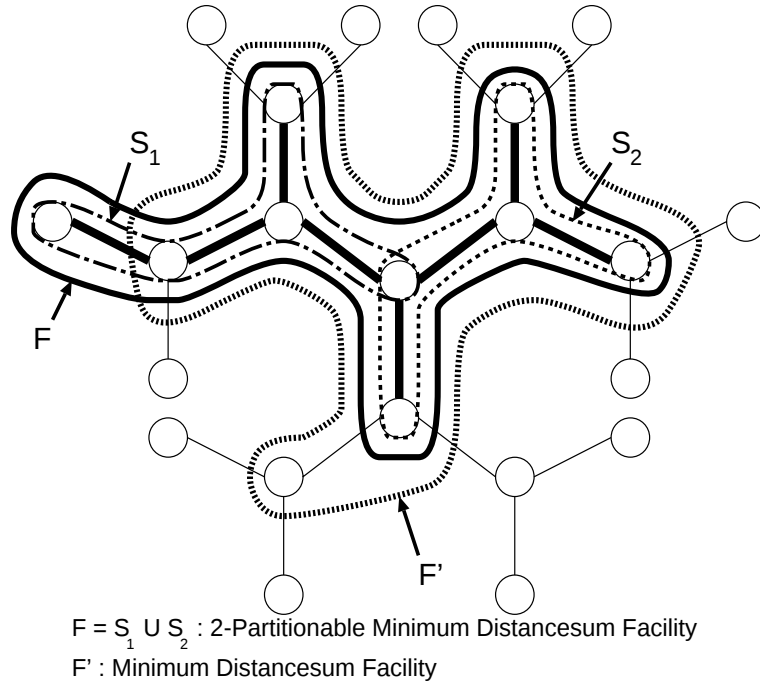
図 4.6: 最適な等分割可能な木形状設備と最適な木形状設備
