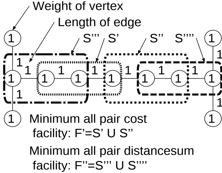
図 5.12: サイズ 2 の木形状の部分設備 2 つからなる，全対コスト最小の設備 F' と全対距離和最小の設備 F''
