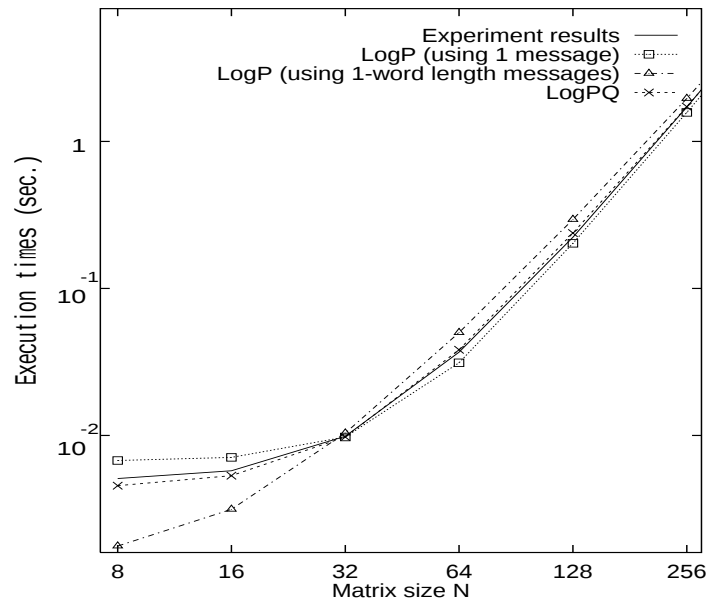
図 3.13: Cannon アルゴリズムの並列計算機 CM5 の 64 プロセッサによる実行時間と LogP および LogPQ モデルによる予測時間の比較
