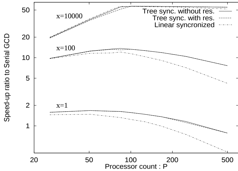
図 3.7: 使用プロセッサ数と並列多倍長 GCD アルゴリズムの高速化率 ( L=32, o=4, g=8 )
