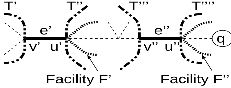
図 5.3: 木 T の設備 F' , F'' と隣接する長さ \epsilon の部分辺 e' , e''
