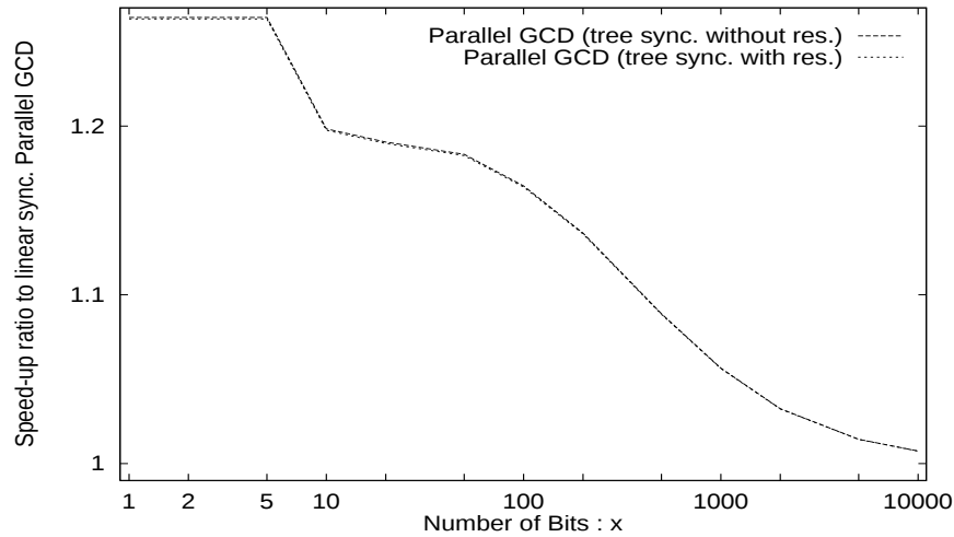
図 3.9: 並列多倍長 GCD アルゴリズムの木状同期の高速化率 ( s=5 )
