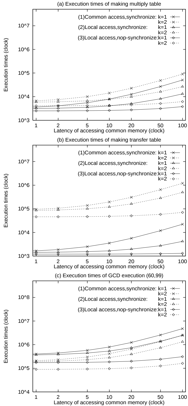
図 3.2: LPRAM モデル上での変形 Chor-Goldreich アルゴリズムの処理時間
