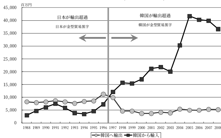
図1 Mold タイプの日韓金型貿易推移(1988～2008)
