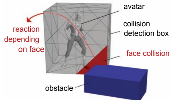
図7 衝突判定モデル
