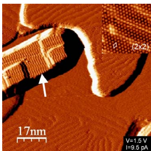
図 3 Si(111)上に成長した \text{ZrB}_2(0001) 薄膜の超高真空走査トンネル顕微鏡像。ほぼ \text{ZrB}_2(0001)-(2 \times 2) 構造 (図中右上に原子分解能像) で覆われているが、成長条件によっては、矢印で示す様な異なる表面構造を示す微結晶が確認された。原子分解能像を詳細に調べた結果、これらは、異なる配向の \text{ZrB}_2 微結晶であることが明らかとなった。
