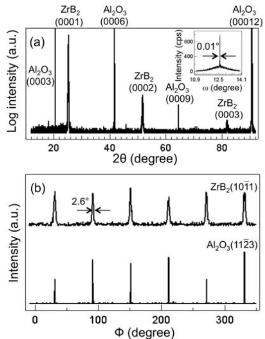
図 2 (a) サファイア上に成長した \text{ZrB}_2 膜の ( \theta - 2\theta ) スキャンと \text{ZrB}_2(0001) 回折のロッピングカーブ。(b) \text{ZrB}_2(10\bar{1}1) と \text{Al}_2\text{O}_3(11\bar{2}3) 回折の \phi スキャン。単一のエピタキシャル関係、 \text{ZrB}_2(0001) // \text{Al}_2\text{O}_3(0001) 及び \text{ZrB}_2[10\bar{1}0] // \text{Al}_2\text{O}_3[11\bar{2}0] が明らかである。
