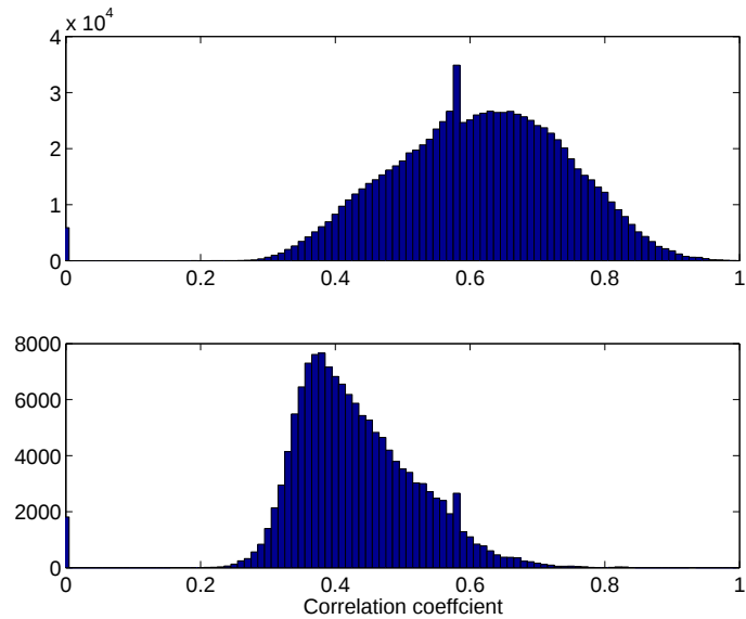
図 3.15: 1 kHz 以下に帯域制限された雑音を付加した音声に対する相関係数の最大値と推定基本周波数誤差の関係: 推定誤差が正解基本周波数の \pm 20\% 未満の点における相関係数のヒストグラム (上)、 \pm 20\% 以上の点における相関係数のヒストグラム (下)
