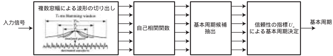
図 A.1: 複数窓幅から得られた自己相関関数を用いる基本周期推定法 (一部、都木 [26] より引用)
