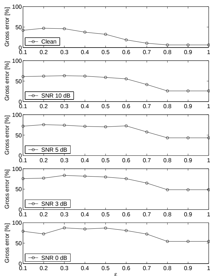
図 4.4: 楕形フィルタの通過帯域幅パラメータ \varepsilon と最終推定結果の関係 (正解基本周波数 F_0(n) \pm 50 Hz が楕形フィルタに入力された場合)
