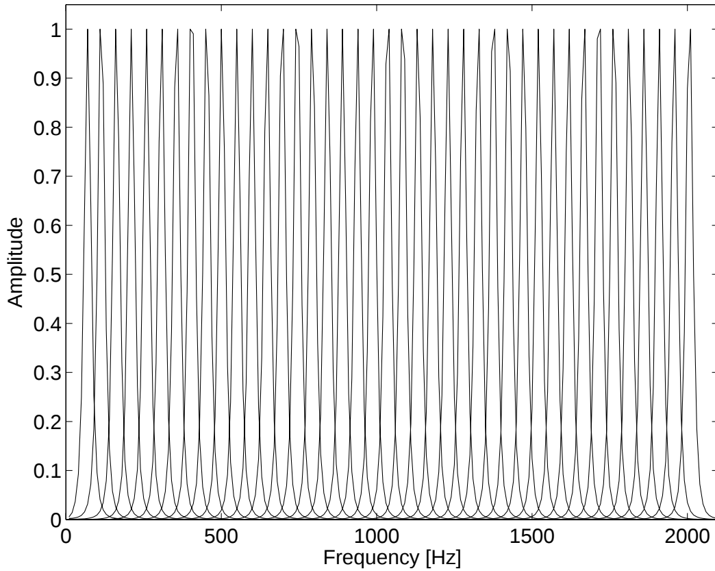
図 3.3: ガンマトーンフィルタによる定帯域フィルタバンクの振幅特性 (チャンネル番号 1, 10, 20, ..., 400 のフィルタを表示)
