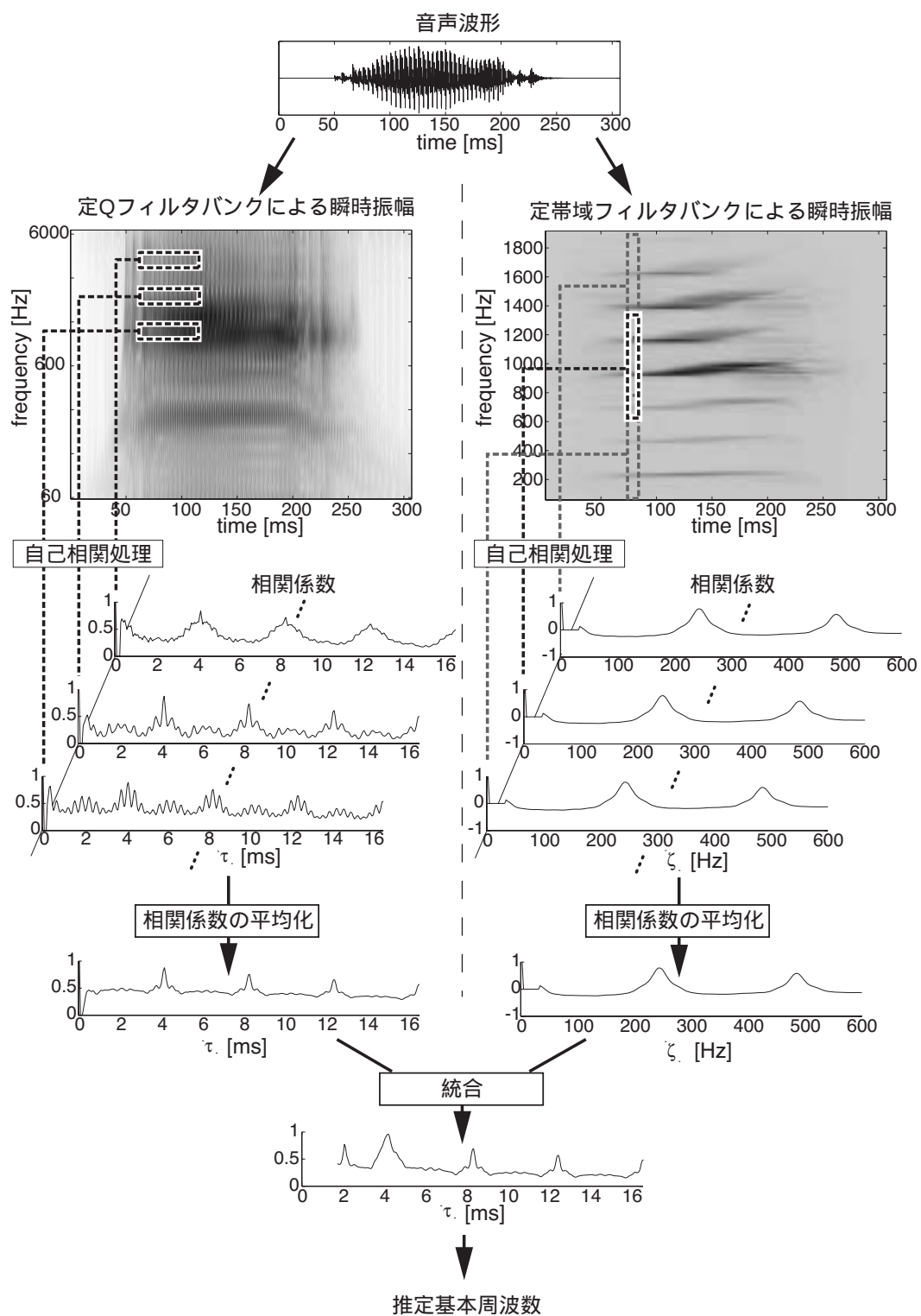
図 3.1: 瞬时振幅の周期性と調波性を基にした基本周波数推定の概要
