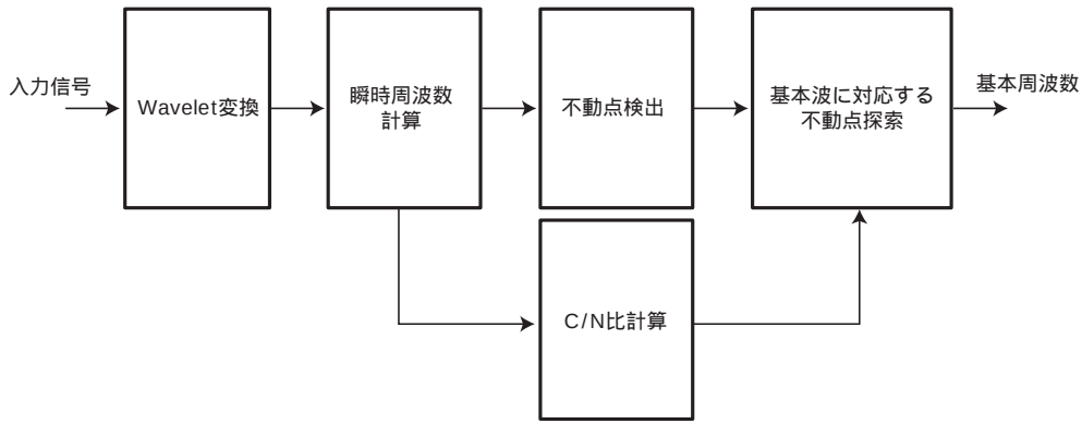
図 B.3: STRAIGHT-TEMPO (Kawahara ら [62])
