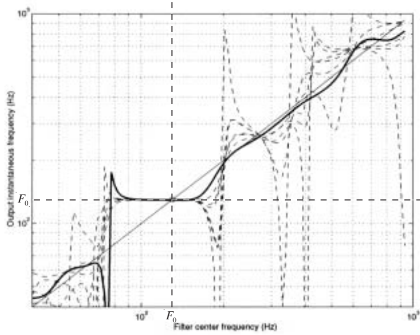
図 B.5: フィルタの中心周波数とフィルタ出力の瞬時周波数の関係 (Kawahara ら [62])
