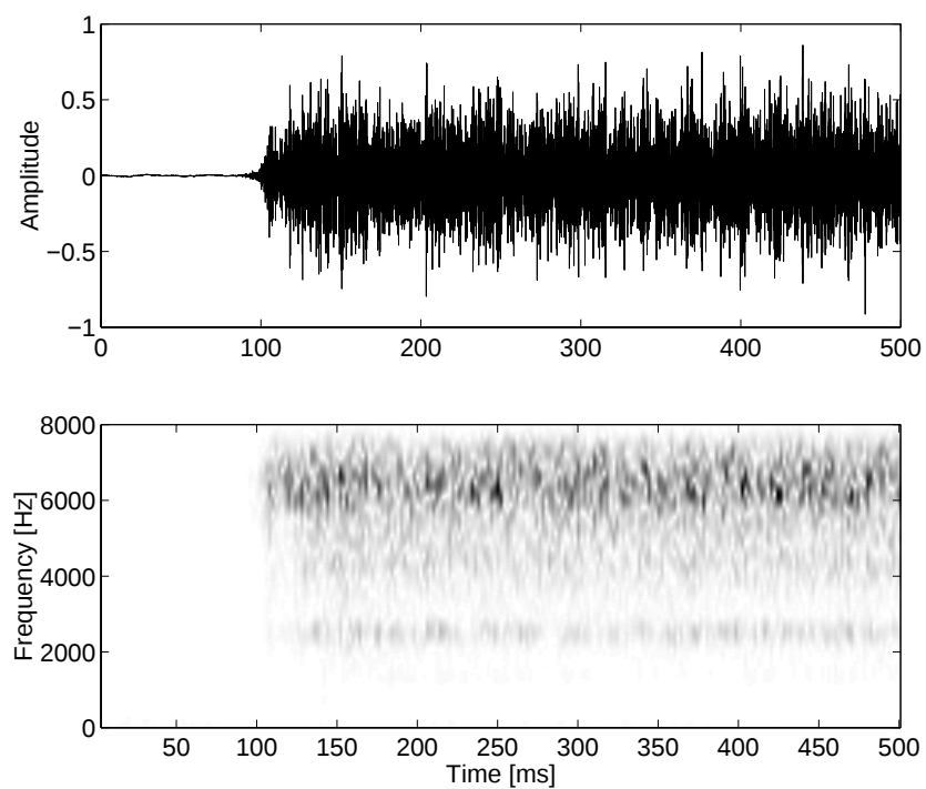
図 1.18: ガススプレーの噴射音 [82] の信号波形とスペクトログラム
