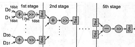
図7 DWT回路
