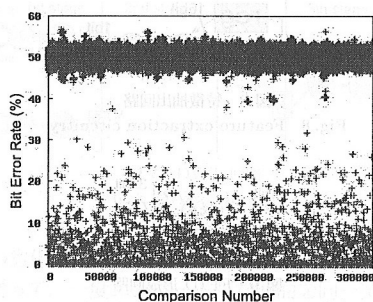
図 10 HiFP(2.97 秒) の BER Fig. 10 BER of HiFP (2.97sec)
