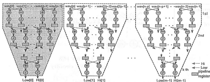
図3 DWTのサブバンド分解のデータフローグラフ
