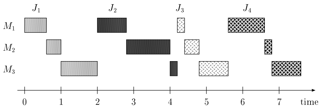
図 2.5: 初期スケジュールの例
