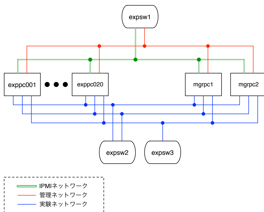
図 6.1: Murubushi の構成
