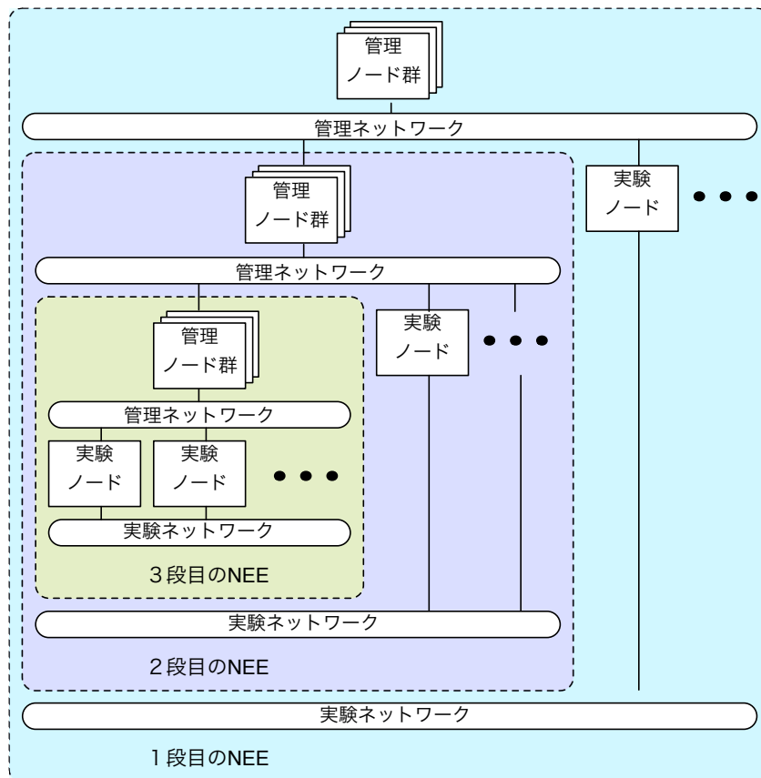
図 4.2: 多段の Nested-NEE
