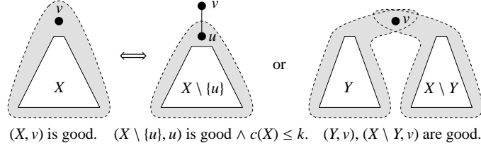
Fig. 3. An illustration of Lemma 4.2.
